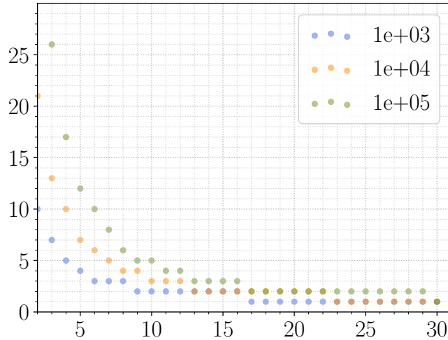
FIGURE 6.12 – Évolution de K_{\text{MISE}} en fonction de la dimension et pour différentes valeurs de la taille de l'échantillon.
