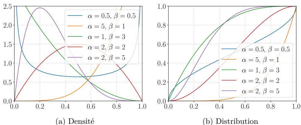
FIGURE 1.8 – Loi bêta pour différentes valeurs des paramètres \alpha et \beta .
