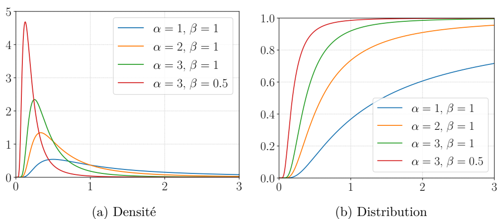
FIGURE 1.9 – Loi inverse-gamma pour différentes valeurs de \alpha et \beta .
