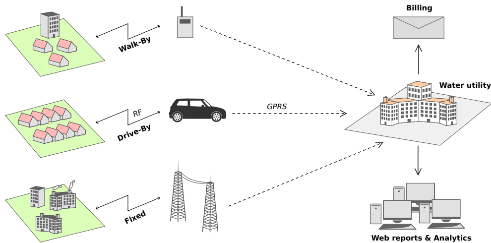
Figure 1.6 – Types de communication des technologies AMR/AMI utilisées dans le comptage de l'eau
