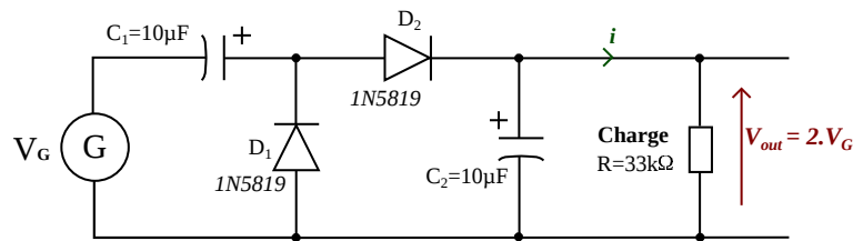
Figure 1.18 – Schéma électrique pour redresser et filtrer la tension alternative récoltée par le générateur électromagnétique proposé
