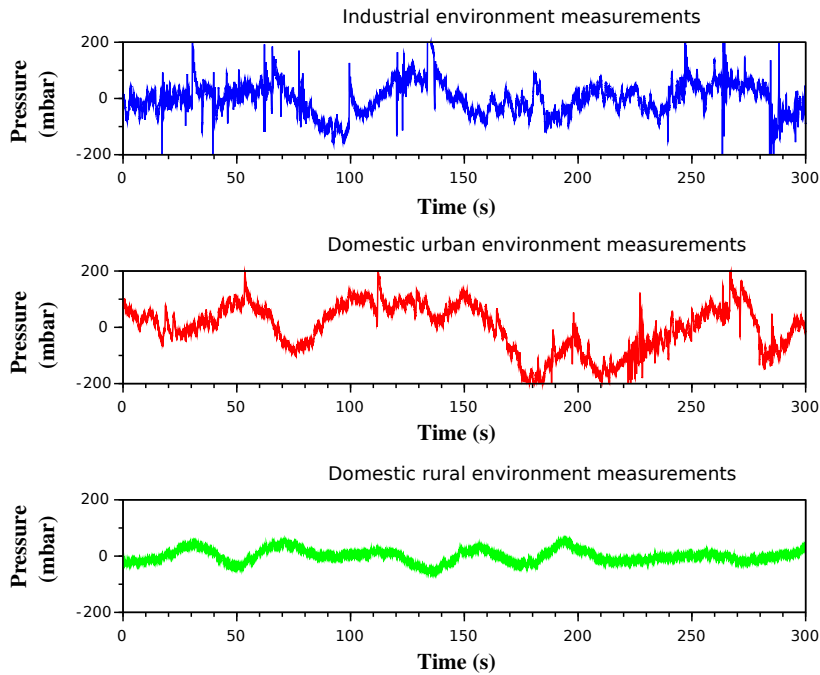
Figure 1.20 – Mesures des variations de pression dans un réseau de distribution industriel, urbain et rural
