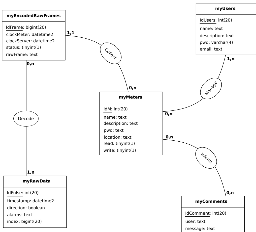
Figure A.5 – Proposition d’un modèle conceptuel de données pour stocker les données collectées dans la plate-forme expérimentale
