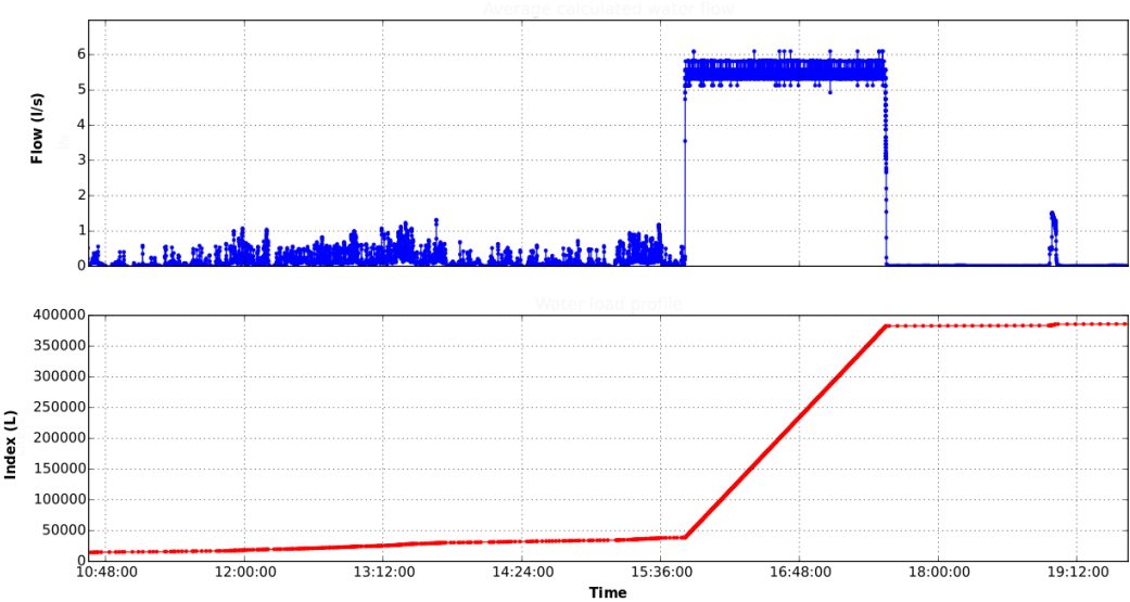
Figure 3.13 – Rupture de canalisation détectée par le système de surveillance le 19 février 2018 sur le compteur principal de l’université
