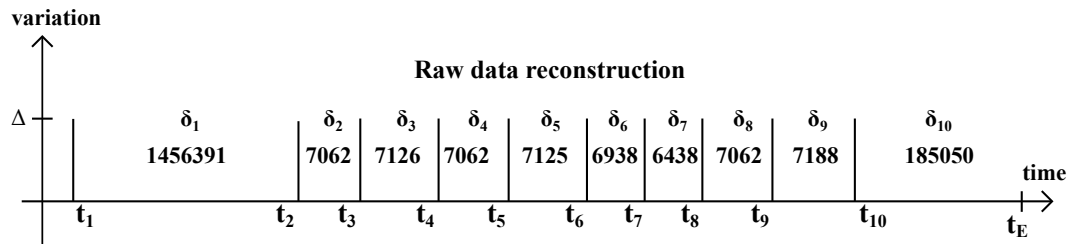
Figure 3.9 – Reconstruction des événements horodatés à partir des données compressées
