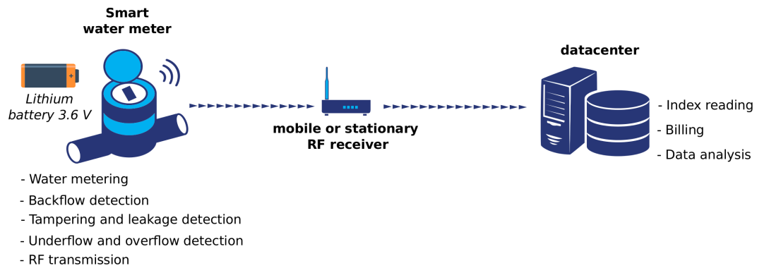
Figure 1.8 – Collecte de données actuelle entre les compteurs d'eau et le centre de données
