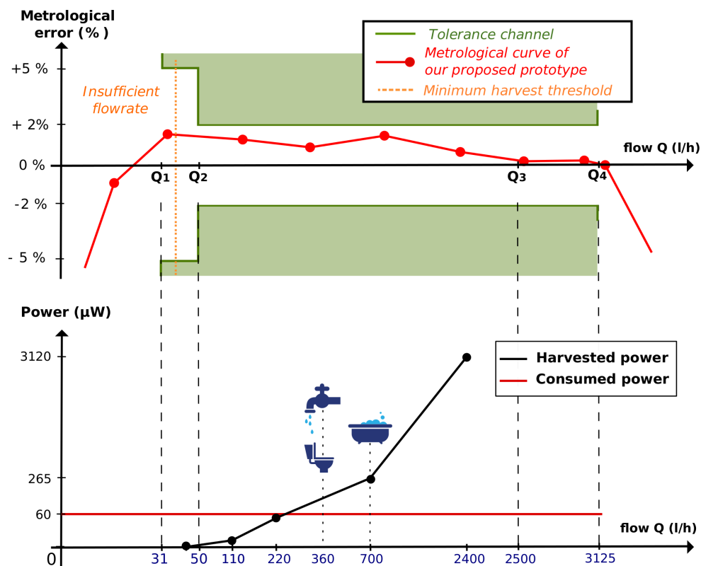
Figure 1.19 – Performances de récupération d'énergie et caractéristiques métrologiques obtenues avec le prototype développé
