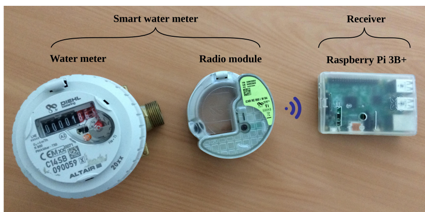
Figure 3.2 – Illustration d'un compteur d'eau mécanique, d'un module radio pour la transmission de données et d'un récepteur pour la réception des messages
