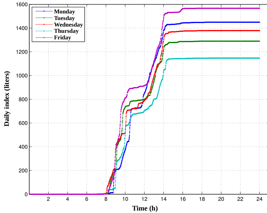
Figure 3.14 – Comparaison des courbes de charge journalières pour une semaine typique de consommation d'eau au restaurant universitaire
