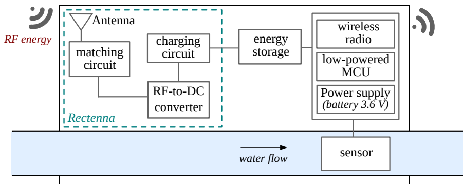
Figure 1.14 – Principe d'un compteur d'eau communicant qui intègre une rectenna pour récupérer l'énergie RF ambiant
