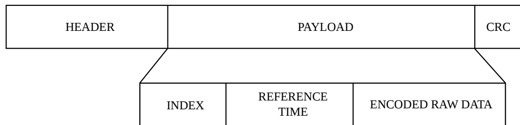
Figure 1.24 – Structure de trame respectant le standard européen EN 13757-4 utilisé dans les tests expérimentaux
