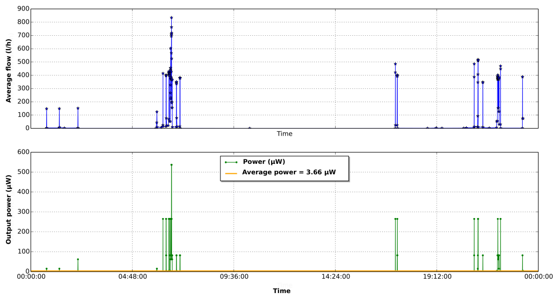
Figure A.4 – Énergie récupérée à partir d'une consommation d'eau journalière dans une maison domestique dans laquelle habite une personne seule
