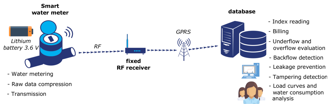
Figure 1.23 – Nouvelle stratégie de collecte de données afin de déporter les traitements et les analyses au niveau du serveur
