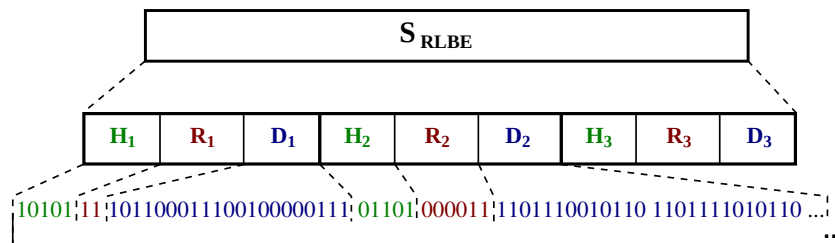
Figure 3.8 – Décomposition de la trame f_E selon la structure RLBE
