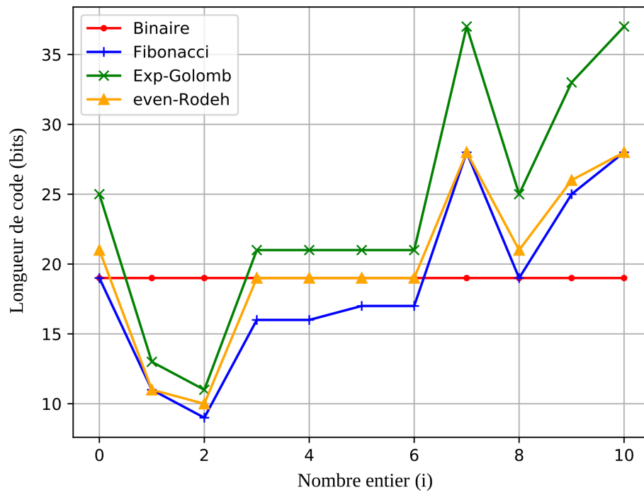
Figure 2.3 – Comparaison du nombre de bits nécessaire pour coder les nombres entiers de la séquence S
