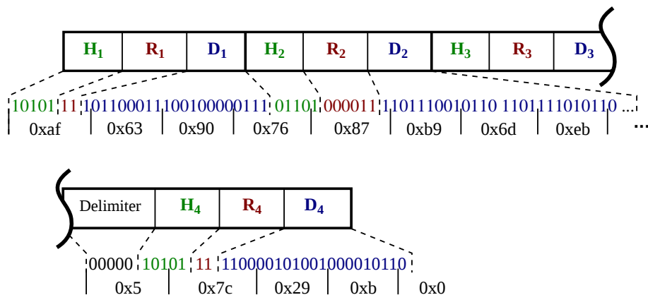
Figure 2.8 – Construction d'un bloc de données selon la structure RLBE définie sur la Fig. 2.7
