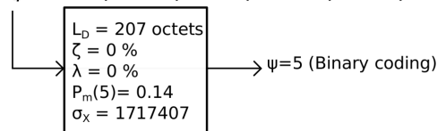
Figure 4.8 – Exemples de valeurs numériques des descripteurs servant à sélectionner l'algorithme de compression pour quatre séquences de données différentes D_1, D_2, D_3 et D_4
