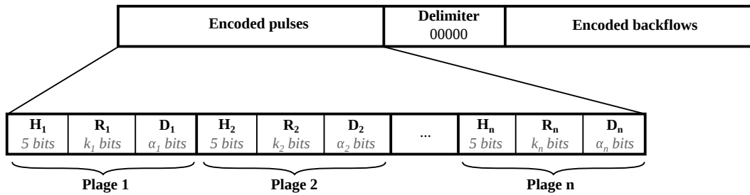
Figure 2.7 – Structure correspondante à l'algorithme RLBE pour l'encapsulation des données compressées
