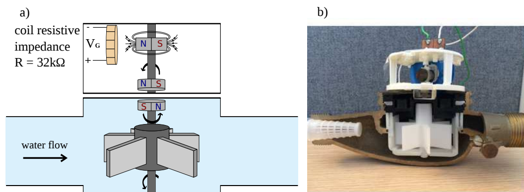
Figure 1.17 – Prototype expérimental qui combine un compteur de vitesse DN15 avec un générateur électromagnétique, a) principe de fonctionnement, b) vue du prototype élaboré
