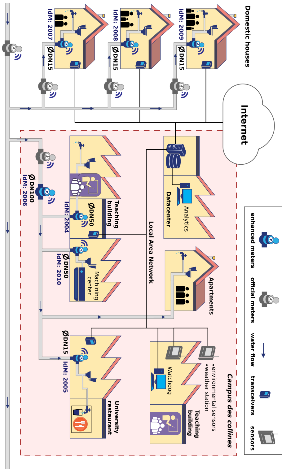
Figure 3.1 – Plate-forme expérimentale conçue pour collecter les données dans des environnements tertiaires, industriels et domestiques
