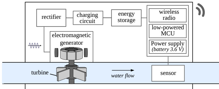
Figure 1.15 – Principe d'un compteur d'eau communicant qui intègre un générateur électromagnétique pour récupérer l'énergie cinétique provenant du flux d'eau
