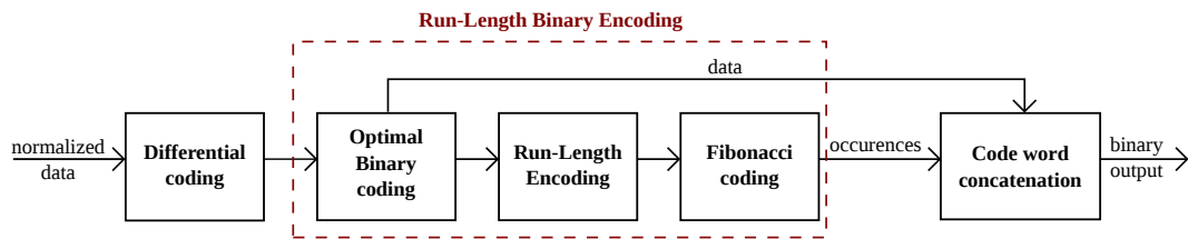
Figure 2.6 – Étapes de codage de l'algorithme de compression RLBE
