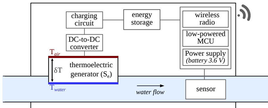
Figure 1.13 – Principe d'un compteur d'eau communicant qui intègre un générateur thermoélectrique pour récolter l'énergie thermique
