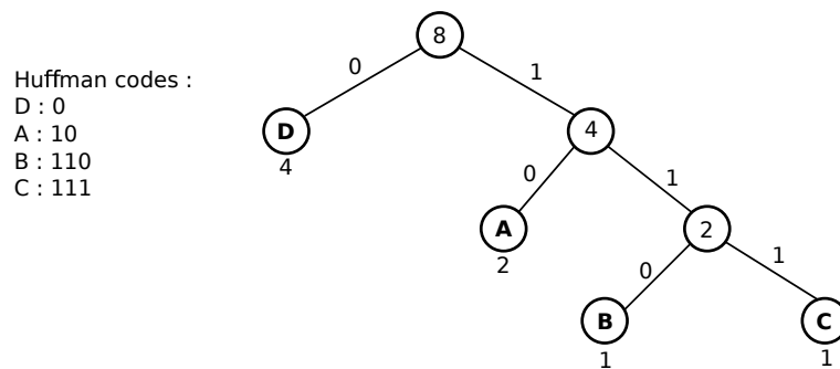
Figure 2.2 – Exemple de construction d’un arbre de Huffman à partir de la séquence S = “AABDCDDD”
