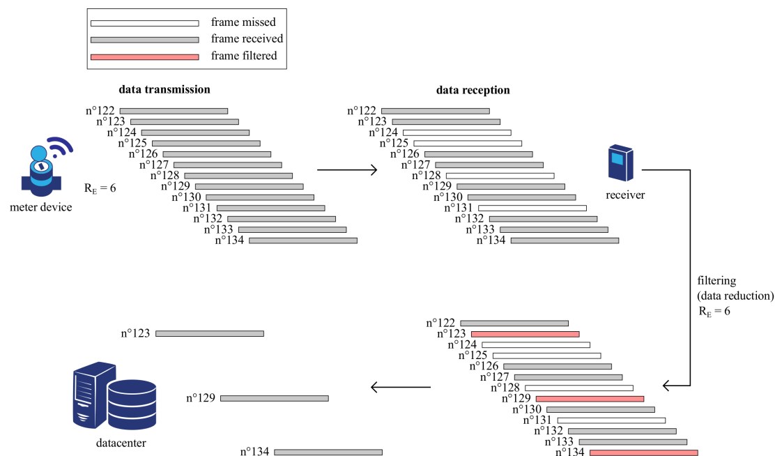
Figure 3.6 – Filtrage mis en place dans le récepteur pour réduire la quantité de données avant les processus de décodage et de stockage
