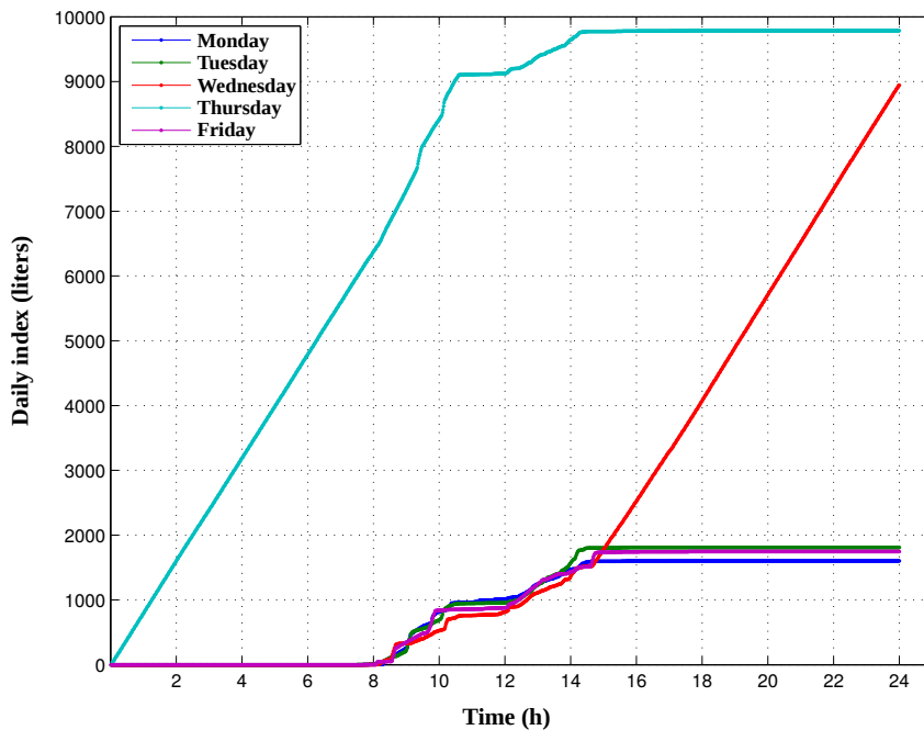
Figure 3.15 – Détection de fuite au restaurant de l'université à partir des courbes de charge échantillonnées entre Mercredi 14h30 et Jeudi 9h00
