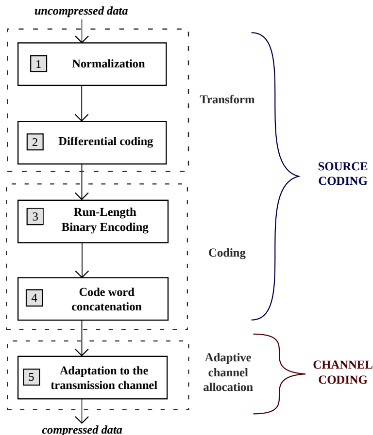
Figure 2.4 – Nouvelle méthode de compression sans perte basée sur cinq étapes de codage différentes
