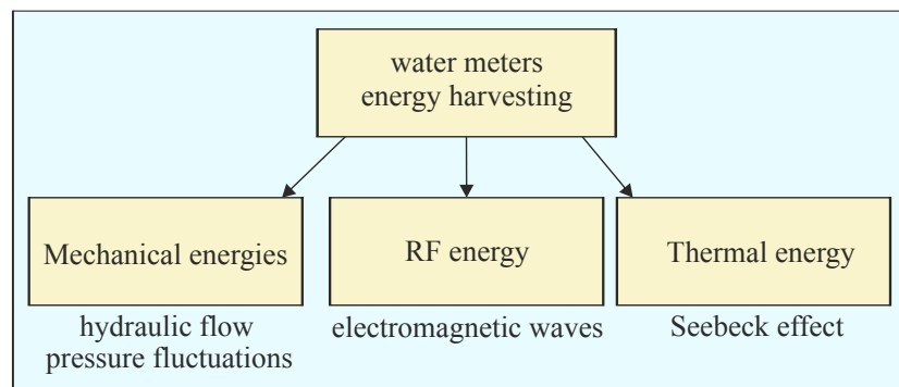
Figure 1.12 – Principes physiques de récolte d'énergie au sein des compteurs d'eau
