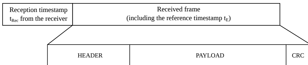
Figure 3.7 – Trame envoyée par le récepteur avec l'horodatage de réception pour synchroniser les dérives d'horloge
