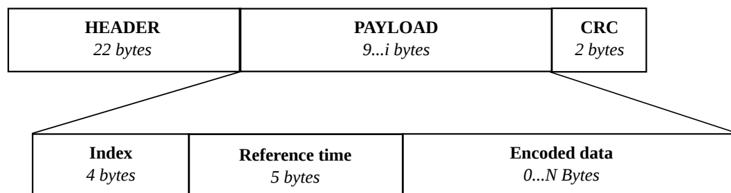
Figure 3.5 – Décomposition des trames réceptionnées pour le décodage de source
