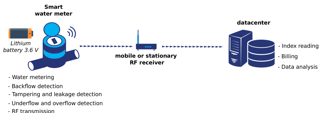
Figure 1 – Chaîne de communication générale entre un compteur d'eau intelligent et un serveur hébergeant une base de données
