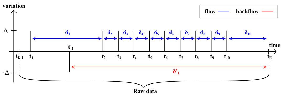
Figure 2.5 – Normalisation et transformation des données brutes entre les instants t_{E-1} et t_E
