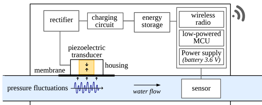
Figure 1.16 – Principe d'un compteur d'eau communicant qui intègre un transducteur piézoélectrique pour récupérer l'énergie hydraulique provenant des variations de pression
