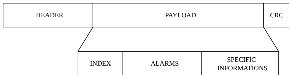
Figure 1.9 – Structure de trame générale respectant le standard européen EN-13757-4
