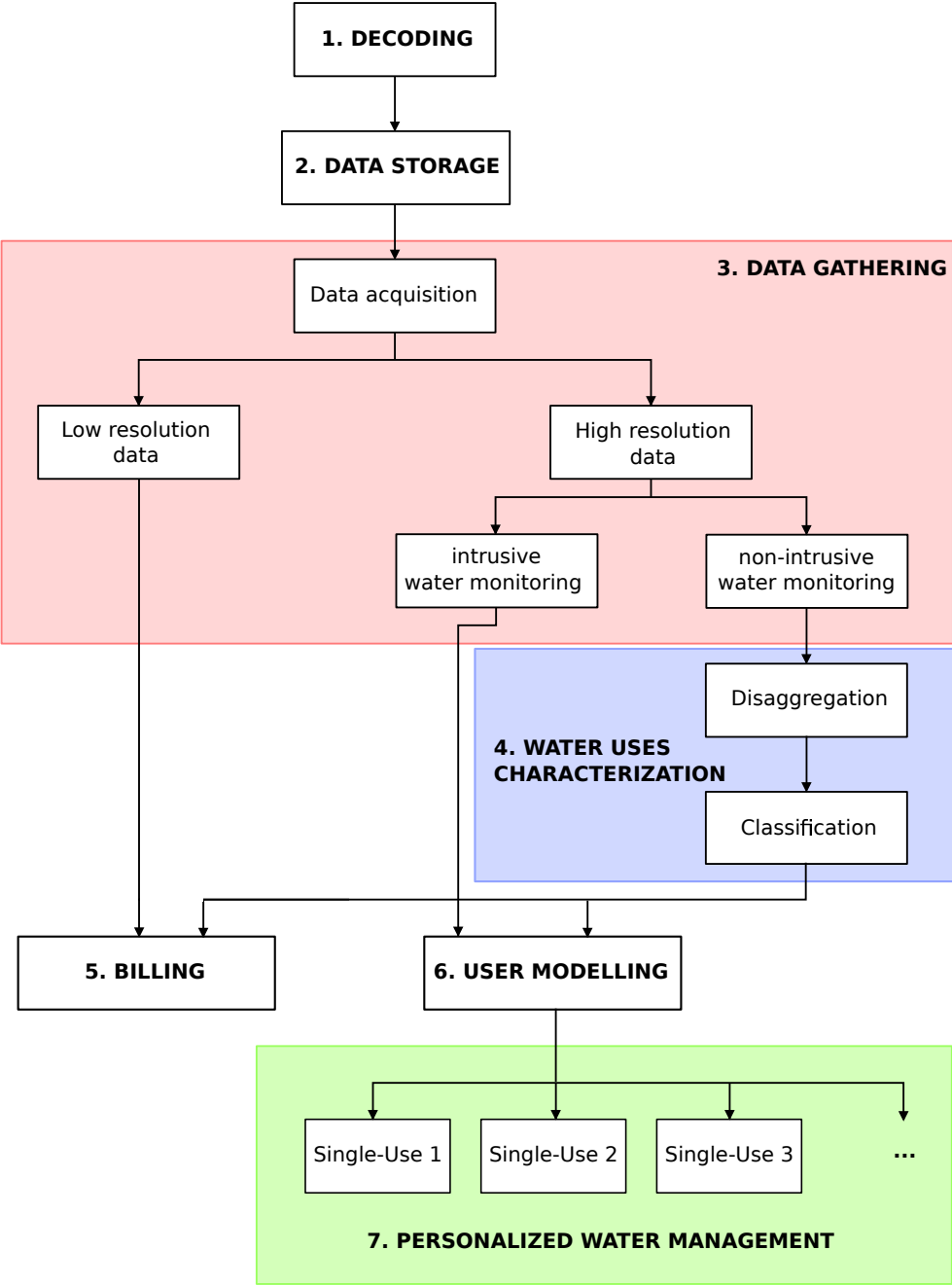
Figure 3.3 – Diagramme illustrant les différentes étapes de la réception des messages jusqu’à la gestion personnalisée de l’eau
