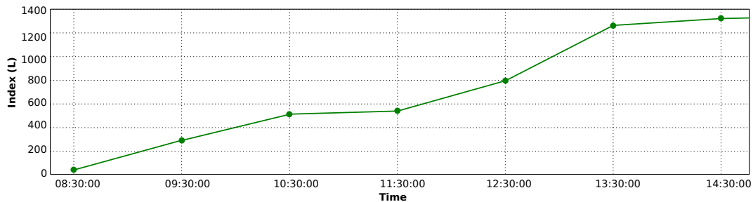
Figure 1.10 – Exemple d'une courbe de charge établie à partir des index collectés toutes les heures
