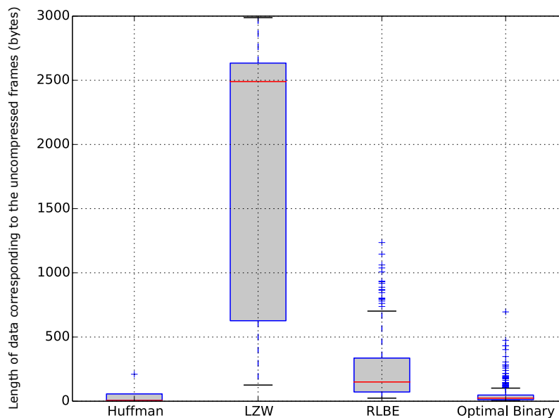
Figure 2.15 – Dispersion statistique sur les performances des algorithmes de compression en fonction de la longueur des données originales
