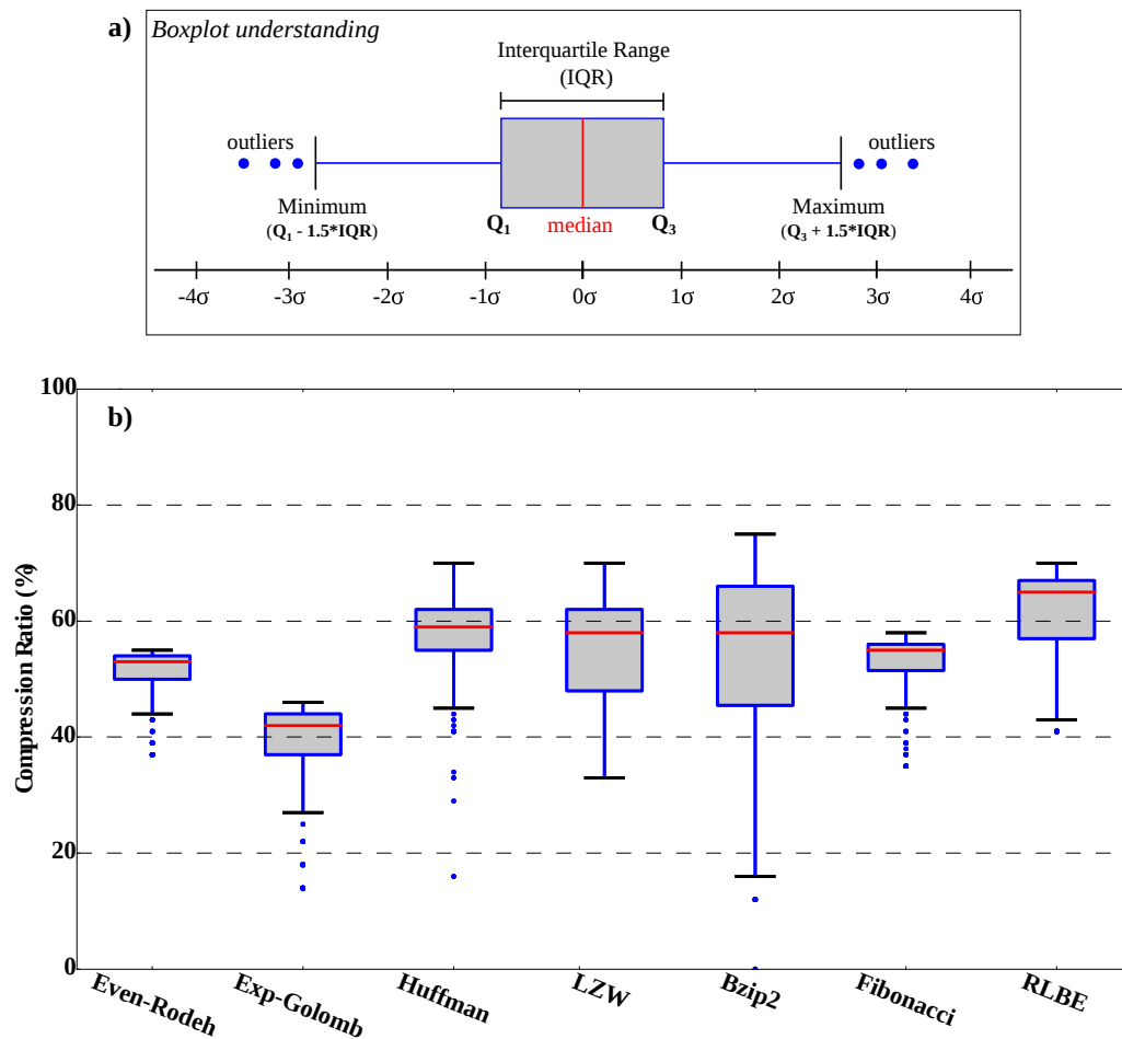
Figure 2.10 – Comparaison de la mesure de dispersion des taux de compression obtenus entre le codage RLBE et six autres algorithmes, a) principe général d'un diagramme en boîte, b) diagrammes en boîte des sept algorithmes de compression
