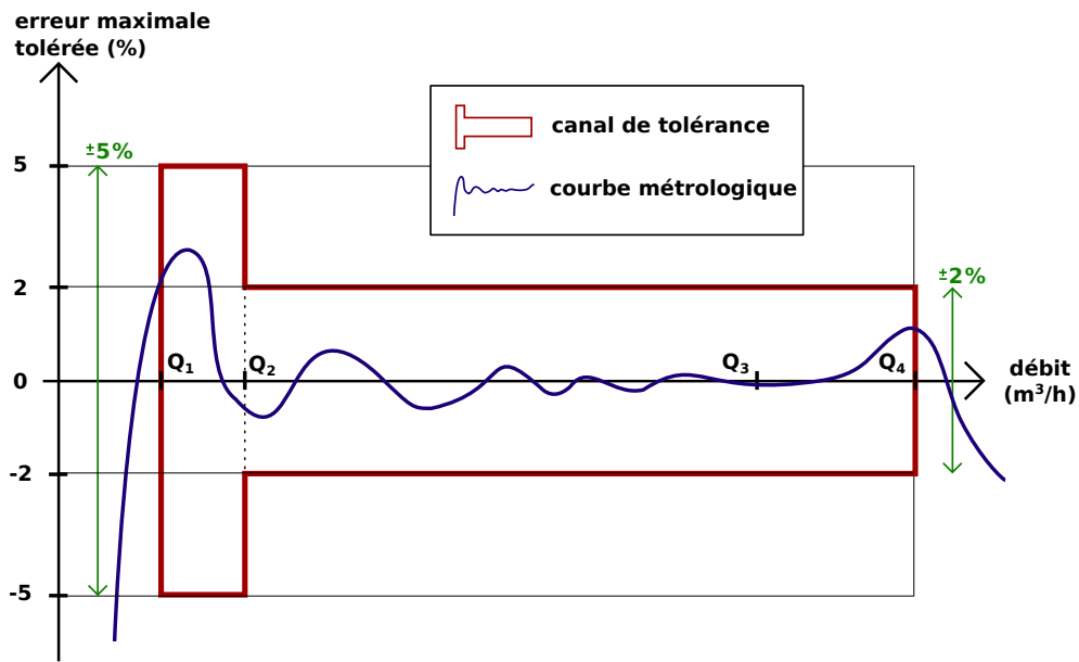
Figure 1.4 – Erreur maximale tolérée en fonction du débit dans le comptage de l'eau selon la norme EN 14151-1
