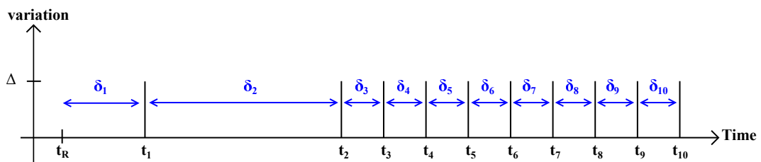
Figure 4.1 – Caractérisation de l'horodatage de référence t_R et codage différentiel des événements horodatés
