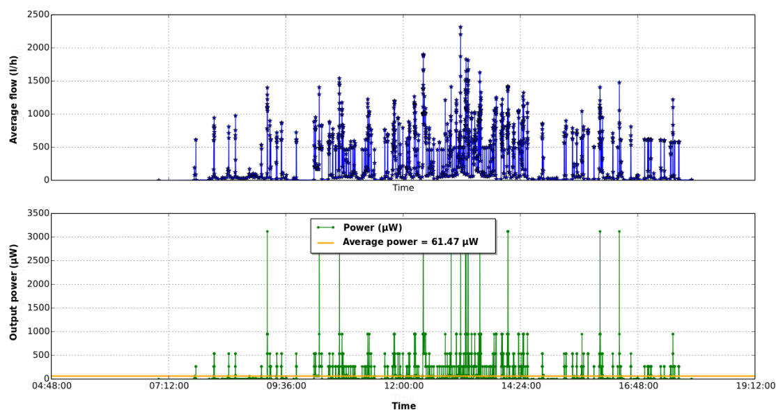
Figure A.2 – Énergie récupérée à partir d'une consommation d'eau journalière dans un bâtiment tertiaire qui accueille environ 80 personnes
