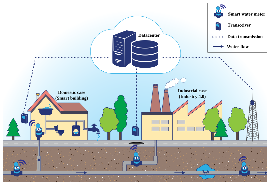
Figure 2 – Contexte général des compteurs d'eau communicants pour améliorer l'analyse de la consommation et la gestion du réseau de distribution
