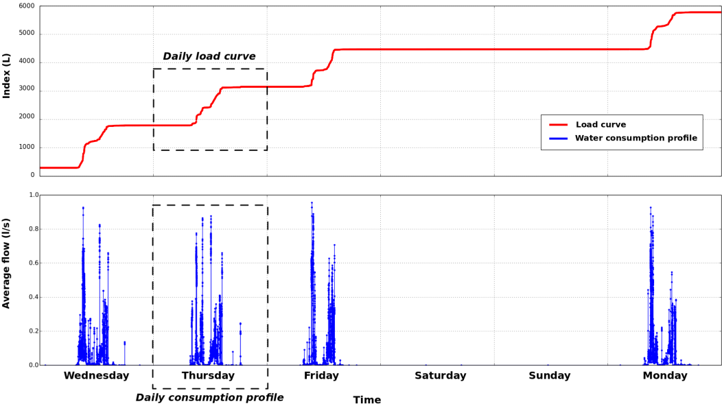
Figure 3.12 – Courbe de charge et profil de consommation illustrant la consommation sur six jours successifs au sein du restaurant universitaire à l’IUT de Mulhouse
