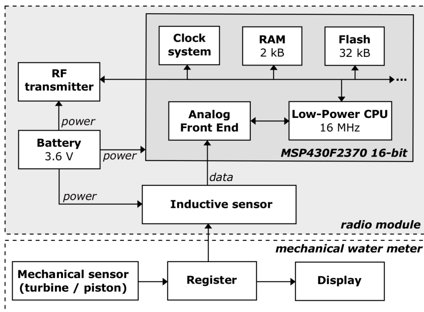
Figure 1.5 – Schéma bloc d'un module radio IZAR RCi de Diehl Metering et utilisé pour les tests expérimentaux
