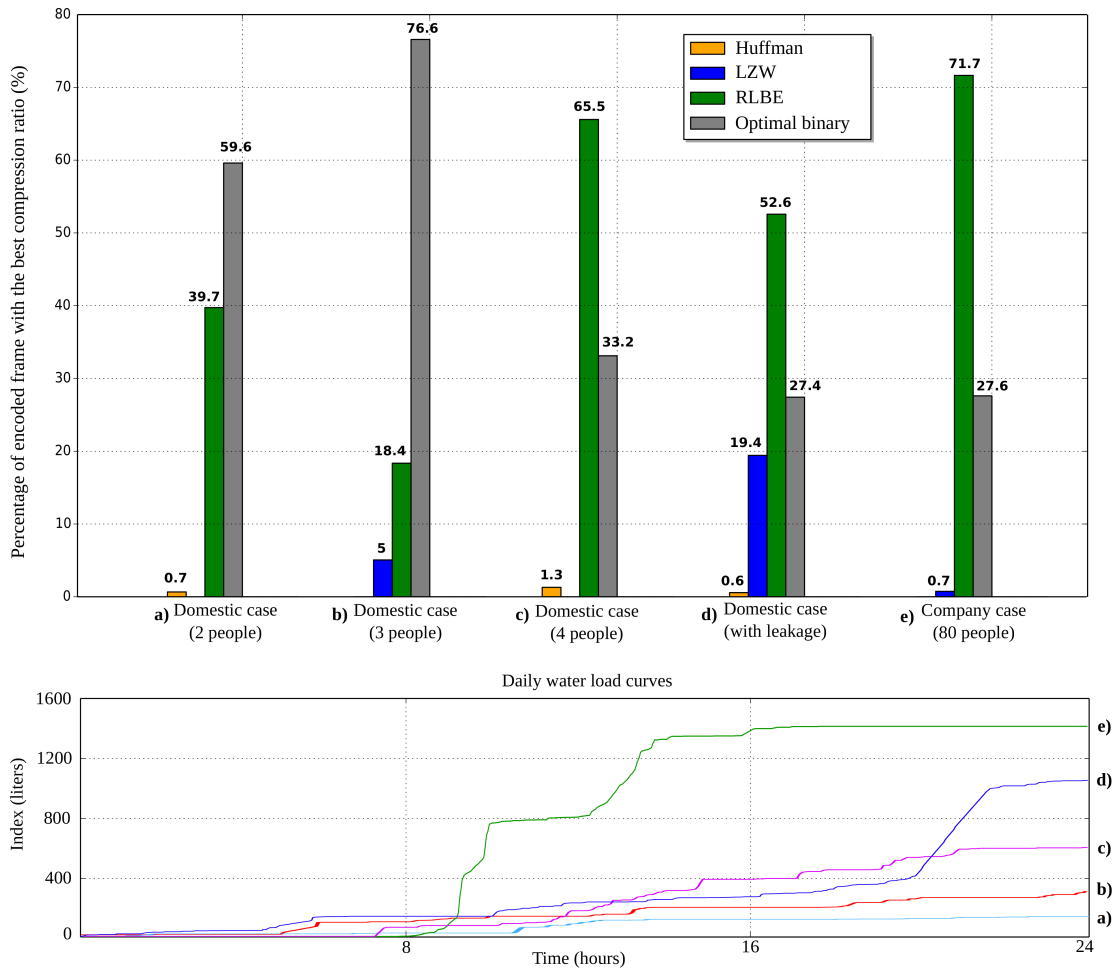
Figure 2.14 – Taux d’utilisation des algorithmes de compression testés pour l’encodage des données de consommation dans cinq environnements différents, illustrés par les courbes de charge a), b), c), d) et e)
