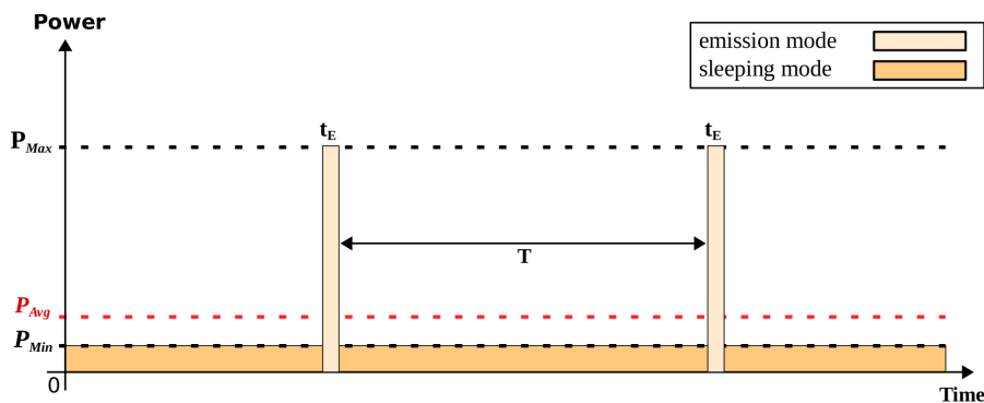
Figure 1.7 – Illustration de la consommation d'énergie lors du mode veille et du mode de communication pour les compteurs d'eau intelligents
