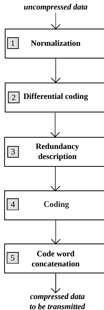
Figure 4.6 – Organigramme de la méthode proposée pour la compression de données dynamique sans perte
