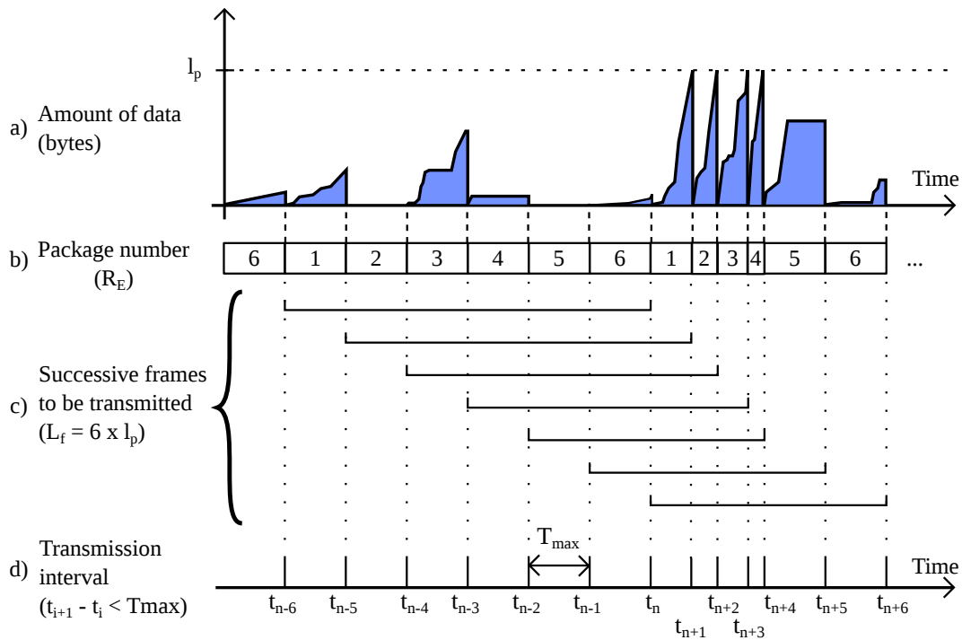
Figure 2.9 – Fiabilisation de la transmission des données à l’aide d’une fenêtre glissante basée sur les paramètres T_{max} , R_E=6 et L_f
