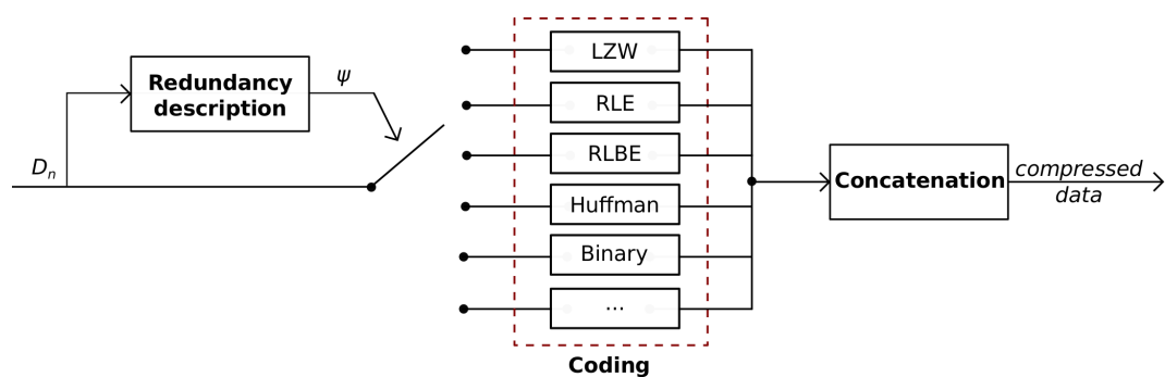
Figure 4.7 – Schéma bloc illustrant la sélection de l'algorithme de compression en fonction des redondances décrites dans les données d'origine
