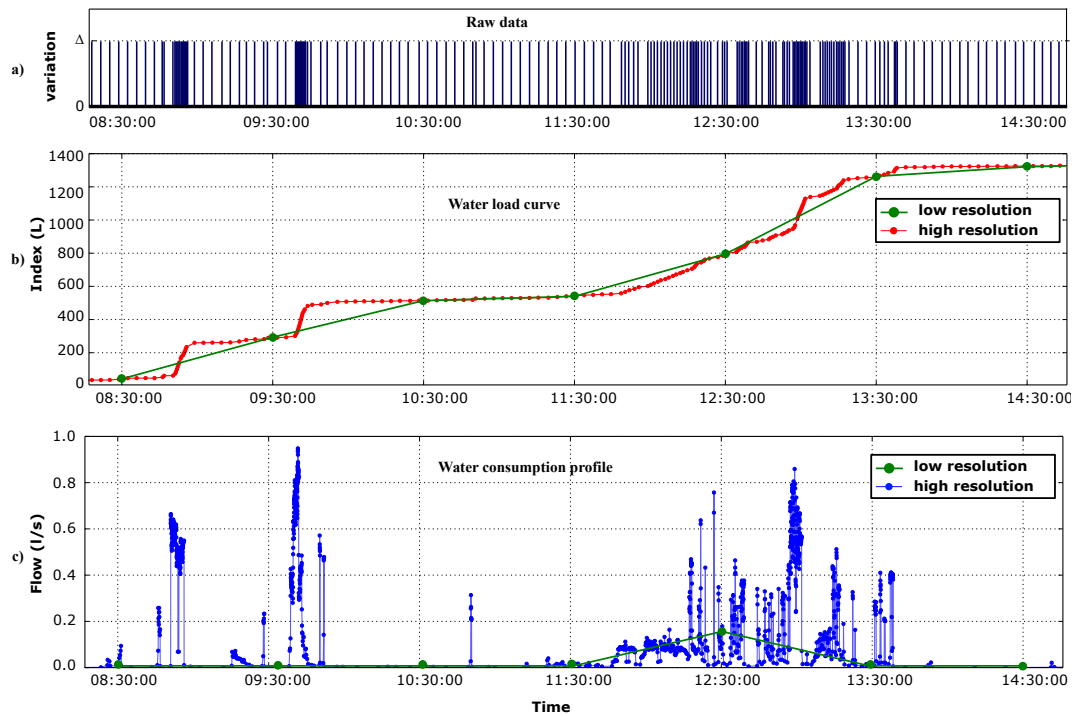
Figure 1.22 – Représentation des données brutes, des courbes de charge et des profils de consommation associés, a) données brutes mesurées, b) comparaison entre la courbe de charge à partir des index relevés toutes les heures et celle à partir des données brutes (événements horodatés), c) profils de consommation calculés à partir des données brutes
