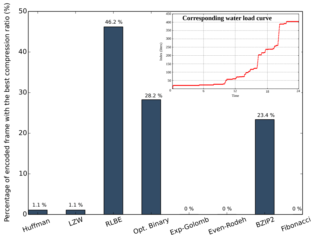
Figure 2.13 – Taux d'utilisation des algorithmes pour la compression des données d'une consommation domestique de trois personnes (taux moyen sur 24h)
