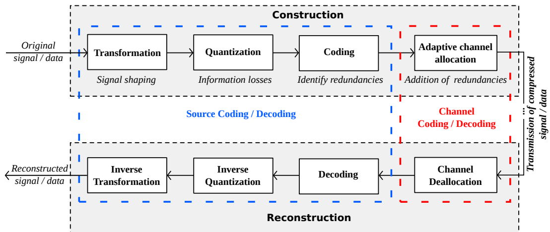
Figure 2.1 – Architecture générale pour la compression et la décompression de données
