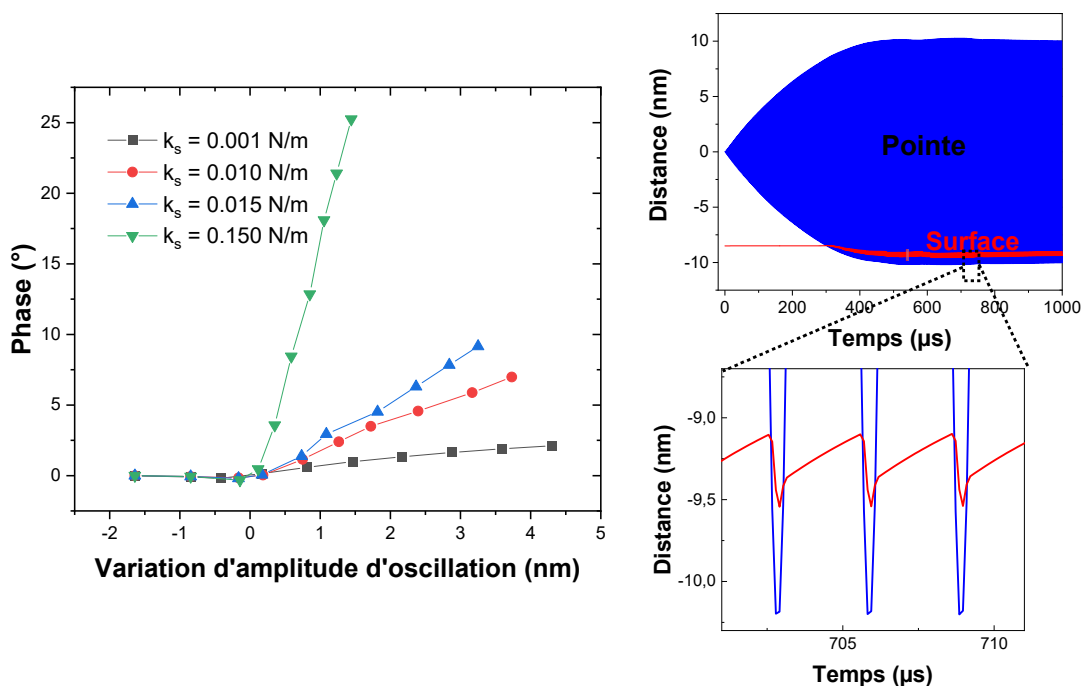
FIGURE 3.11 – Simulation du décalage de phase pour des valeurs croissantes de rigidités de la surface. La variation de phase pour k_s = 0,15N/m montre une variation très proche de nos valeurs expérimentales montrées dans la Fig 3.7. Les inserts montrent les déformations instantanées du levier et de la surface
