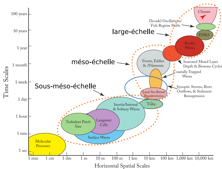
FIGURE 1.9. – Échelles temporelles et spatiales des processus océanographiques. Les processus constituant la circulation océanique peuvent être caractérisés par trois grandes catégories spatio-temporelles : la sous-méso-échelle (dizaines de m – dizaine de km, horaire à journalier), la méso-échelle (dizaines de km – centaines de km, dizaines de jours – quelques mois) et la large-échelle (dizaines de km – centaines de km, dizaines de jours – quelques mois). D’après Dickey et Bidigare, 2005 ; Nichols et Raghukumar, 2020.
