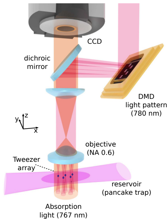
Fig. 0.2: Schéma de l'installation de notre laboratoire à Strasbourg utilisée pour produire et charger les réseaux de pincettes en projetant la lumière d'un dispositif numérique à micromiroirs directement sur les atomes confinés dans un piège à réservoir optique (reproduite de [51]).
