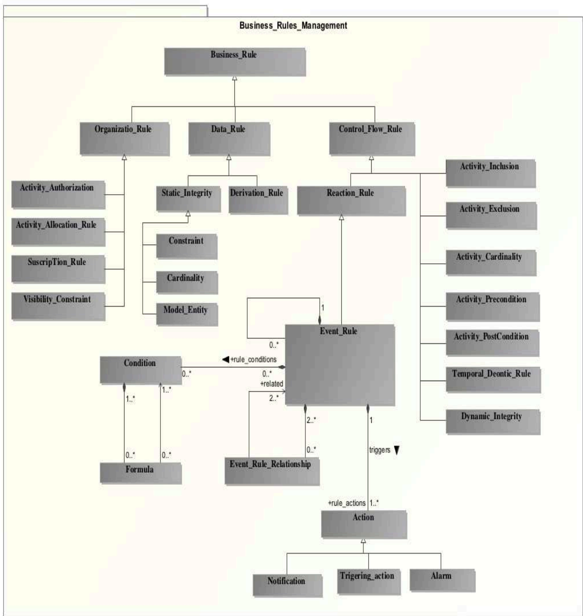
Figure 12. Méta-modèle des contraintes et des règles métier
