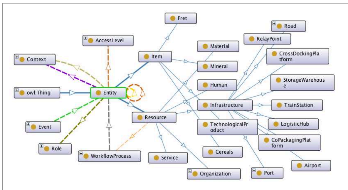
Figure 59. Arbre de classification de la classe Entity
