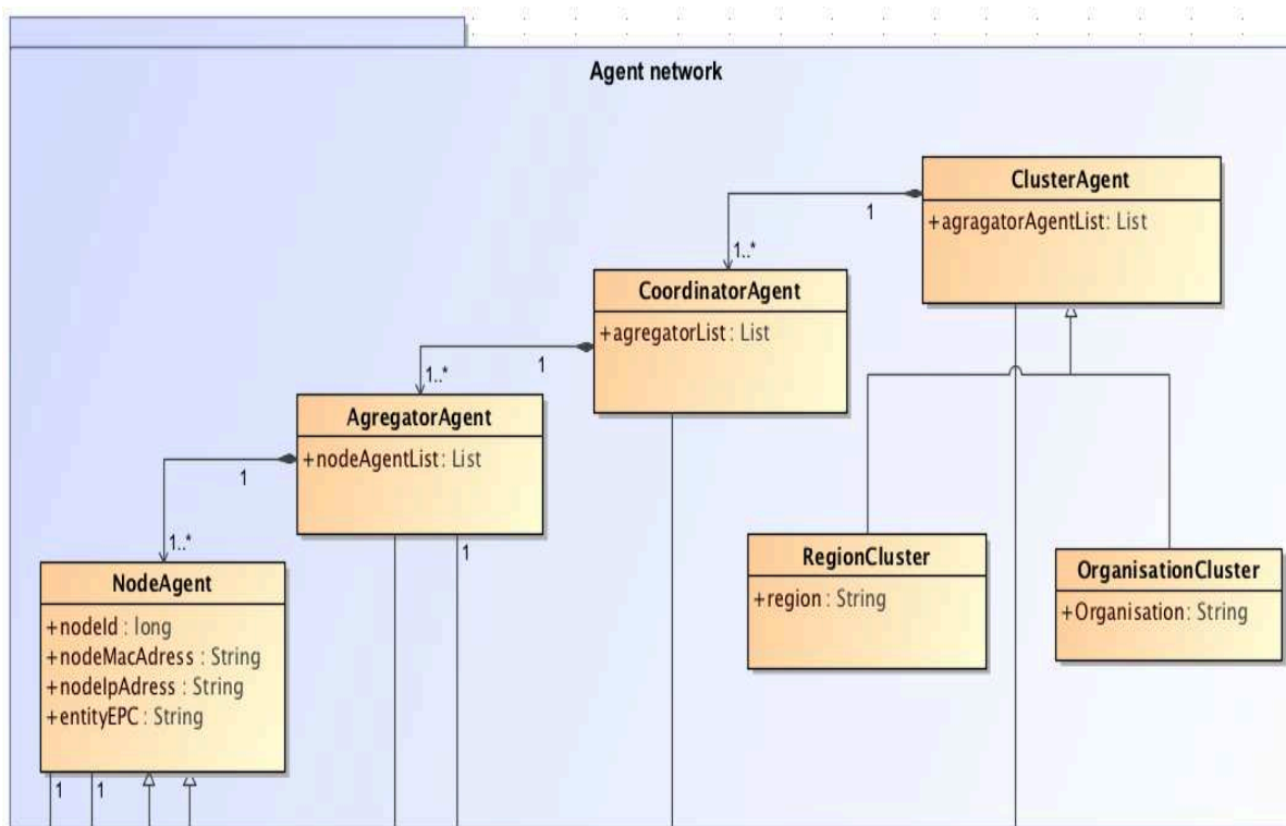
Figure 54. Diagramme UML du réseau d'agents
