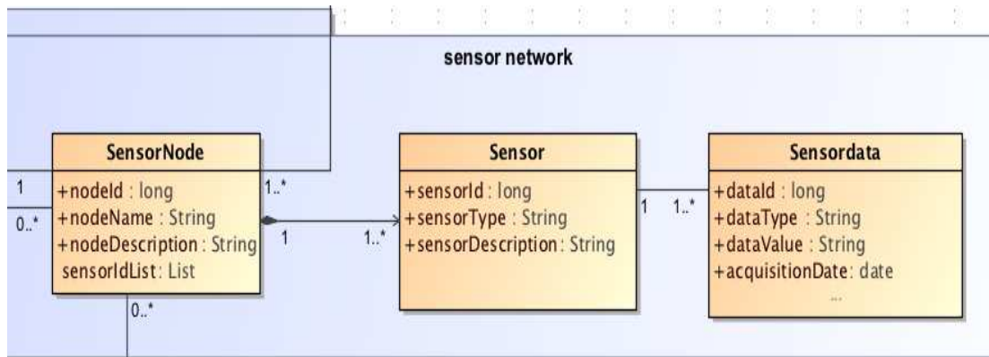
Figure 51. Schéma UML du réseau de capteurs
