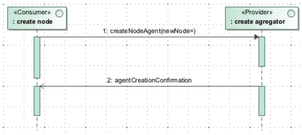
Figure 58. Diagramme d'interaction lors de la création d'un NodeAgent
