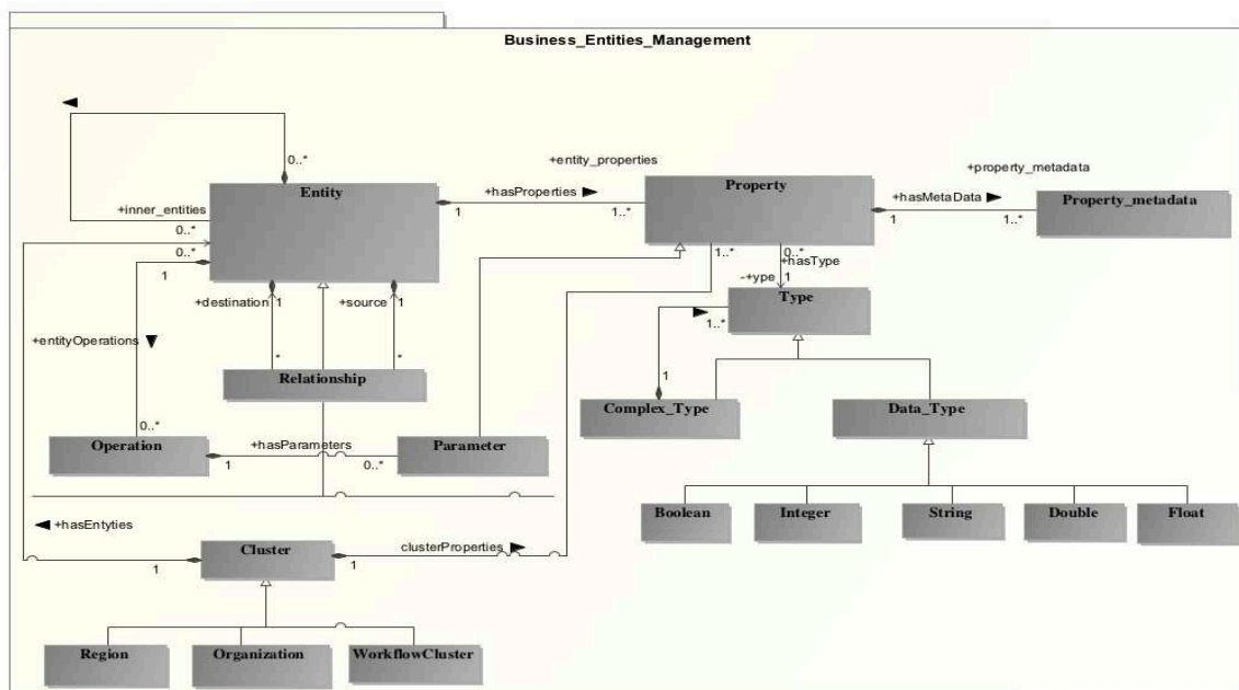
Figure 7. Méta-modèle des entités logistiques et leurs dépendances
