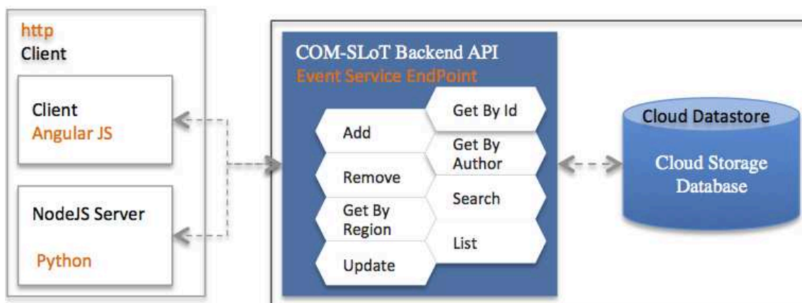
Figure 84. Composant du service de gestion et publication d'événements
