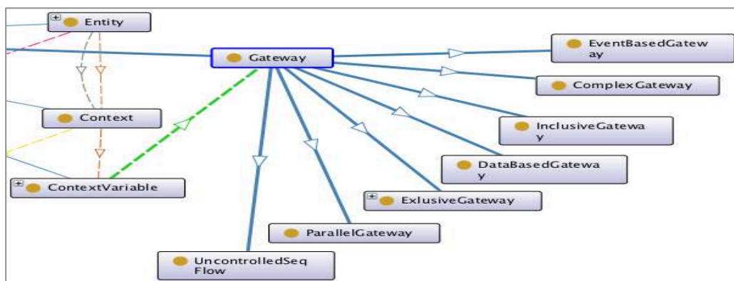
Figure 65. Ontologie du Gateway
