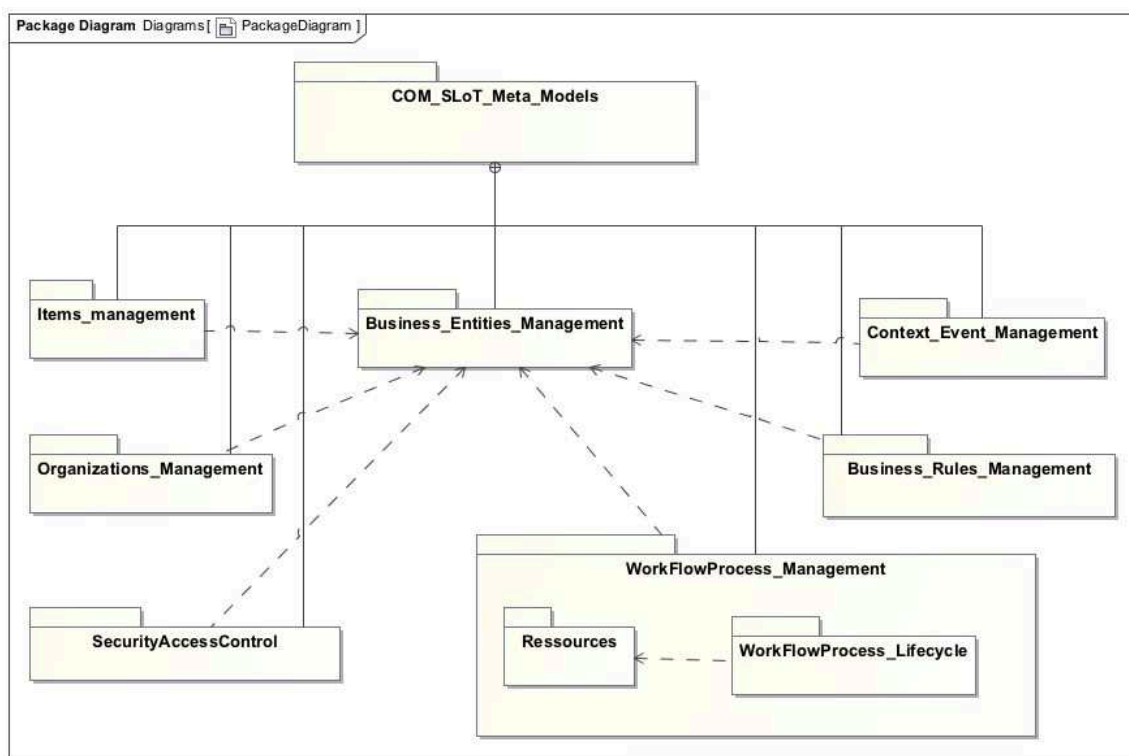
Figure 6. Diagramme de Packages et leurs interdépendances
