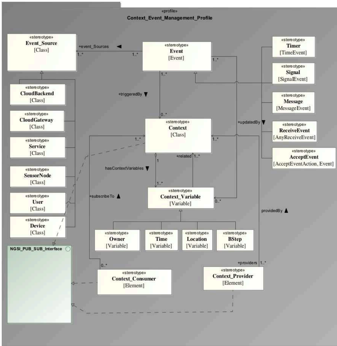
Figure 18. Profil UML pour le contexte de l'objet logistique
