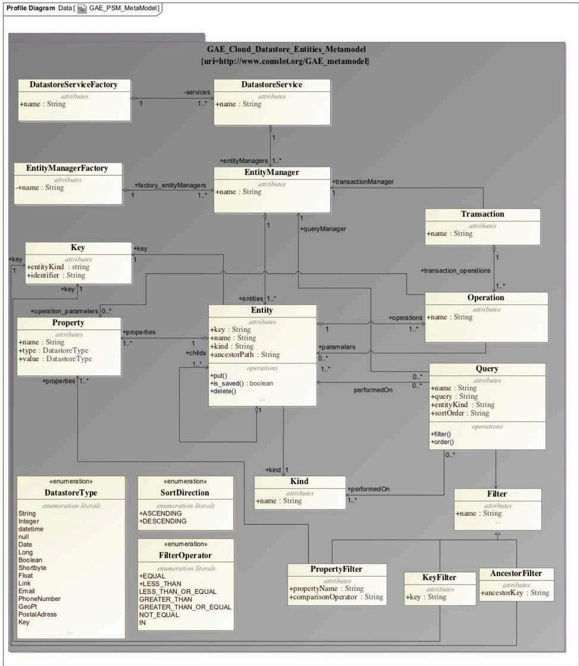
Figure 25. Méta-modèle des entités du Cloud Datastore
