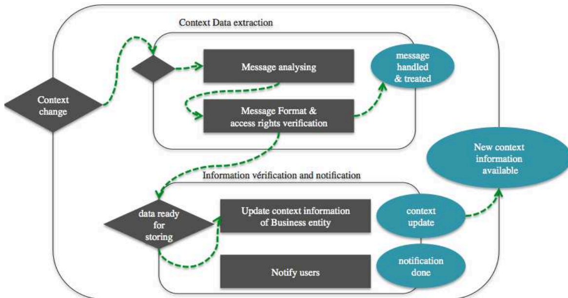
Figure 71. Traitement d'évènements et notification
