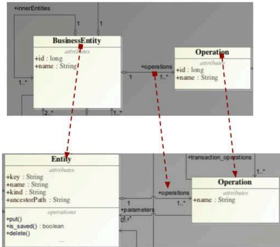
Figure 31. Mapping des operations du Business Entity vers des opérations de l'entité GAE
