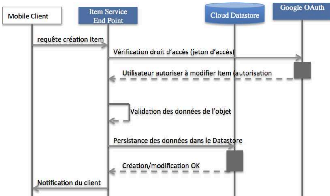
Figure 92. Diagramme de séquence de la publication /mise à jour d'un objet
