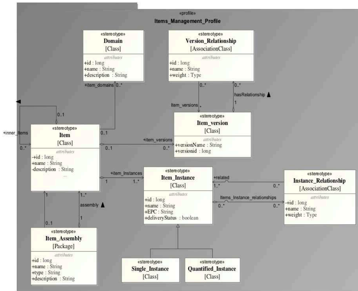
Figure 16. Profil UML des Items
