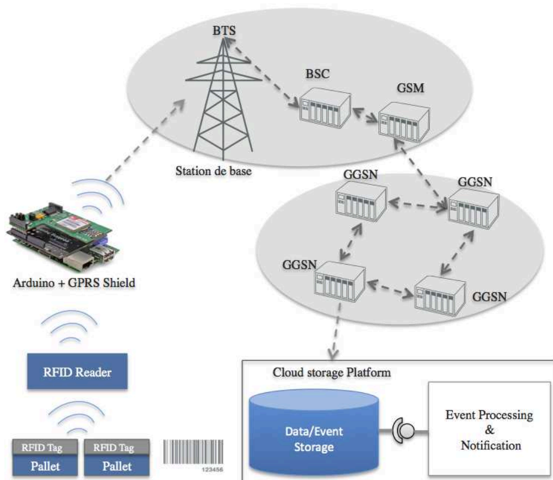
Figure 72. Transmission de données via GPRS
