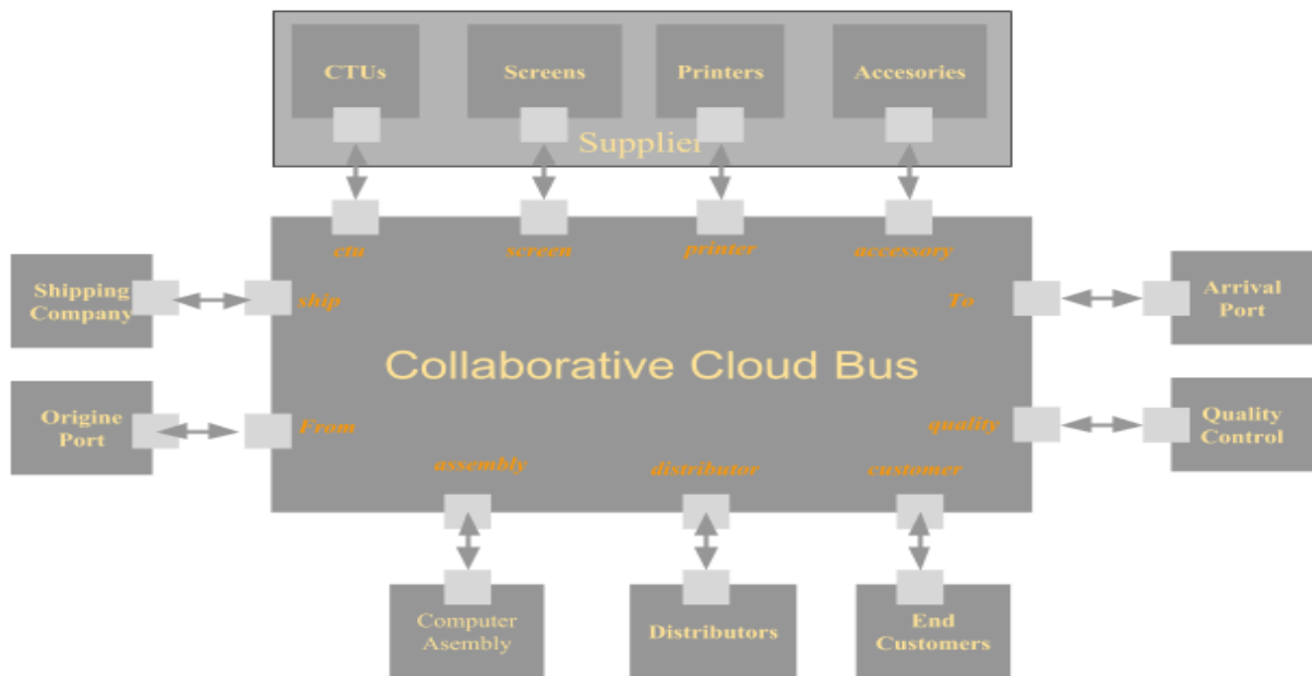
Figure 40. Chaîne logistique communicante et collaborative
