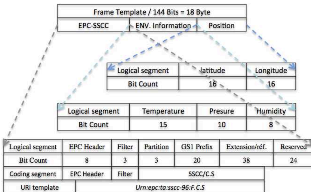
Figure 73. Format de la trame
