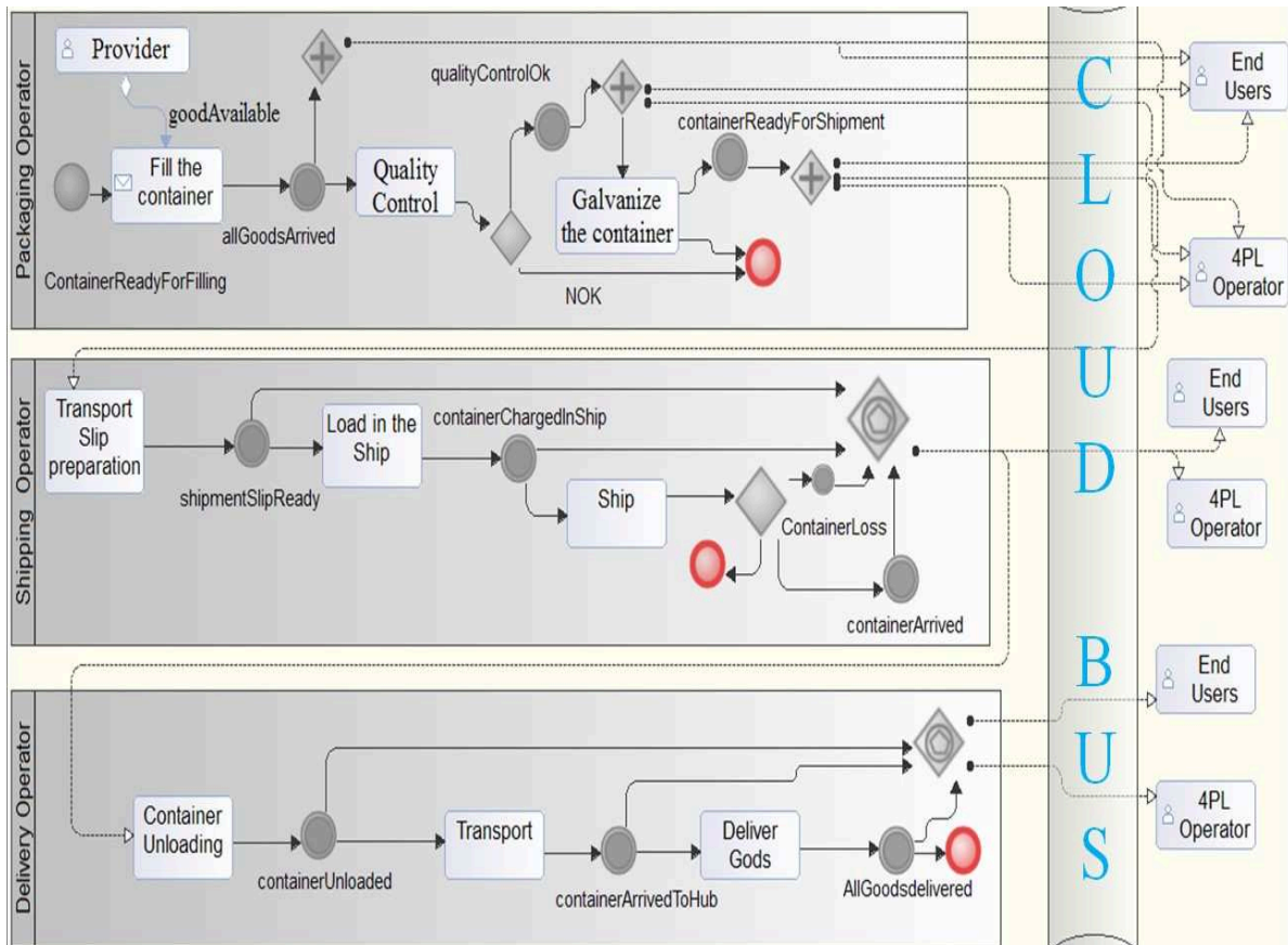
Figure 76. Diagramme BPMN du cas d'utilisation
