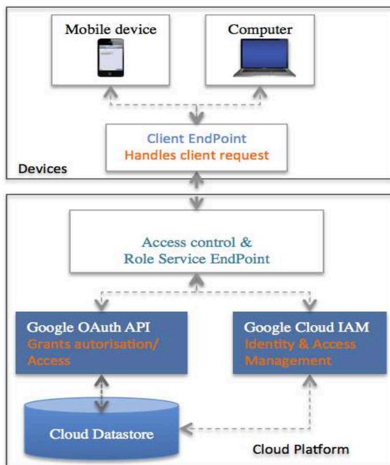
Figure 95. Architecture fonctionnelle du service de contrôle d'accès et de gestion des rôles
