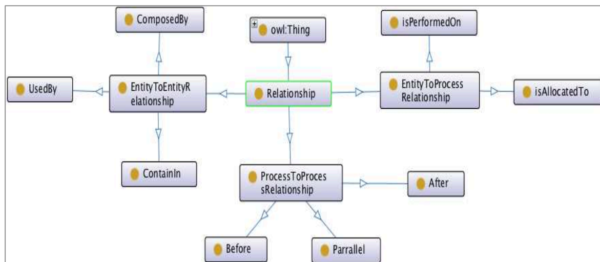
Figure 66. Ontologie des relations d'inter-dépendance (Relationship)
