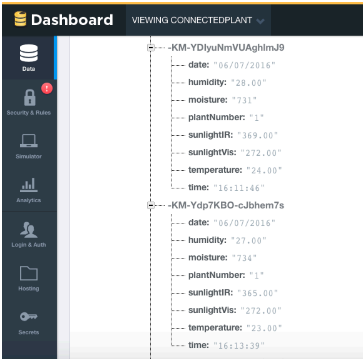
Figure 78. Acquisition des données sur le contexte du BU et stockage dans Firebase
