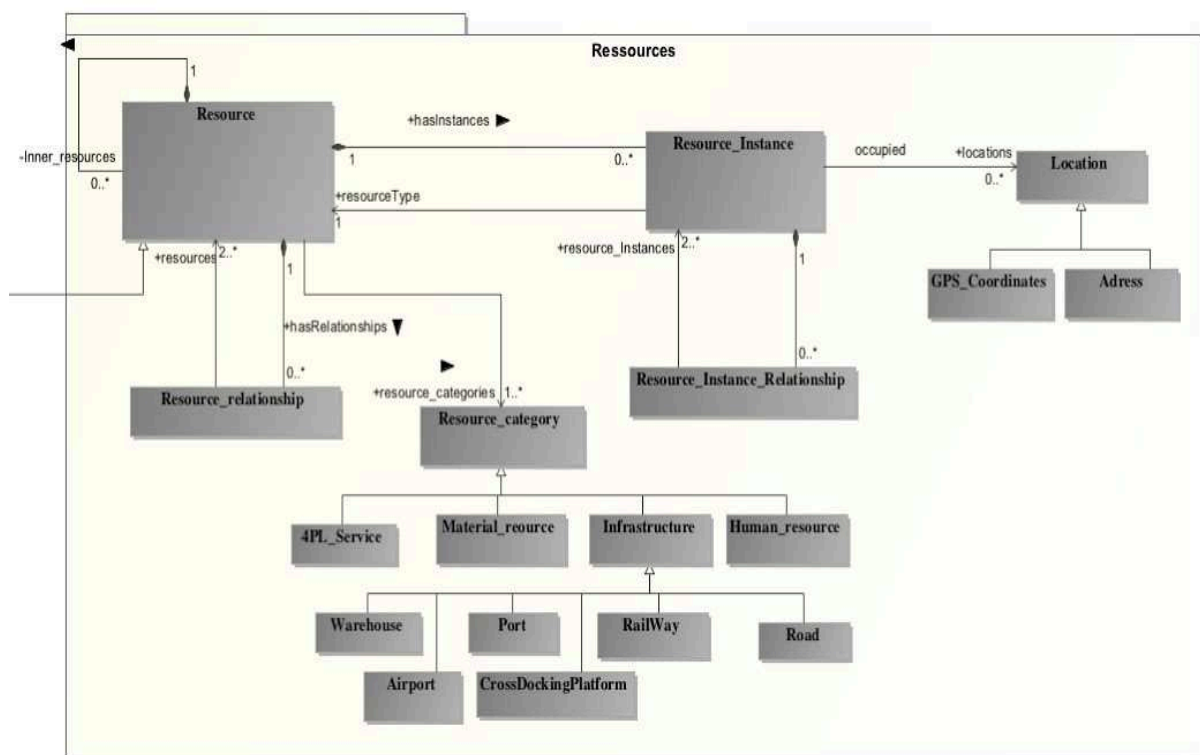
Figure 11. Méta-modèles des ressources engagées dans le processus
