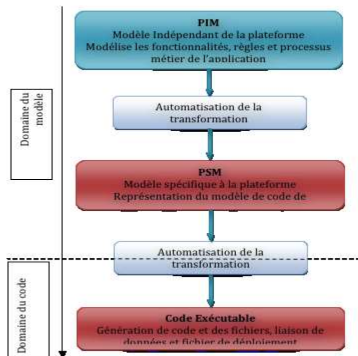
Figure 2. Architecture des modèles dans MDA
