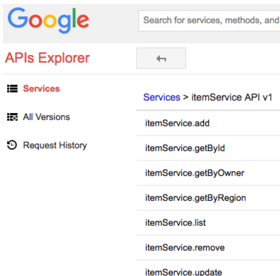
Figure 93. Service de publication des objets logistiques dans le Cloud Endpoint
