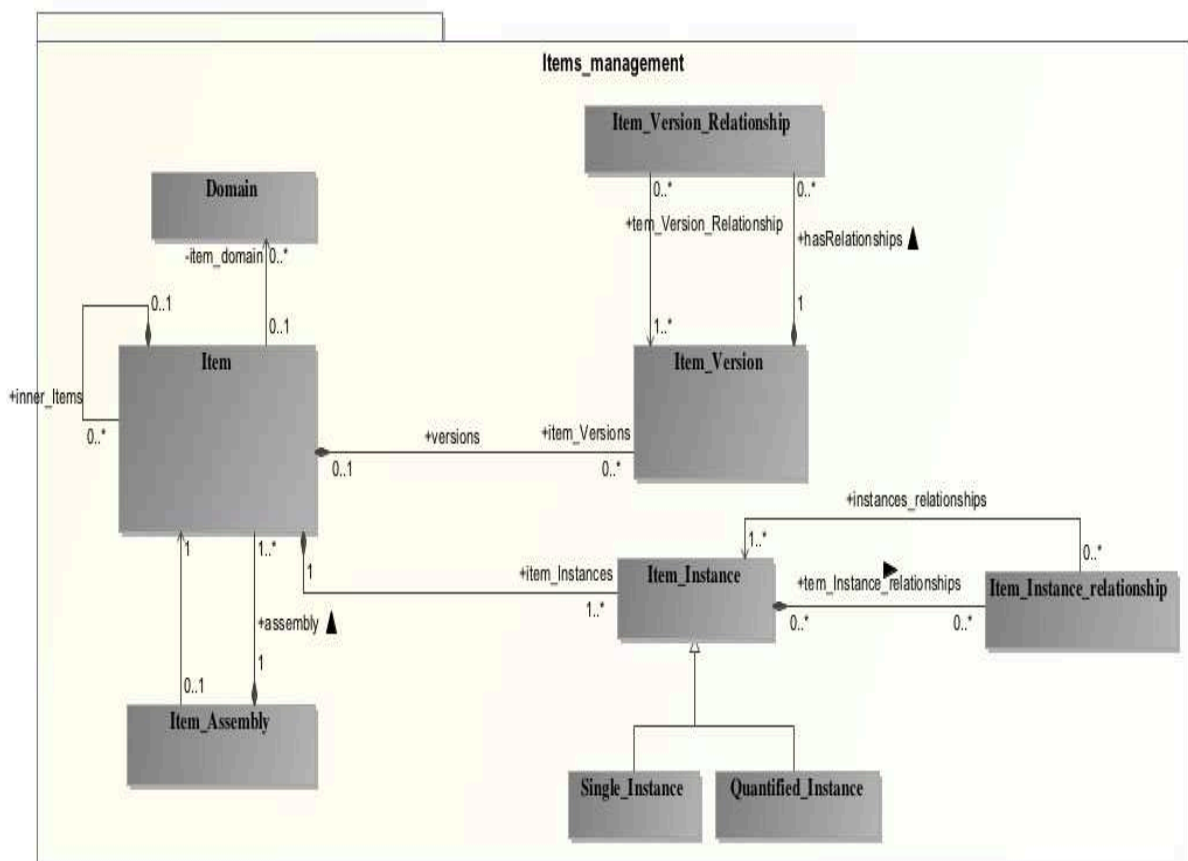
Figure 8. Diagramme du méta-modèle des Items
