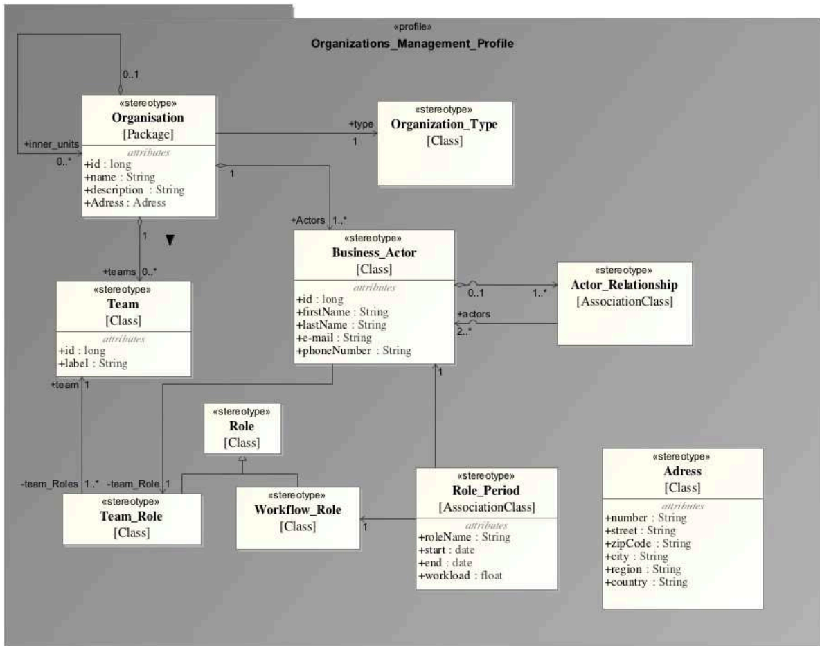
Figure 19. Profil UML pour la gestion des organisations et l’attribution des rôles
