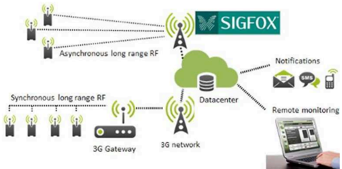
Figure 74. Architecture du réseau Sigfox 4
