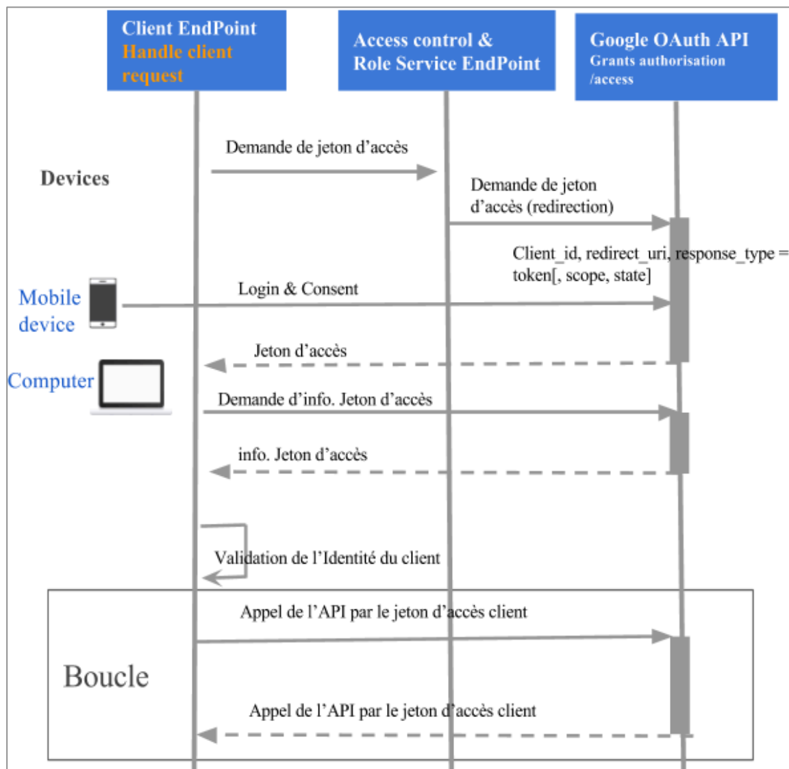
Figure 96. Séquence de fonctionnement du contrôle d'accès via Google OAuth (Cas Implicite Grant Flow)
