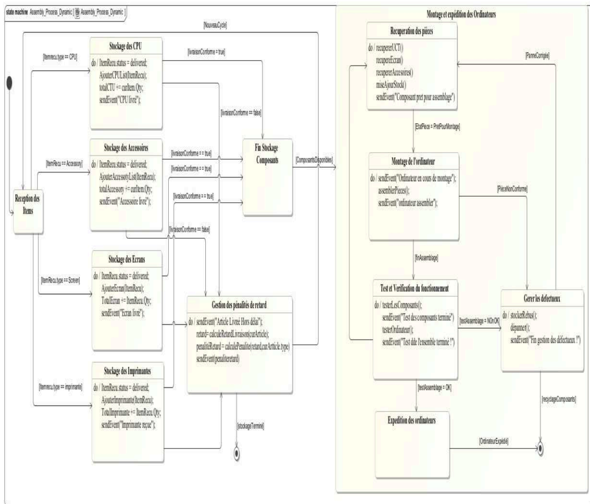
Figure 43. Diagramme d'états transition du système d'assemblage
