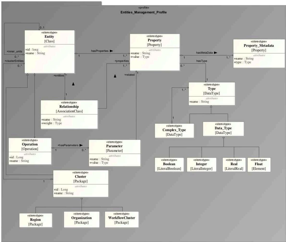
Figure 15. Profil UML des entités logistiques
