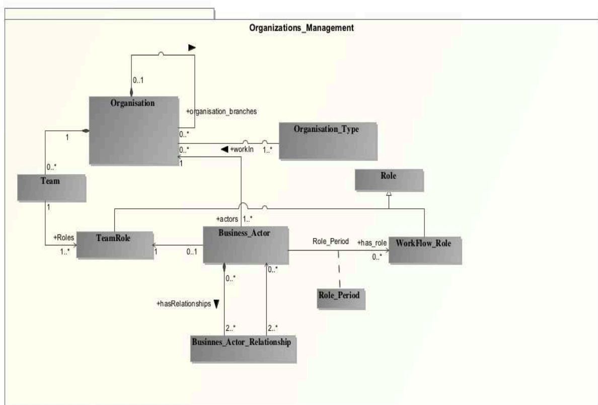
Figure 9. Méta-modèle des organisations logistiques et des acteurs impliqués dans le flux
