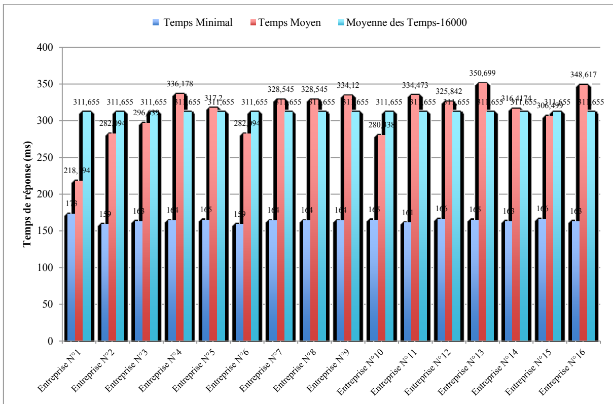
Figure 101. Comparaison des temps de réponse à la moyenne globale des 16000 requêtes
