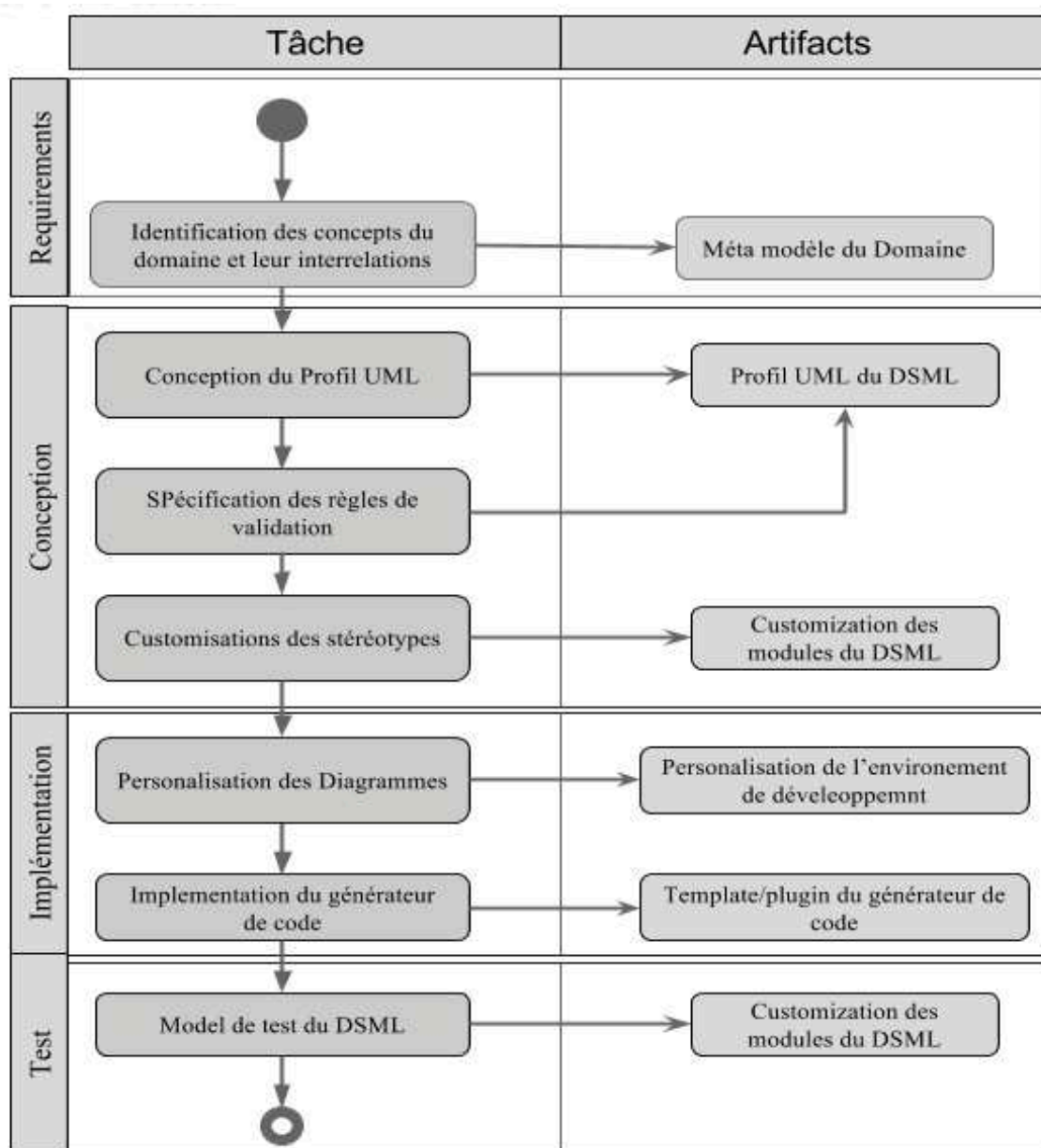
Figure 14. Les étapes de mise en oeuvre du profil UML du DSML
