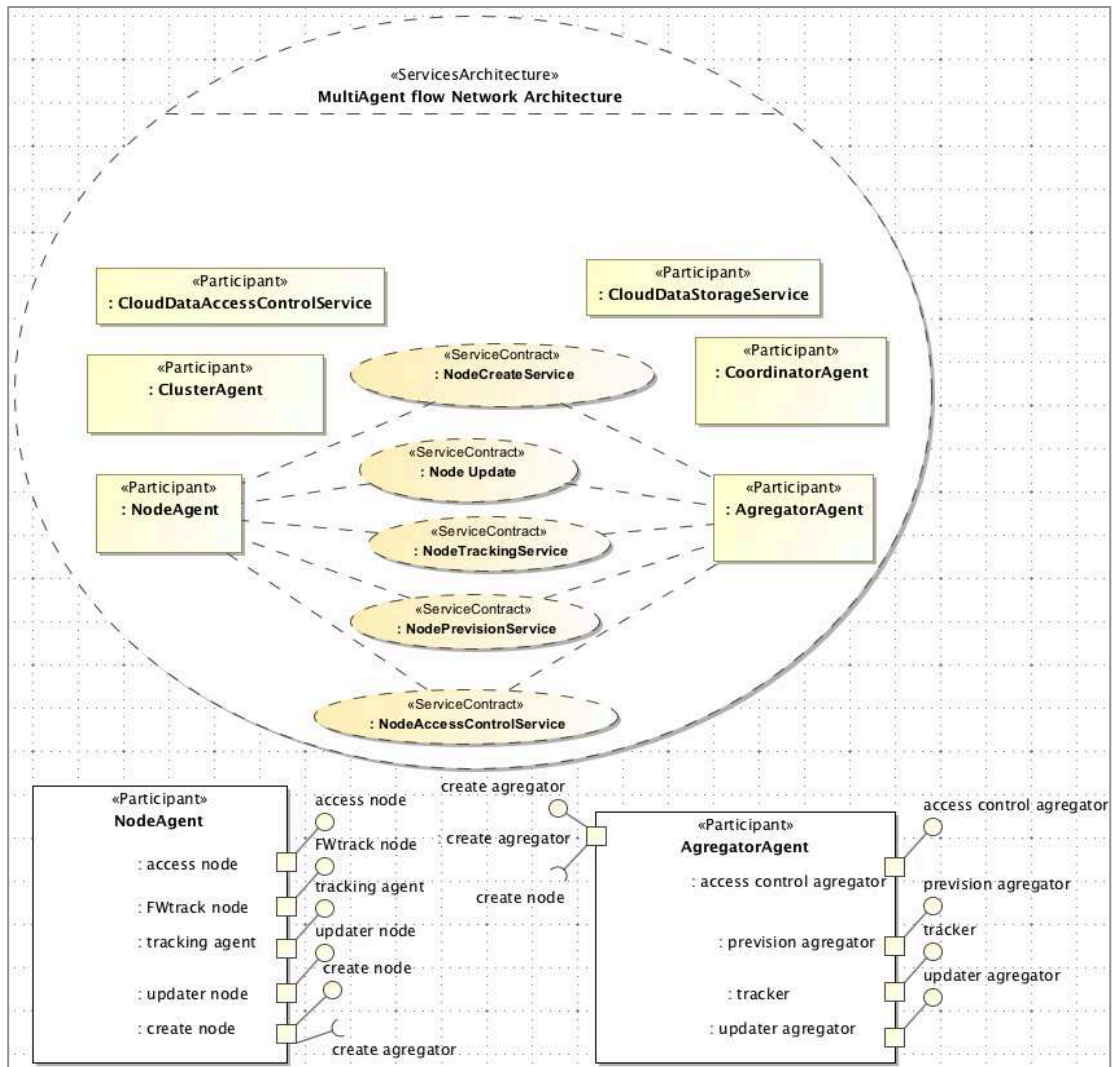
Figure 56. Architecture Orientée Service du système
