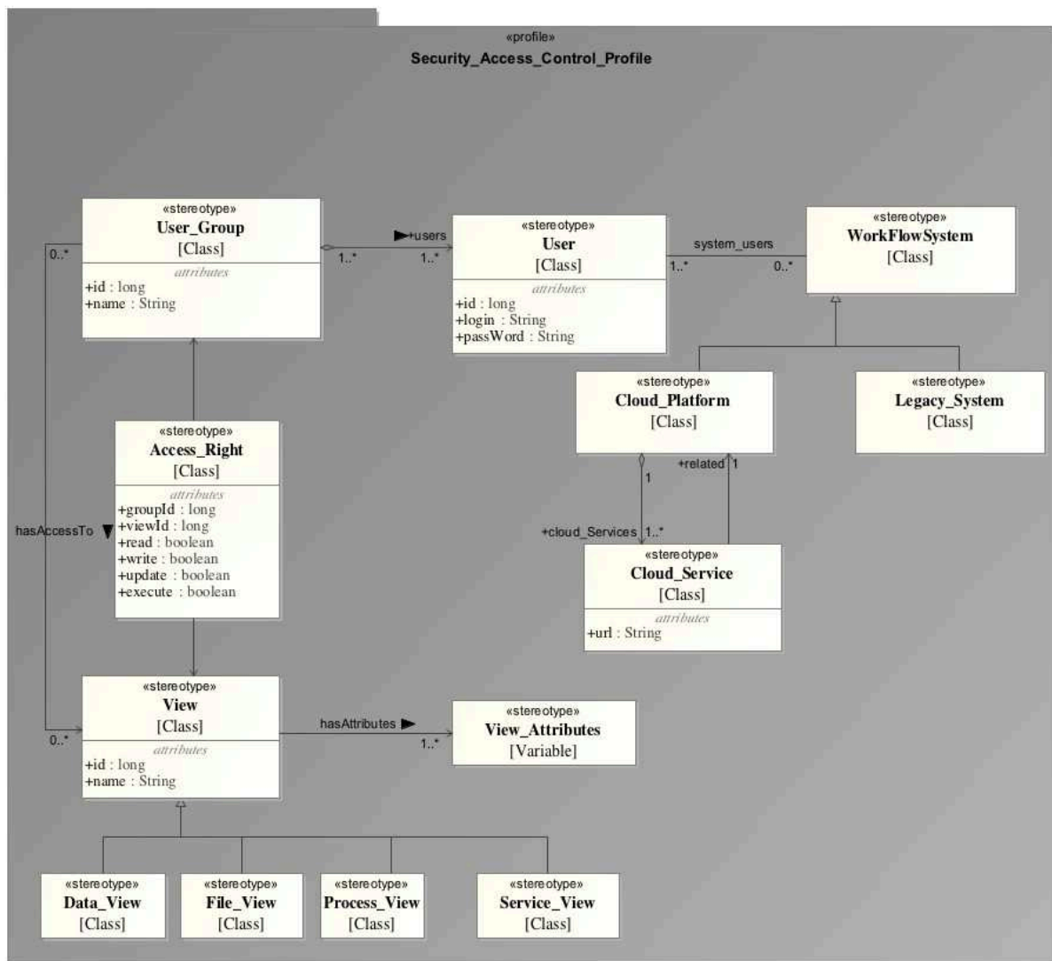
Figure 20. Profil UML pour la gestion de la sécurité et droit d'accès
