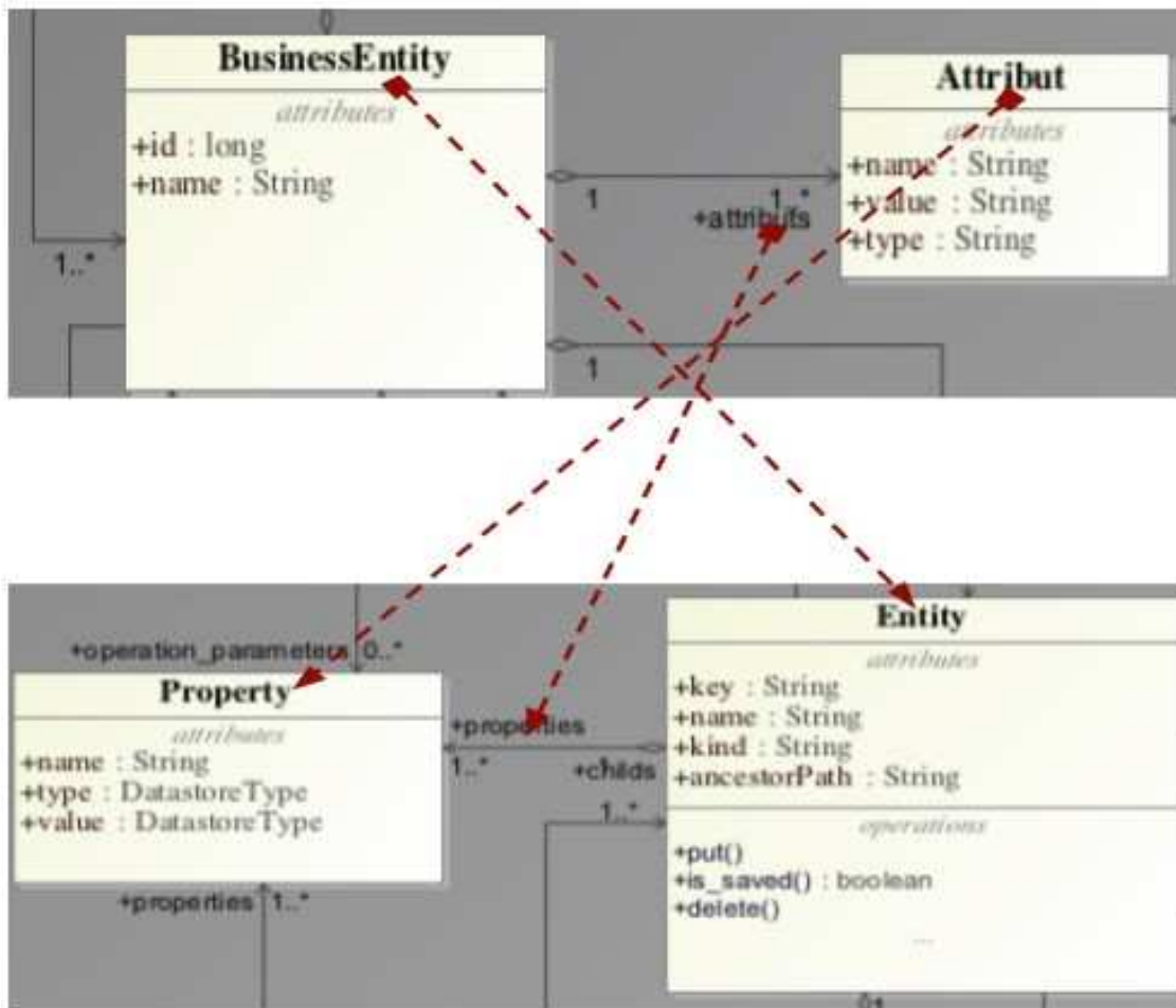
Figure 29. Mappings des Attributs aux Properties
