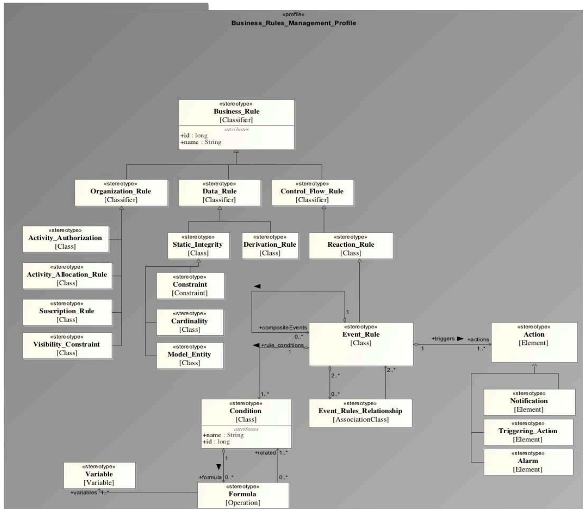
Figure 21. Profil UML pour la gestion des cotraintes et des règles metier
