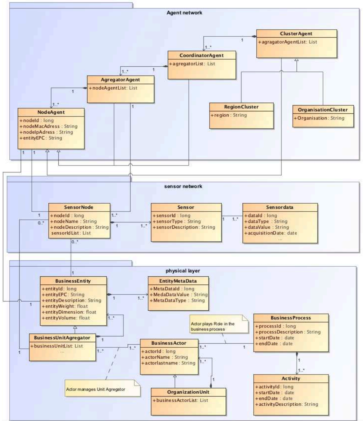
Figure 55. Schéma UML de l'architecture multi-agents
