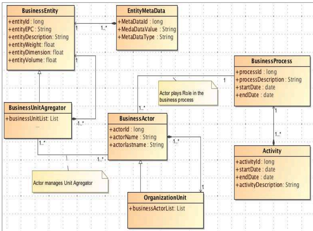
Figure 49. Diagramme UML du niveau physique du flux de marchandises
