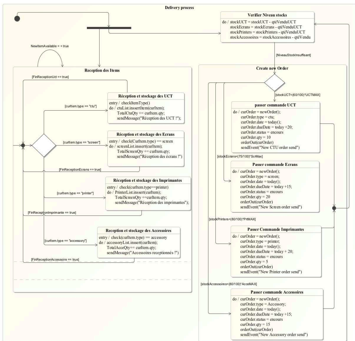
Figure 41. diagramme d'états transitions SysML du processus de distribution
