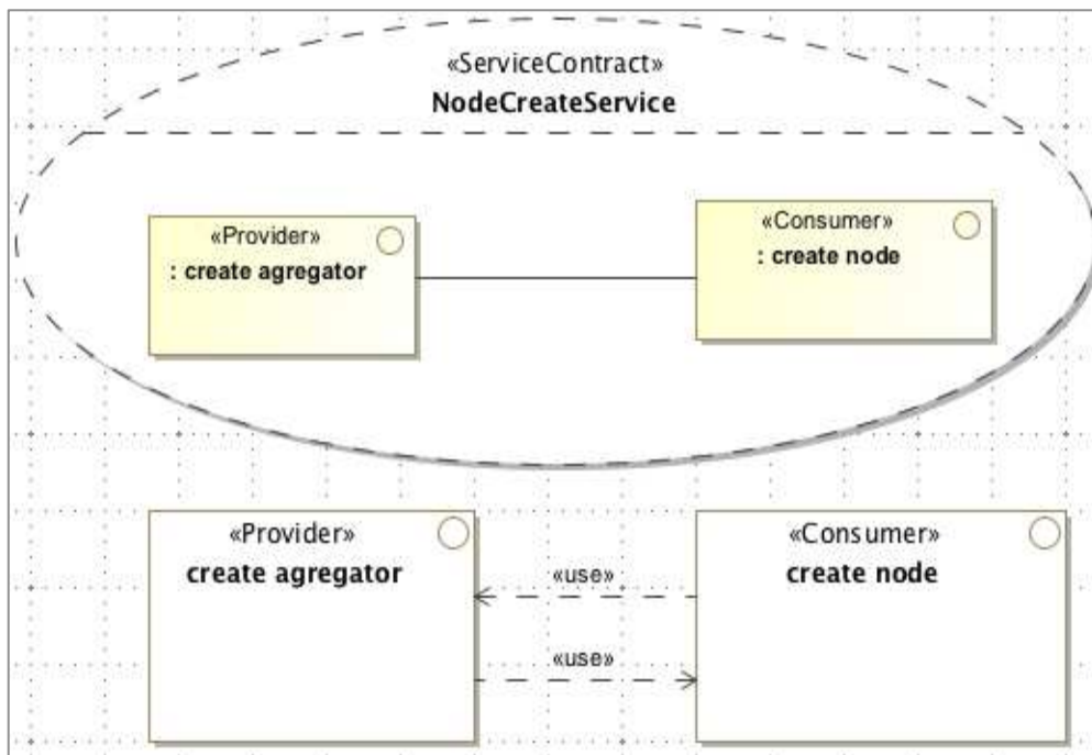
Figure 57. Service de création d'un NodeAgent
