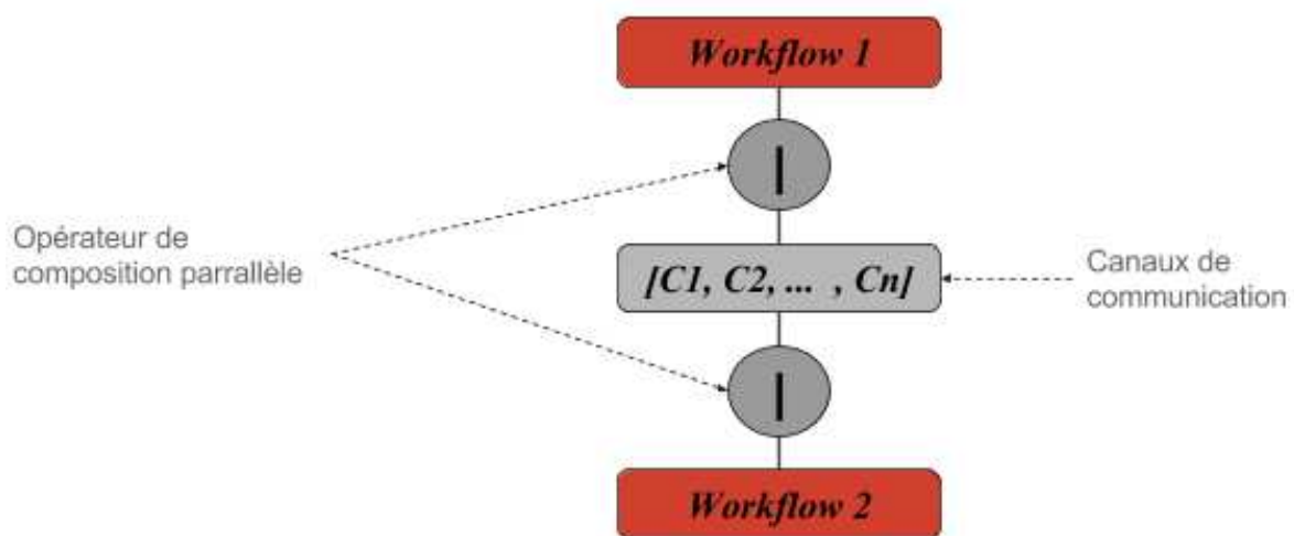
Figure 36. Opérateur de composition parallèle de workflows
