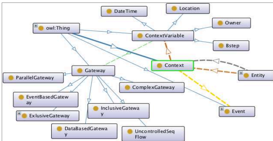
Figure 61. Ontologie du contexte du Business Entity
