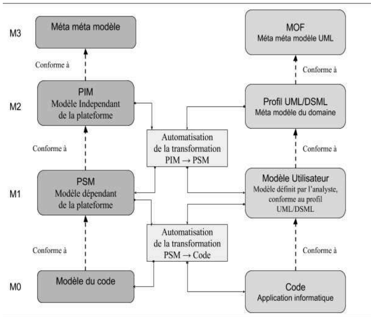
Figure 26. Niveau de méta-modélisation du MOF avec transformation
