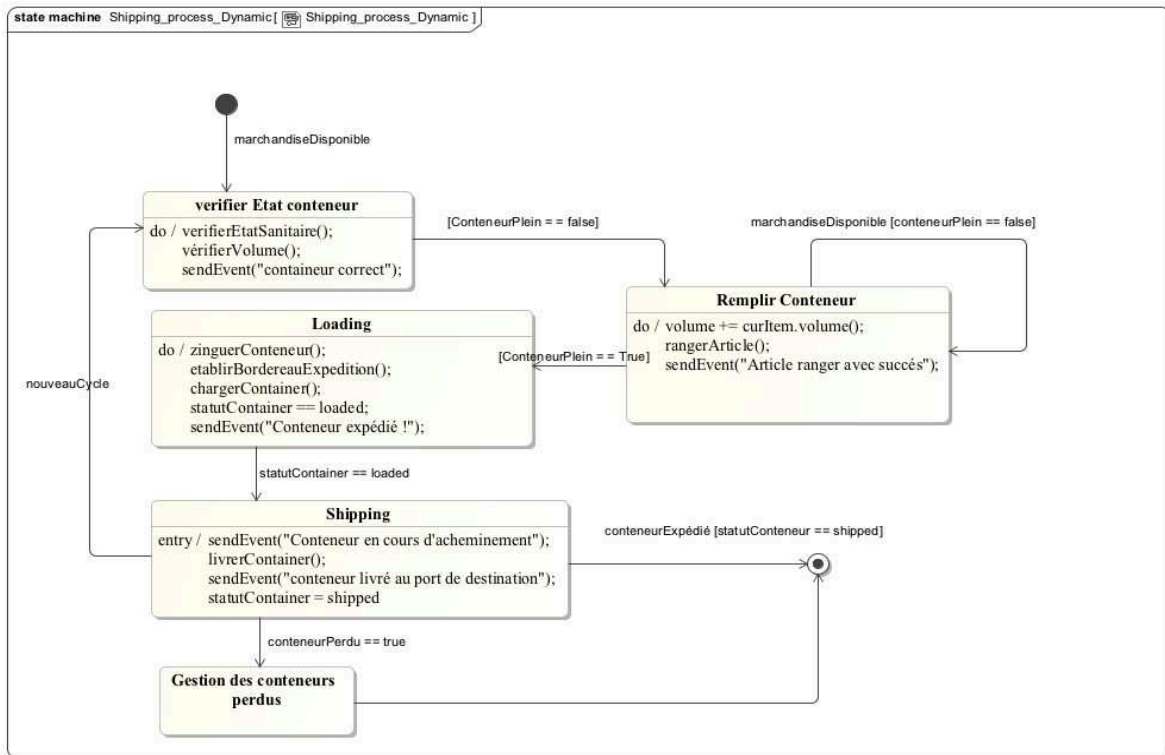
Figure 42. Diagramme d'états transition du processus de shipping
