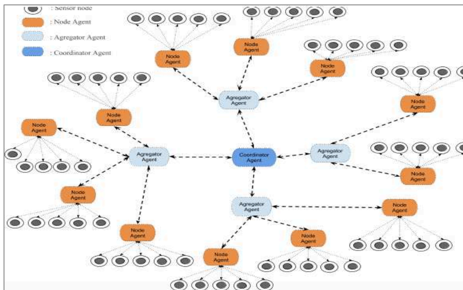
Figure 52. Architecture du système multi-agents d'intégration dans le réseau du flux physique et du réseau de capteurs
