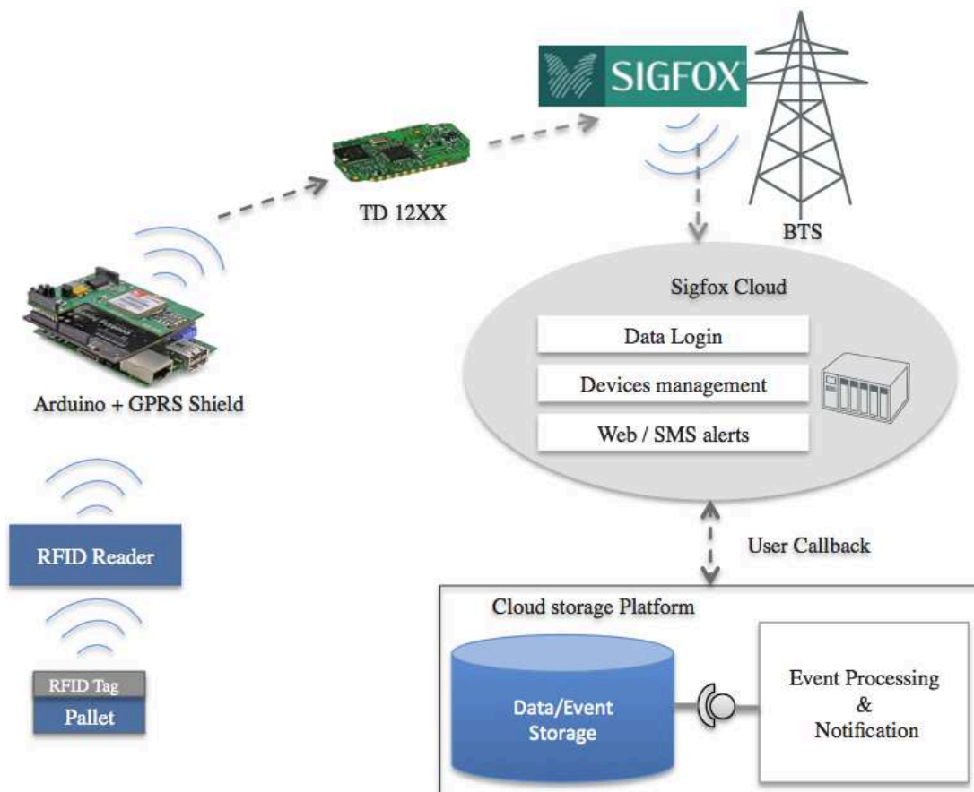
Figure 75. Transmission de données utilisant le réseau Sigfox et un module Arduino
