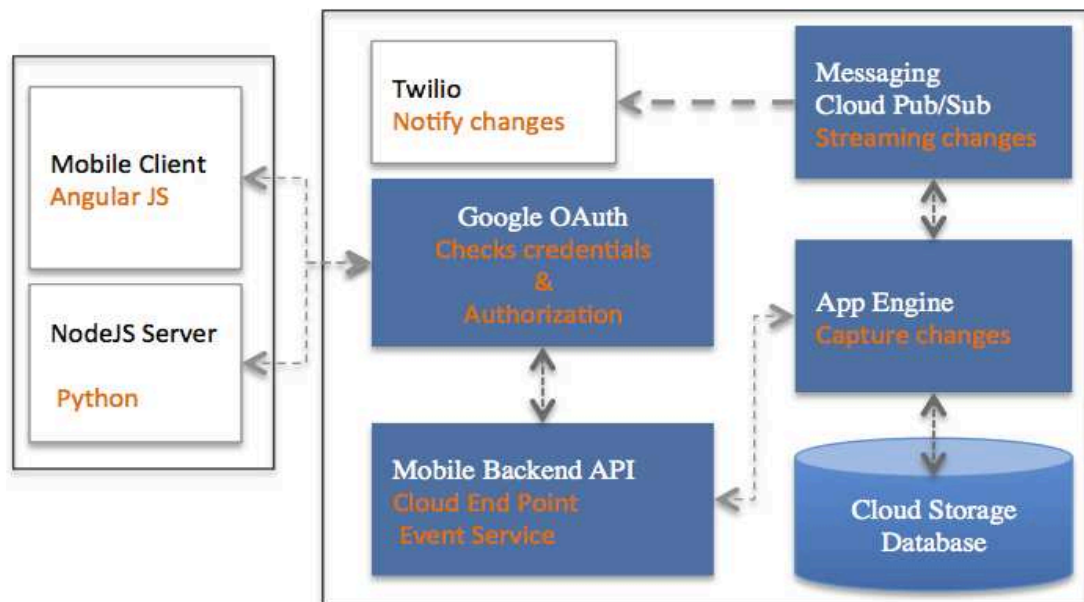
Figure 85. Architecture fonctionnelle du module de publication des événements
