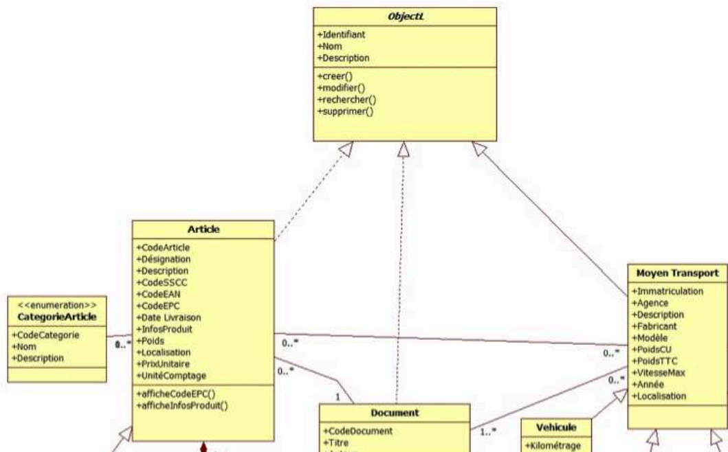
Figure 5. Exemple de diagramme UML
