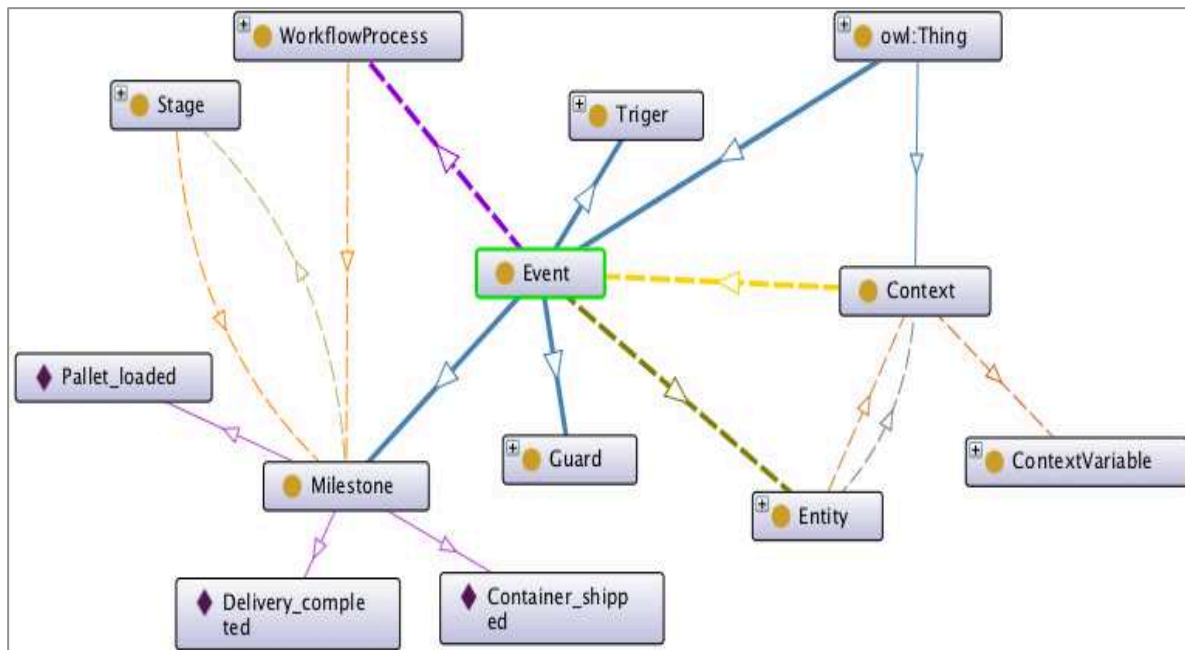
Figure 62. Ontologie des événements (Event)
