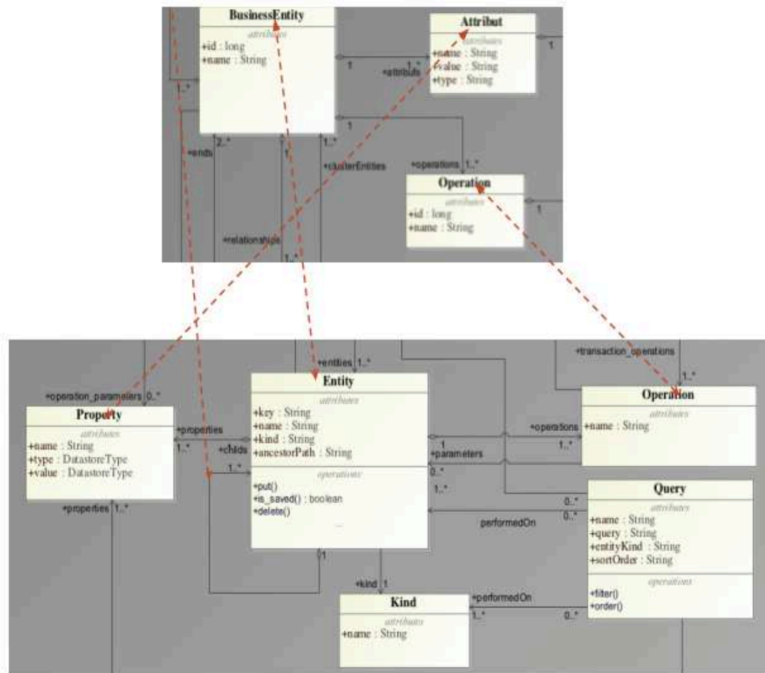
Figure 27. Mapping des entités Business aux entités du Datastore
