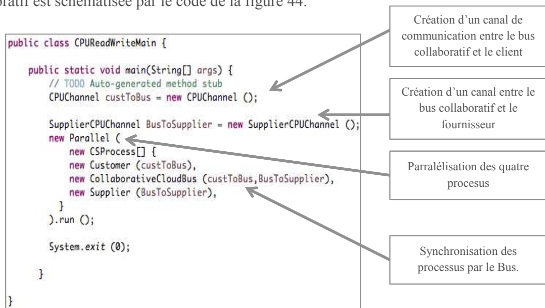
Figure 44. Synchronisation des processus client fournisseur via le bus
