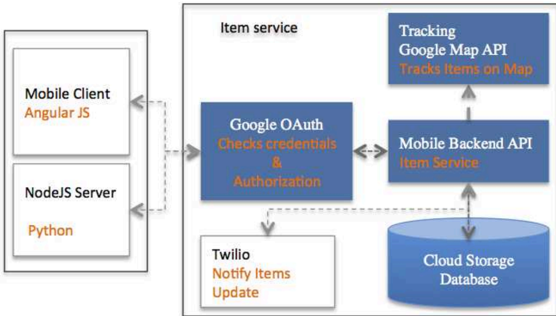
Figure 91. Architecture fonctionnelle du module de publication des objets logistiques
