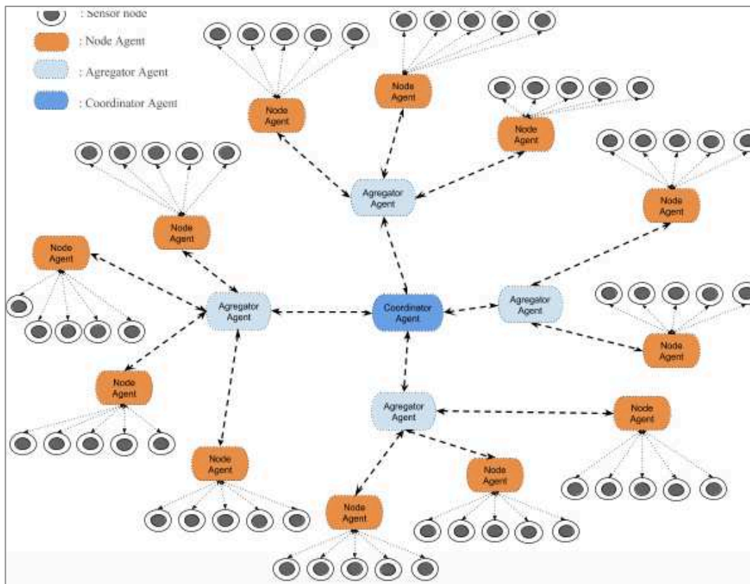
Figure 53. Réseau multi-agents
