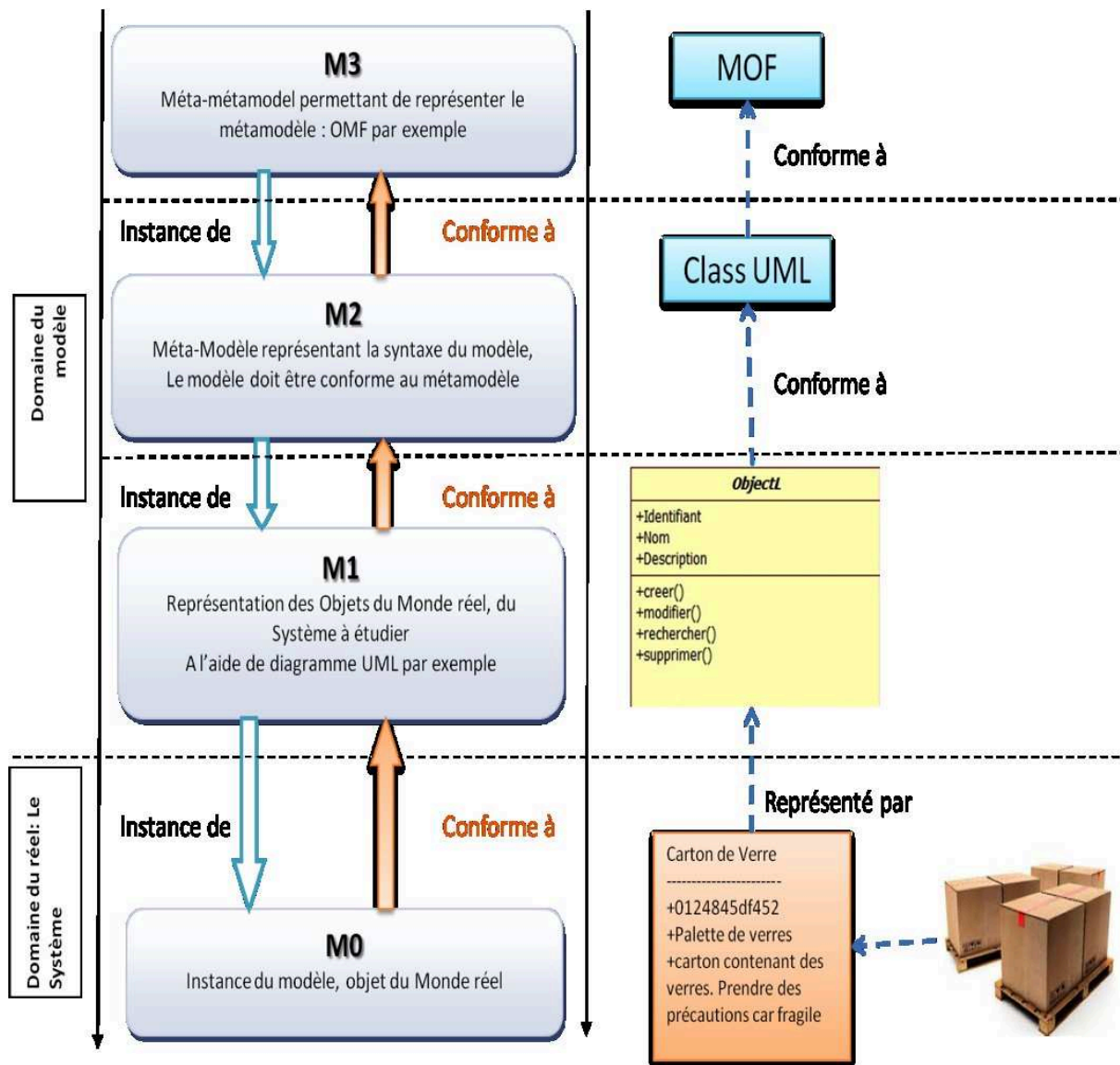
Figure 3. Les différents niveaux de méta-modélisation dans MDA
