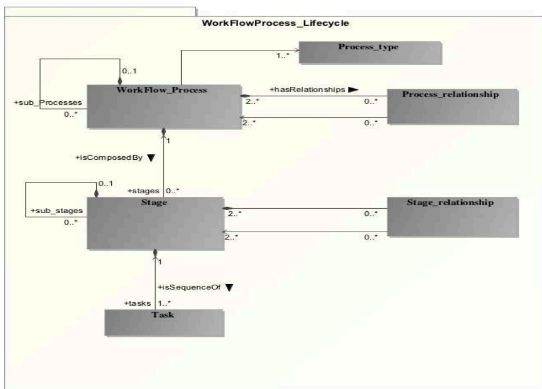
Figure 10. Méta-modèle du cycle de vie du workflow process
