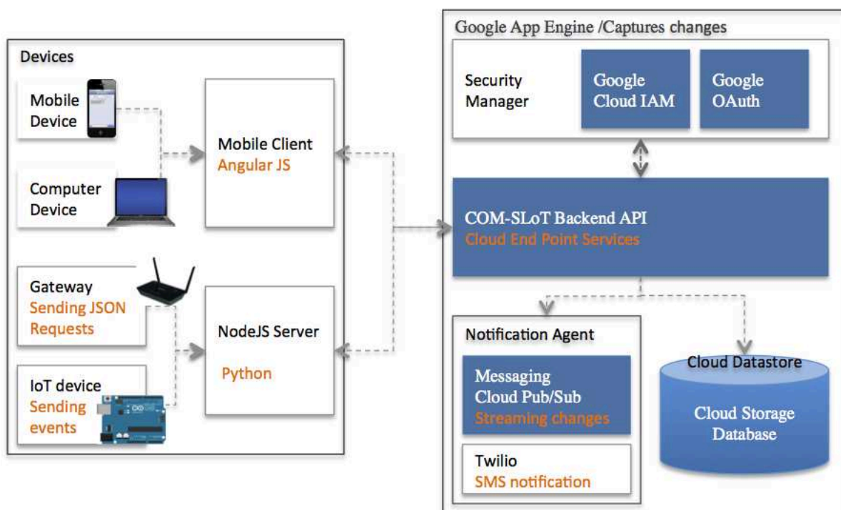
Figure 83. Architecture d'implémentation de la plateforme dans Google Cloud Platform
