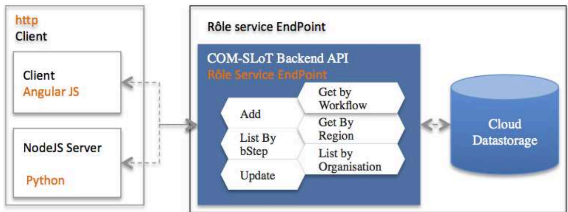
Figure 94. EndPoint du service de gestion des Acteurs et des organisations
