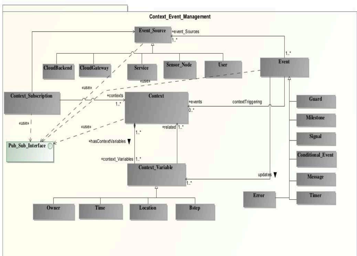
Figure 13. Méta-modèle des événements liés au contexte du workflow process
