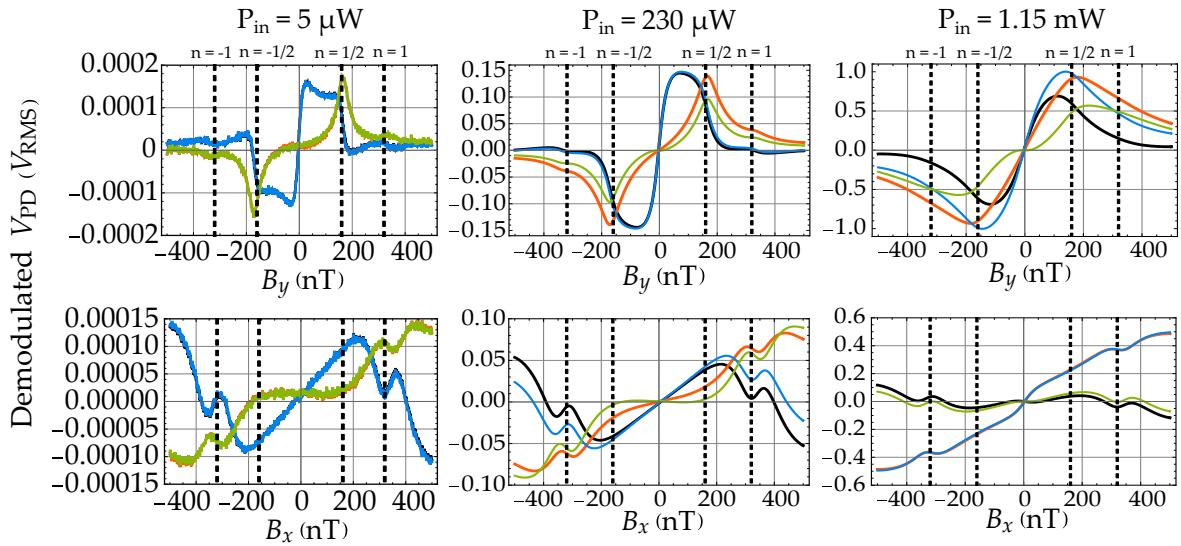
FIGURE 0.7 : Résonances paramétriques observées avec deux champs RF pour les composantes B_y et B_x à différentes puissances optiques. Ligne du haut : Résonances en fonction de B_y , signal démodulé à 9 kHz. Ligne du bas : Résonances en fonction de B_x , signal démodulé à 9 kHz du signal démodulé à 40 kHz. Pour toutes les figures : les courbes noires et oranges représentent les composantes en phase et en quadrature, respectivement, du signal démodulé avec la phase de détection synchrone réglée à faible puissance optique. Les courbes bleues et vertes représentent les composantes en phase et en quadrature, respectivement, du signal démodulé avec modification de la phase de détection synchrone afin d'annuler la pente sur la composante en quadrature du signal démodulé. Les lignes verticales tiretées montre les valeurs n \Omega / \gamma .
