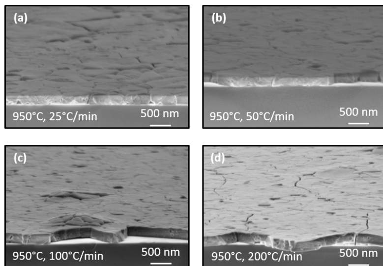
FIGURE 2.11 – Observation MEB des échantillons recuits à 950^\circ\text{C} pour différentes rampes de montées en température de (a) 25, (b) 50, (c) 100 et (d) 200^\circ\text{C}\cdot\text{min}^{-1} .
