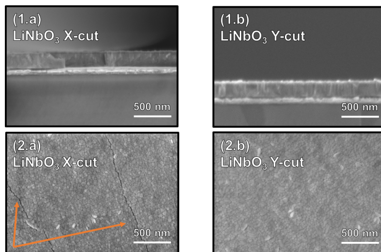
FIGURE 4.9 – Observation MEB en (1) vue de coupe et (2) vue de dessus des couches de LiNbO 3 déposées sur substrats LiNbO 3 (a) X-cut et (b) Y-cut avec une électrode de Pt.
