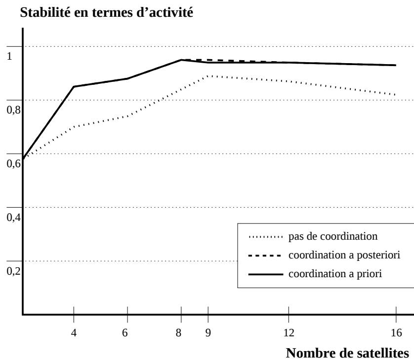
FIGURE 5.13 – Stabilité de la constellation
