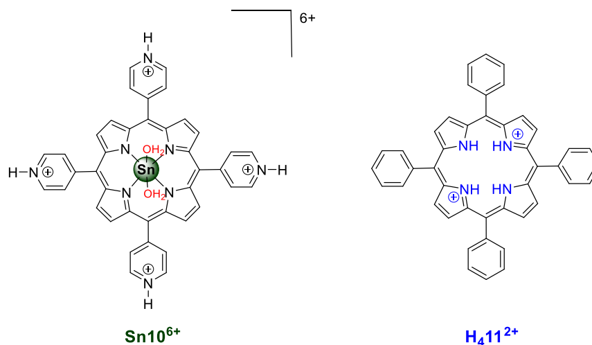
Figure 25 : Les porphyrines cationiques synthétisées par Kim ( SnX 6+ ) et par Asif ( H 4 X 2+ )
