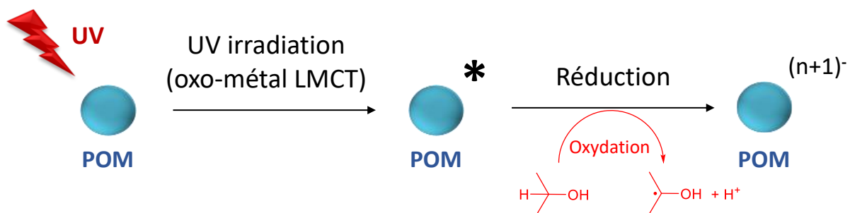
Figure 11 : Processus redox des POMs photoexcités
