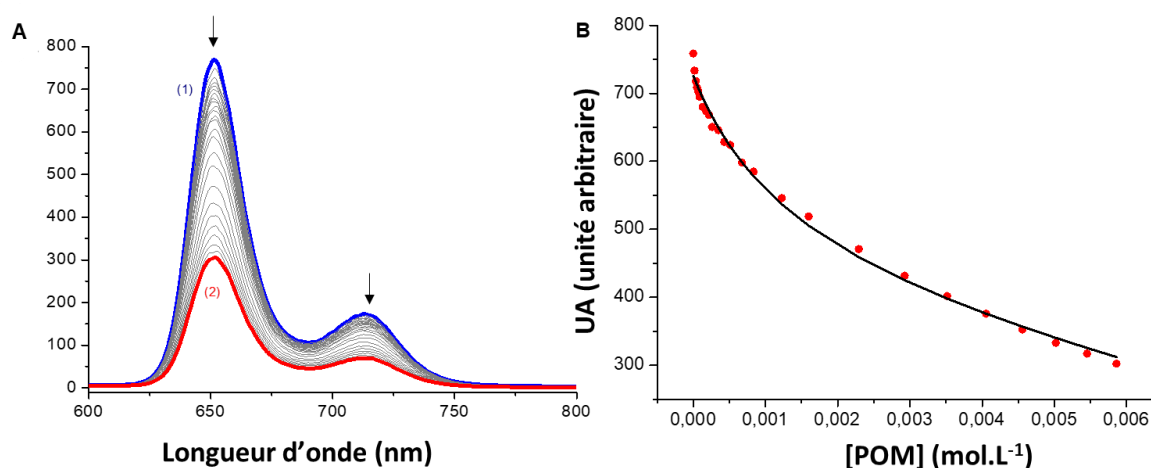
Figure 102 : A) Titrage par émission de fluorescence de 40 par [\text{Mo}_6\text{O}_{19}][(\text{n-Bu})_4\text{N}]_2 . Solvant : DMF, T = 25,0 \text{ }^\circ\text{C} , \lambda_{\text{ex}} = 517 \text{ nm} , largeurs de fente d'émission et d'excitation 20 nm, (1) [\mathbf{40}] = 4,39 \cdot 10^{-6} \text{ M} ; (2) [\text{POM}] / [\mathbf{40}] = 2000 . B) Variation de l'intensité de l'émission à 657 nm en fonction de la concentration de [\text{Mo}_6\text{O}_{19}][(\text{n-Bu})_4\text{N}]_2 . Les spectres d'émission de fluorescence ne sont pas corrigés de la dilution
