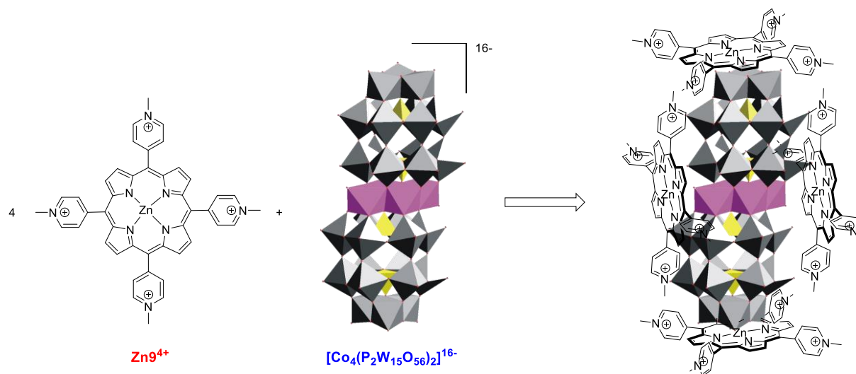
Figure 24 : Représentation schématique proposée par Ruhlmann du complexe électrostatique 4 : 1 formé entre la meso-tétrakis(N-méthyl-4-pyridium)porphyrine de zinc et le POM
