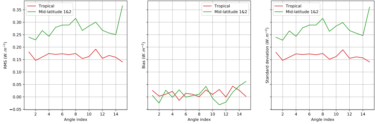
FIGURE 4.21 – Statistiques sur la base d'évaluation des 30 PMC sélectionnés en fonction de l'angle de visée pour les deux types de masse d'air (tropicale et tempérée). Les trois figures partagent la même échelle des ordonnées.
