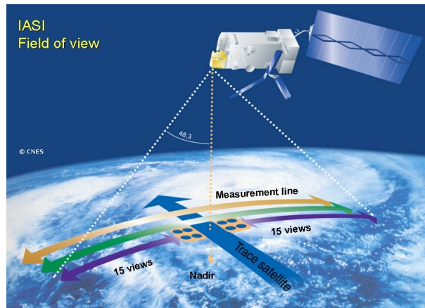
FIGURE 1.8 – Géométrie de balayage de l’instrument IASI (Source : CNES).
