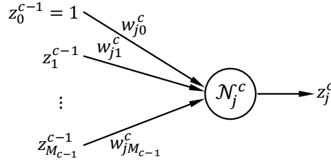
FIGURE 4.1 – Représentation schématique du neurone formel. Il s'agit du j^{\text{ième}} neurone noté \mathcal{N}_j^c , situé en c^{\text{ième}} couche d'un PMC. Les sorties des M_{c-1} neurones de la couche c - 1 sont notées (z_i^{c-1})_{1 \leq i \leq M_{c-1}} avec une entrée unitaire supplémentaire notée z_0^{c-1} pour la représentation du biais. Les synapses reliant les neurones de la couche c - 1 au neurone j de la couche c sont affectées des poids synaptiques notés (w_{ji}^c)_{0 \leq i \leq M_{c-1}} . La sortie du neurone \mathcal{N}_j^c est notée z_j^c .
