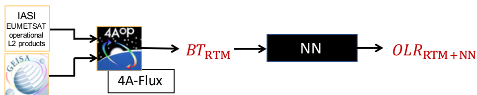
FIGURE 4.14 – Représentation schématique de l'approche RTM+NN. BT_{RTM} est le spectre de température de brillance simulé par 4A/OP tel que le mesurerait IASI.
