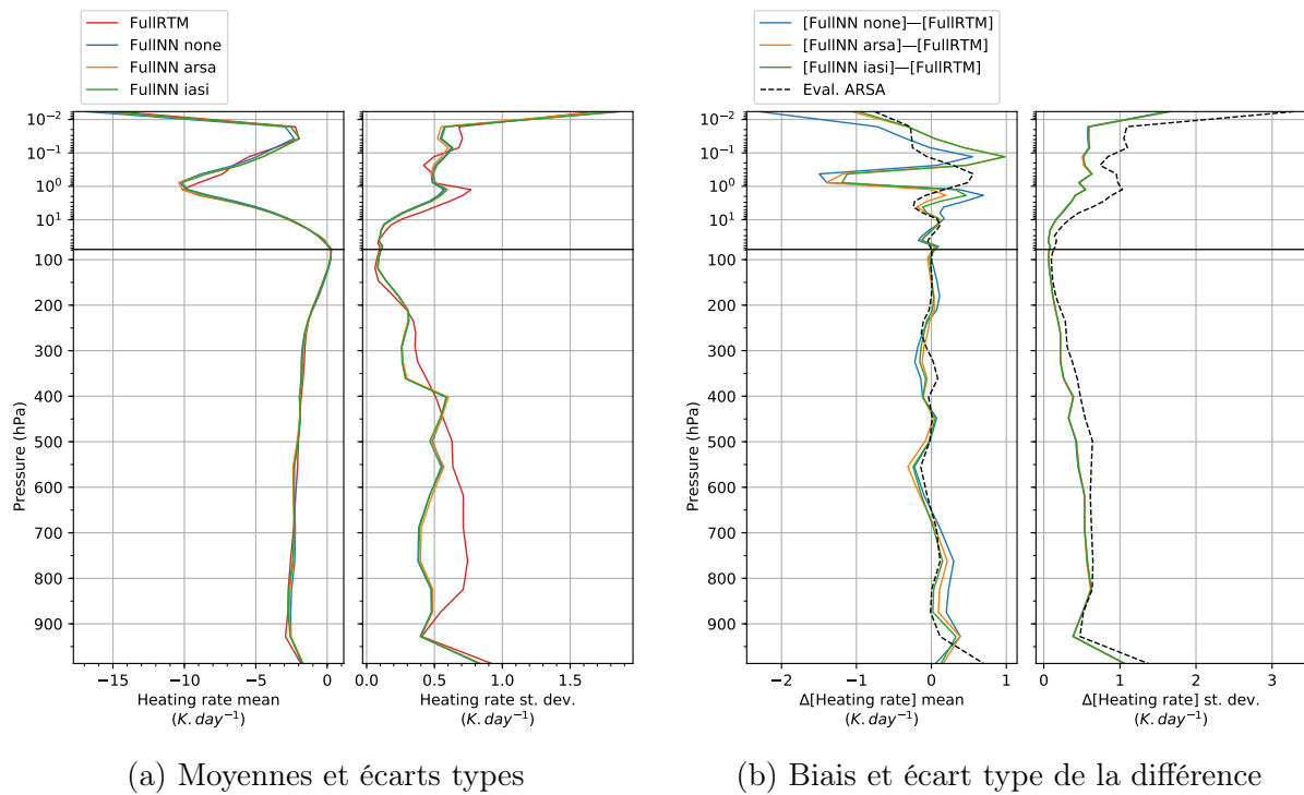
FIGURE 5.15 – Comparaison entre les approches FullNN et FullRTM pour l'estimation du profil de taux de chauffage. Moyennes ((a) gauche) et écarts types ((a) droite) des profils de taux de chauffage sur les 542 situations pour chacune des deux approches. Biais ((b) gauche) et écart type des différences ((b) droite) entre les approches FullNN et FullRTM. Les résultats FullNN sont donnés en absence de prétraitement (bleu), avec prétraitement ARSA (orange) et IASI (vert). En traits pointillés sont reportés le biais et l'écart type obtenus sur la base d'évaluation ARSA.
