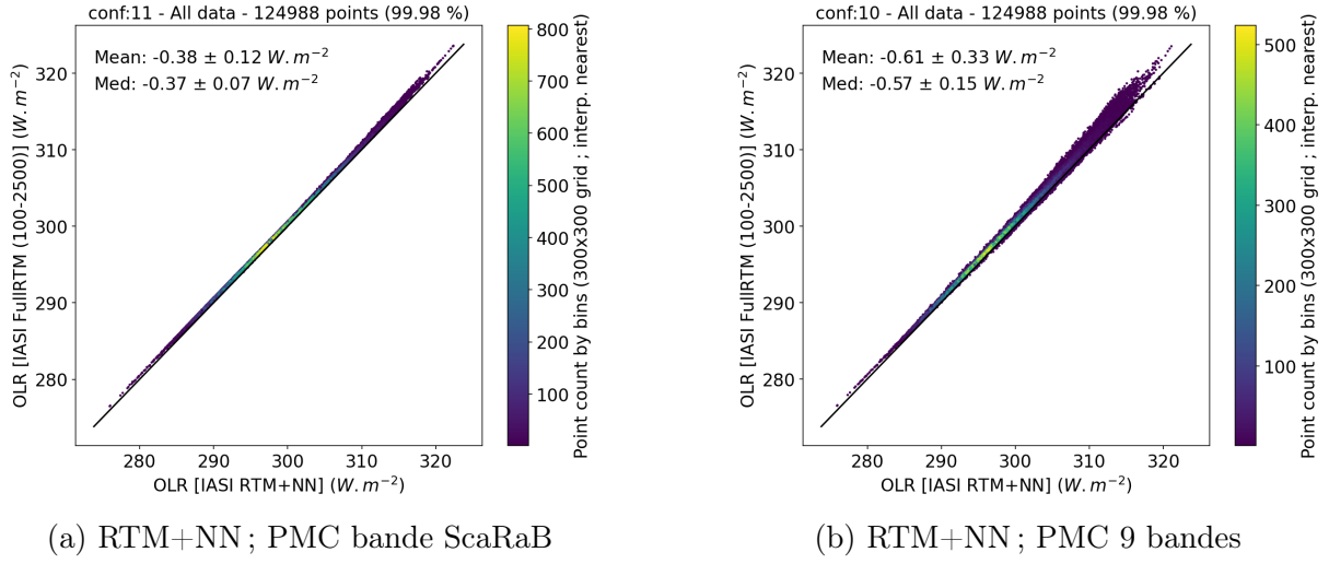
FIGURE 4.17 – Diagramme de dispersion et statistiques des OLR IASI estimés avec l’approche RTM+NN (abscisses) comparés à l’approche FullRTM (ordonnées) pour deux architectures de PMC différentes. (a) : Le PMC utilisé est celui avec pour sortie l’OLR sur la bande spectrale 100 – 2500 \text{cm}^{-1} . (b) : Le PMC utilisé est celui avec 9 sorties dont 7 sorties sont additionnées pour obtenir l’OLR sur la bande spectrale 100 – 2500 \text{cm}^{-1} . Les statistiques des différences [RTM + NN] – [FullRTM] sont la moyenne et l’écart type en première ligne et la médiane et l’écart type robuste en deuxième ligne.
