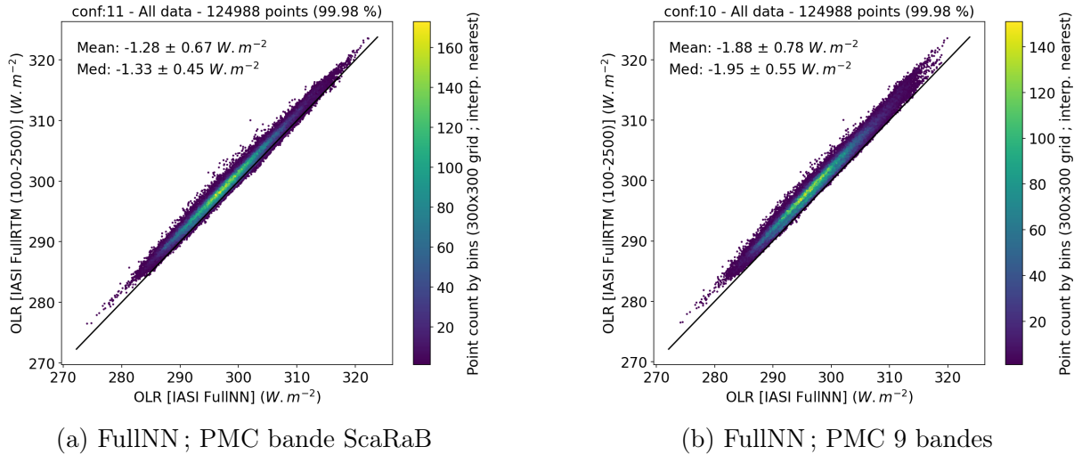
FIGURE 4.18 – Diagramme de dispersion et statistiques des OLR IASI estimés avec l’approche FullNN (abscisses) comparés à l’approche FullRTM (ordonnées) pour deux architectures de PMC différentes. (a) : Le PMC utilisé est celui avec pour sortie l’OLR sur la bande spectrale 100 – 2500 \text{cm}^{-1} . (b) : Le PMC utilisé est celui avec 9 sorties dont 7 sorties sont additionnées pour obtenir l’OLR sur la bande spectrale 100 – 2500 \text{cm}^{-1} . Les statistiques des différences [FullNN] – [FullRTM] sont la moyenne et l’écart type en première ligne et la médiane et l’écart type robuste en deuxième ligne.
