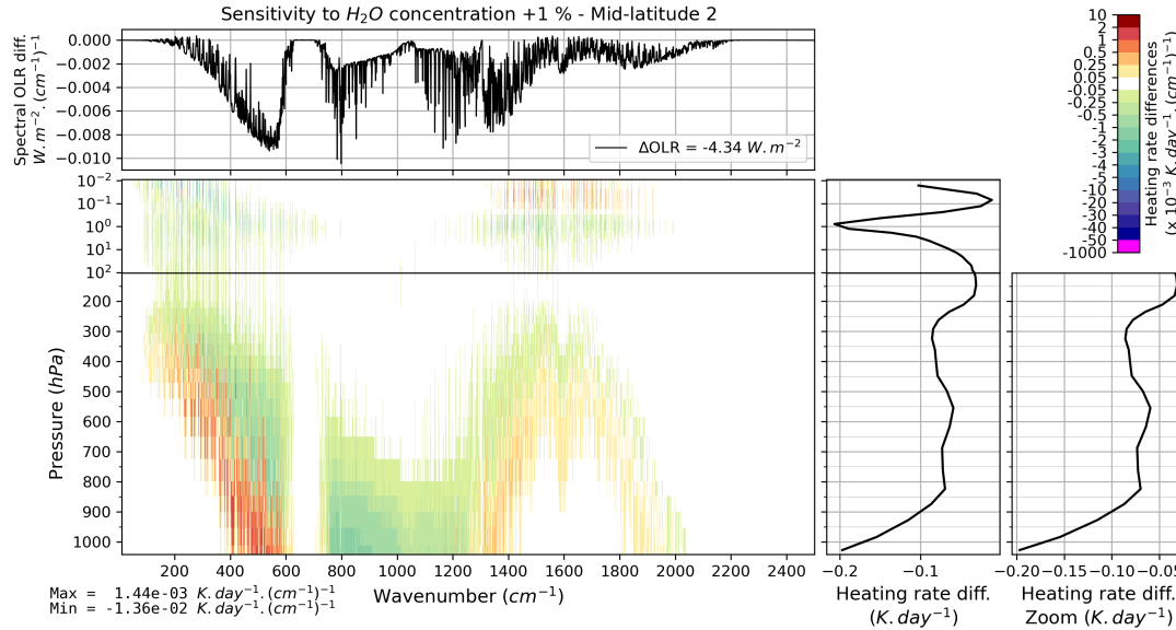
FIGURE B.33 – Effet d’une augmentation verticalement uniforme de 1 % de la concentration de vapeur d’eau sur l’OLR et le taux de chauffage vertical pour l’atmosphère moyenne Mid-latitude 2 de TIGR 2000.
