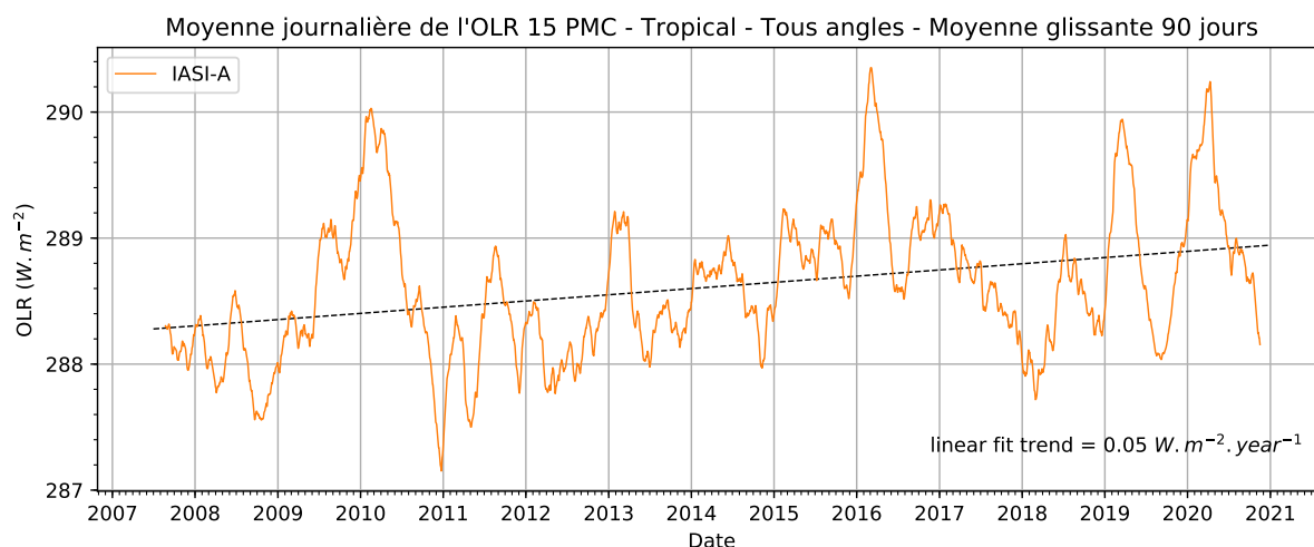
FIGURE 5.2 – Série temporelle de la moyenne journalière des OLR (ciel-clair, nuit, océans) estimés par l'ensemble des PMC en atmosphère tropicale uniquement pour tous les angles de vue de IASI. Une régression linéaire est montrée par la courbe en pointillé. Un lissage de la série est réalisé sur 90 jours glissants.
