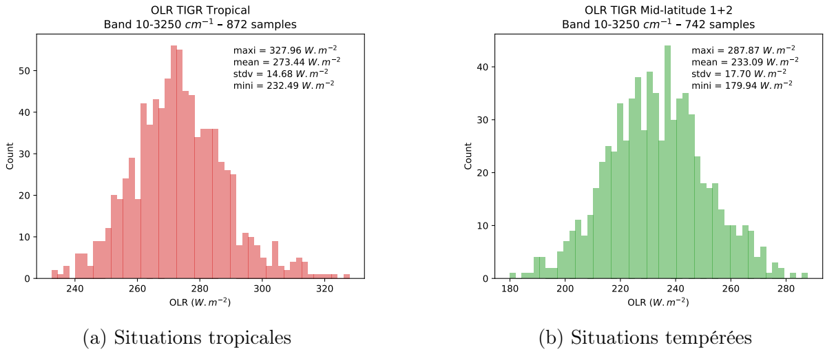
FIGURE 4.7 – Histogrammes des OLR simulés par l'approche avec 4A-Flux à partir de la base TIGR sur la bande spectrale 10 – 3250 \text{cm}^{-1} .
