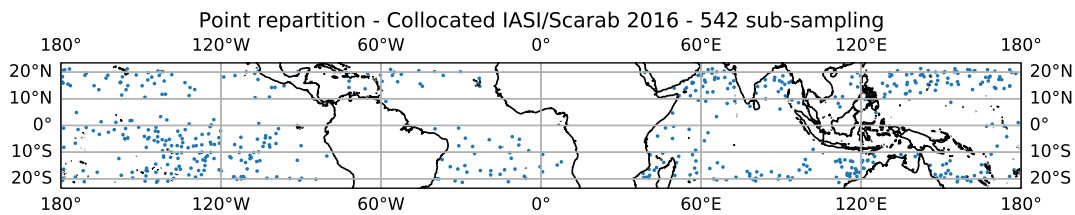
FIGURE 5.12 – Répartition géographique des 542 observations IASI extraites de la base colocalisée IASI/ScaRaB.
