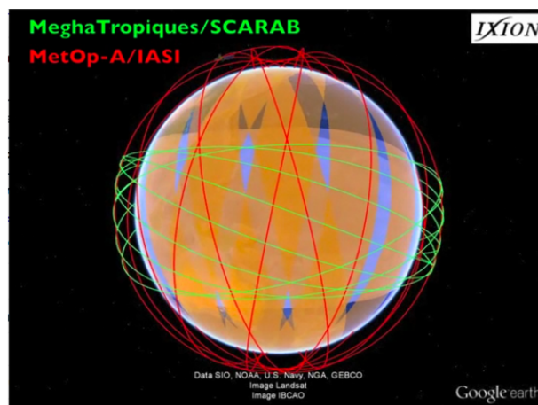
FIGURE 4.10 – Représentation d'orbites suivies par les plateformes Megha-Tropiques embarquant l'instrument ScaRaB (vert) et Metop-A embarquant IASI (rouge). Figure réalisée grâce au logiciel d'orbitographie IXION ( https://climserv.ipsl.polytechnique.fr/ixion/ ).
