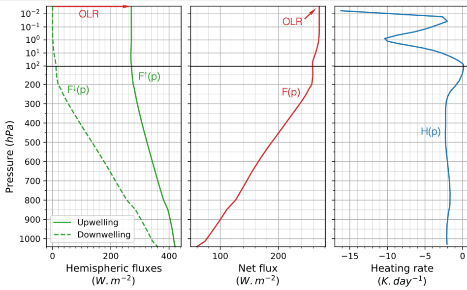
FIGURE 1.4 – Profils de flux radiatifs hémisphériques (gauche), de flux net (centre) et de taux de chauffage (droite) à grande longueur d'onde et en ciel-clair, simulés avec 4A-Flux pour l'atmosphère moyenne tropicale de TIGR 2000.
