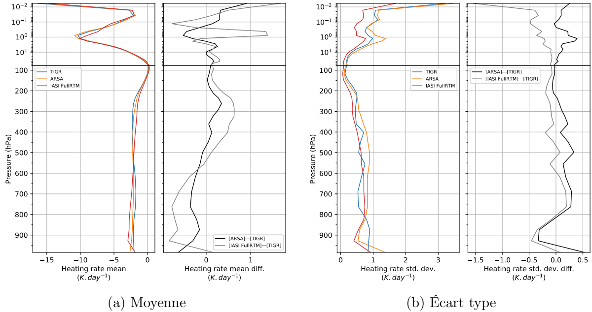
FIGURE 5.14 – Moyennes et écarts types des profils de taux de chauffage simulés par 4A-Flux sur la base d'apprentissage TIGR (bleu), sur la base d'évaluation ARSA (orange) et sur la base colocalisée IASI/ScaRaB (rouge) pour des atmosphères de type tropical et différences entre profils de moyenne et d'écart type par rapport à TIGR (noir et gris).
