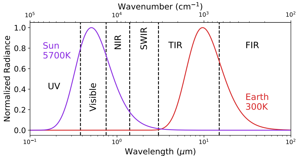
FIGURE 1.2 – Luminance de Planck normalisée pour un corps à la température du Soleil (violet), et à la température de la Terre (rouge). Le spectre de Planck à la température du Soleil couvre une partie du domaine ultraviolet (UV) et les domaines du visible, du proche infrarouge (Near Infrared : NIR) et de l'infrarouge moyen (Shortwave Infrared : SWIR). Le spectre de Planck à la température de la Terre couvre l'infrarouge thermique (Thermal Infrared : TIR) et l'infrarouge lointain (Far Infrared : FIR).
