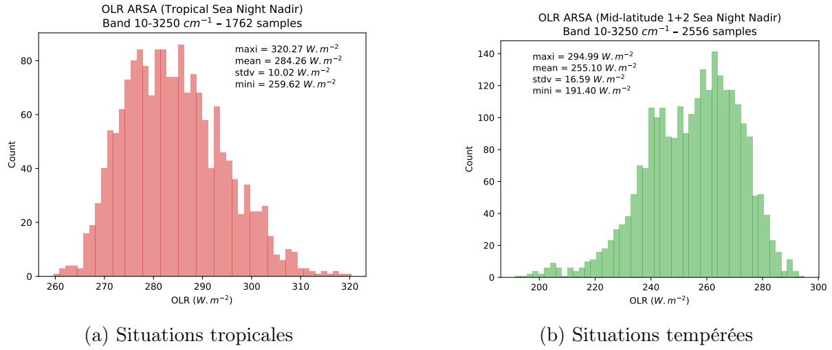
FIGURE 4.9 – Histogrammes des OLR simulés par l’approche avec 4A-Flux à partir de la base ARSA (sous-sélection mer, nuit et nadir) sur la bande spectrale 10 – 3250 \text{cm}^{-1} .
