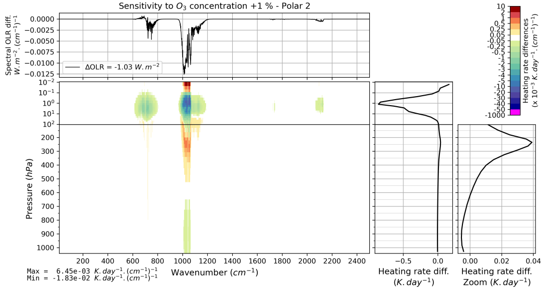
FIGURE B.40 – Effet d'une augmentation verticalement uniforme de 1 % de la concentration d'ozone sur l'OLR et le taux de chauffage vertical pour l'atmosphère moyenne Polar 2 de TIGR 2000.
