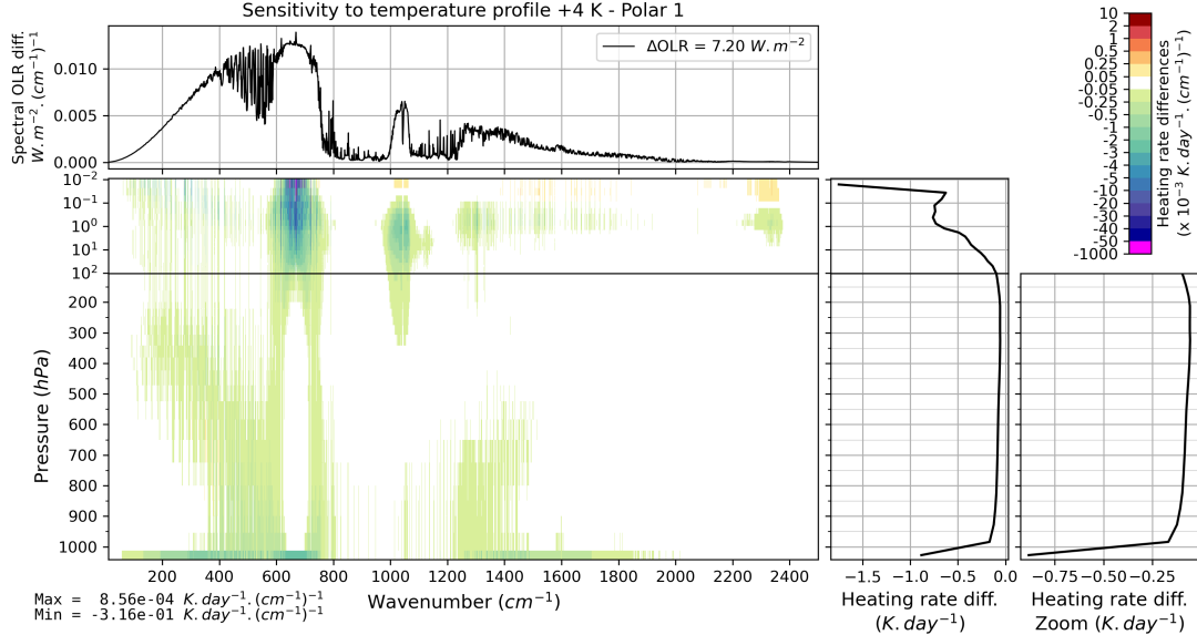
FIGURE B.14 – Effet d’une perturbation uniforme de 4 K de la température de l’atmosphère sur l’OLR et le taux de chauffage vertical pour l’atmosphère moyenne Polar 1 de TIGR 2000.
