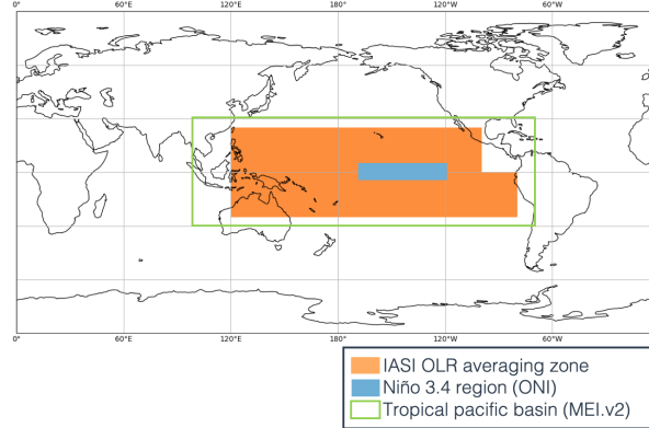
FIGURE 5.4 – Définitions des régions sur lesquelles sont calculés les indices ENSO et de la région sur laquelle est calculée l'anomalie d'OLR pour la comparaison présentée dans cette section.
