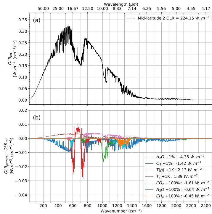
FIGURE B.3 – OLR (a) et sensibilité \Delta OLR_\nu (b) aux différentes perturbations de paramètres atmosphériques et de surface pour l’atmosphère moyenne Mid-latitude 2 de TIGR.
