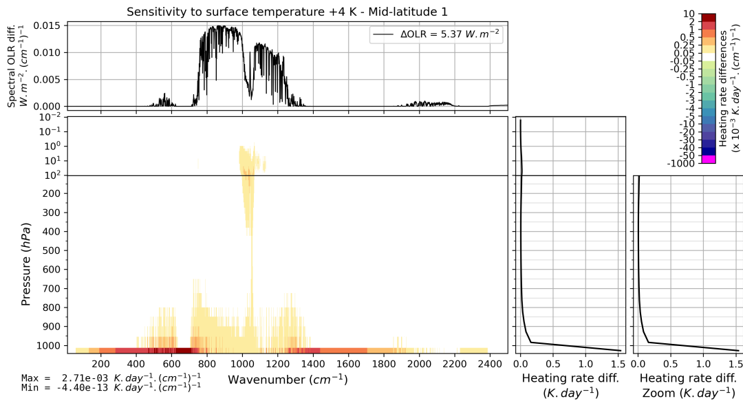
FIGURE B.7 – Effet d’une perturbation de 4 K de la température de surface sur l’OLR et le taux de chauffage vertical pour l’atmosphère moyenne Mid-latitude 1 de TIGR 2000.
