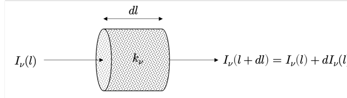
FIGURE 2.3 – Représentation schématique d'une parcelle de gaz de coefficient d'extinction k_\nu et d'épaisseur infinitésimale dl , traversée longitudinalement par un faisceau de luminance spectrale I_\nu(M, \vec{\Omega}) à l'entrée de la parcelle et subissant une extinction de dI_\nu à sa traversée.
