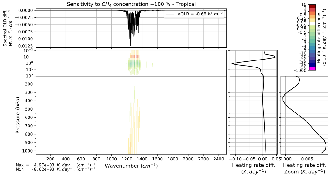
FIGURE B.21 – Effet d'un doublement verticalement uniforme de la concentration de \text{CH}_4 (de 1860 à 3720 ppbv) sur l'OLR et le taux de chauffage vertical pour l'atmosphère moyenne Tropical de TIGR 2000.
