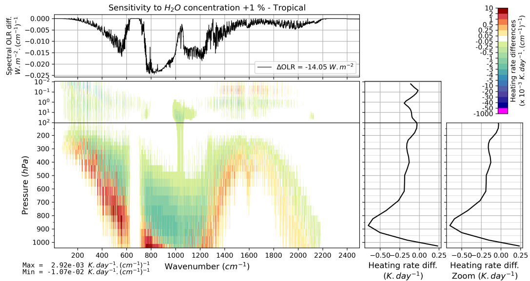
FIGURE B.31 – Effet d'une augmentation verticalement uniforme de 1 % de la concentration de vapeur d'eau sur l'OLR et le taux de chauffage vertical pour l'atmosphère moyenne Tropical de TIGR 2000.
