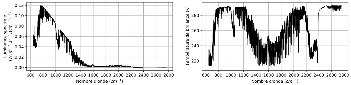
FIGURE 1.7 – Spectre de luminance (gauche) et spectre de température de brillance (droite) IASI simulés par 4A/OP pour l’atmosphère moyenne tropicale de TIGR 2000 a au nadir. L’échantillonnage spectral est 0.25 \text{ cm}^{-1} entre 645 et 2760 \text{ cm}^{-1} , soit 8461 canaux.
