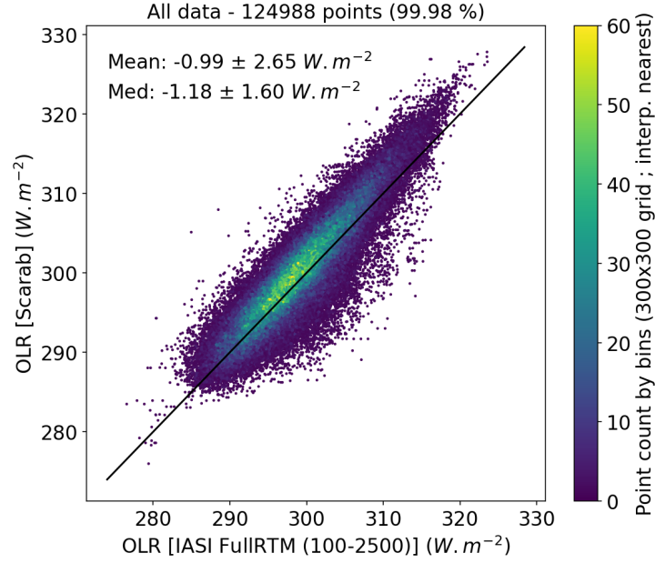
FIGURE 4.20 – Diagramme de dispersion et statistiques de l’OLR IASI avec l’approche FullRTM sur la bande spectrale 100 – 2500 cm -1 (abscisses) comparés à l’OLR mesuré par ScaRaB (ordonnées). Les statistiques sont calculées sur la différence [IASI moins ScaRaB] et les statistiques affichées correspondent à la moyenne et à l’écart type en première ligne et à la médiane et l’écart type robuste en deuxième ligne.
