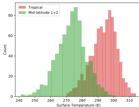
FIGURE 4.4 – Histogrammes des températures de surface de TIGR pour les masses d'air de types tropical (rouge) et tempéré (vert).
