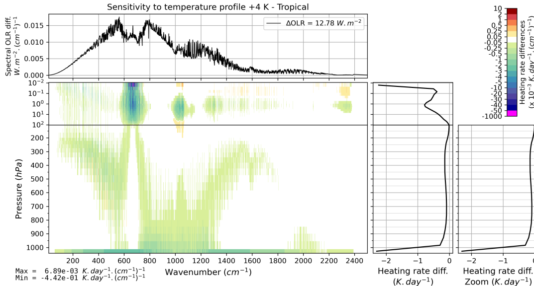
FIGURE B.11 – Effet d’une perturbation uniforme de 4 K de la température de l’atmosphère sur l’OLR et le taux de chauffage vertical pour l’atmosphère moyenne Tropical de TIGR 2000.
