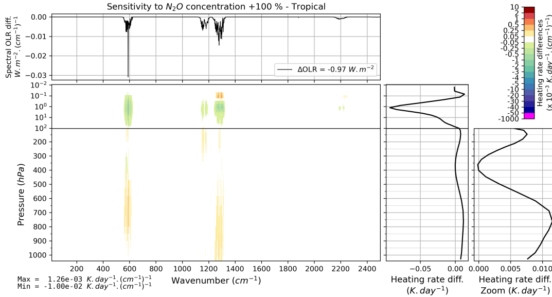
FIGURE B.26 – Effet d'un doublement verticalement uniforme de la concentration de N_2O (de 324 à 648 ppbv) sur l'OLR et le taux de chauffage vertical pour l'atmosphère moyenne Tropical de TIGR 2000.
