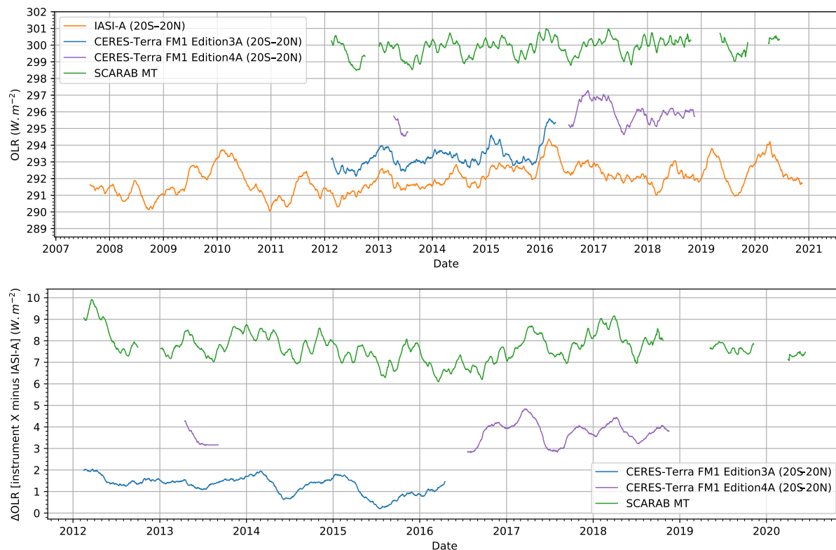
FIGURE 5.3 – En haut : Séries temporelles de la moyenne journalière des OLR (ciel-clair, nuit, océans) entre 20°S-20°N pour les trois instruments IASI, CERES et ScaRaB (données partielles pour CERES et ScaRaB). En bas : différence des séries temporelles [instrument X moins IASI-A]. Un lissage des séries est réalisé sur 90 jours glissants.
