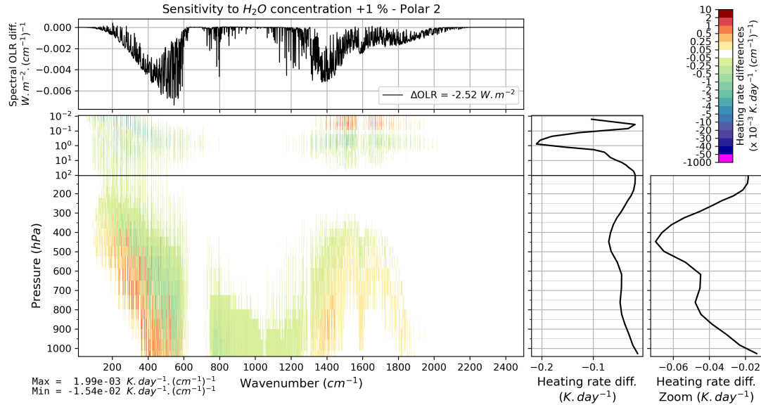
FIGURE B.35 – Effet d’une augmentation verticalement uniforme de 1 % de la concentration de vapeur d’eau sur l’OLR et le taux de chauffage vertical pour l’atmosphère moyenne Polar 2 de TIGR 2000.
