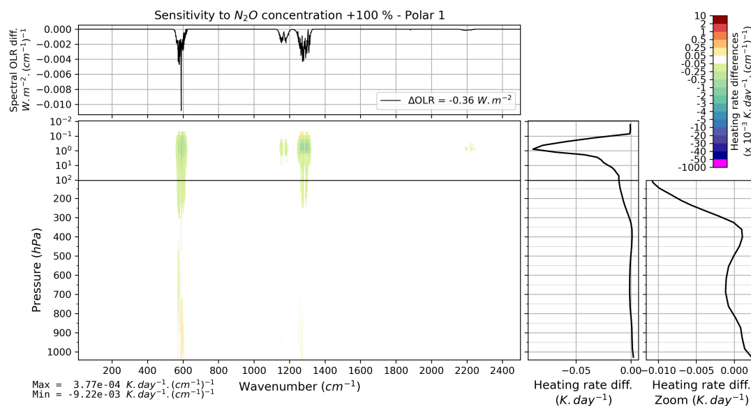
FIGURE B.29 – Effet d'un doublement verticalement uniforme de la concentration de N_2O (de 324 à 648 ppbv) sur l'OLR et le taux de chauffage vertical pour l'atmosphère moyenne Polar 1 de TIGR 2000.
