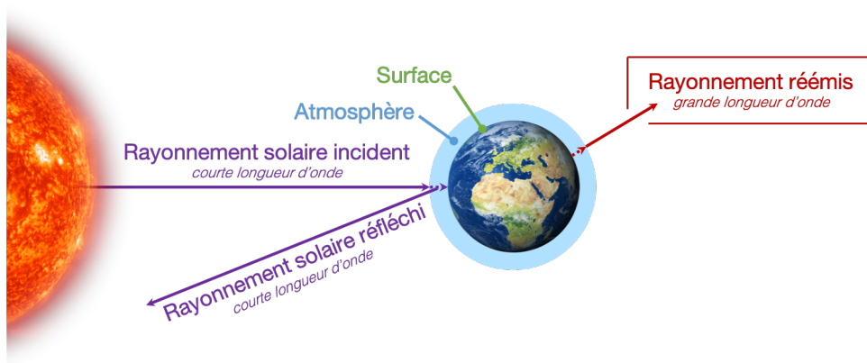
FIGURE 1.1 – Représentation schématique de l'équilibre radiatif du système Terre au sommet de l'atmosphère. Le rayonnement solaire incident et le rayonnement solaire réfléchi définissent le domaine spectral à courte longueur d'onde. Le rayonnement réémis après absorption définit le domaine à grande longueur d'onde.
