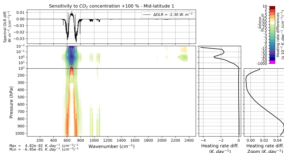
FIGURE B.17 – Effet d'un doublement verticalement uniforme de la concentration de CO 2 (de 395 à 790 ppmv) sur l'OLR et le taux de chauffage vertical pour l'atmosphère moyenne Mid-latitude 1 de TIGR 2000.
