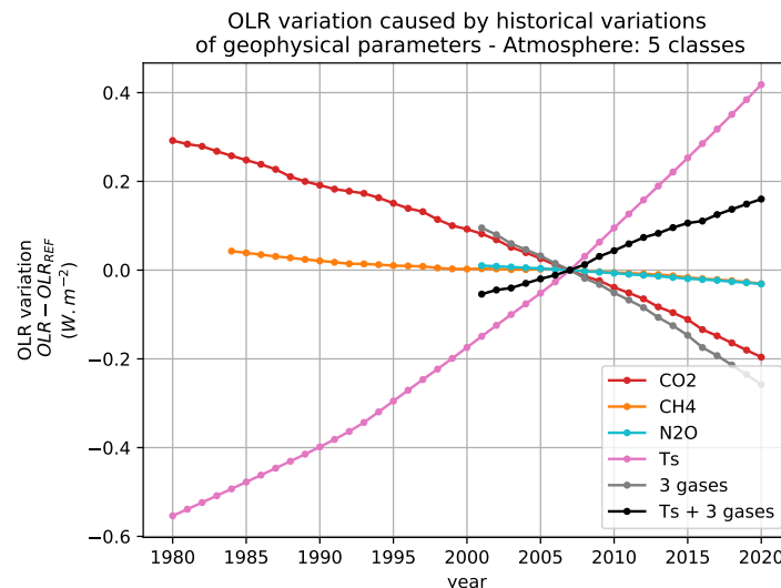
FIGURE 3.13 – Variations de l'OLR par rapport à 2007 estimées à partir des variations historiques récentes de température de surface et des concentrations des gaz à effet de serre (facteurs pris séparément ou en combinaison) en moyenne sur les cinq classes TIGR 2000.
