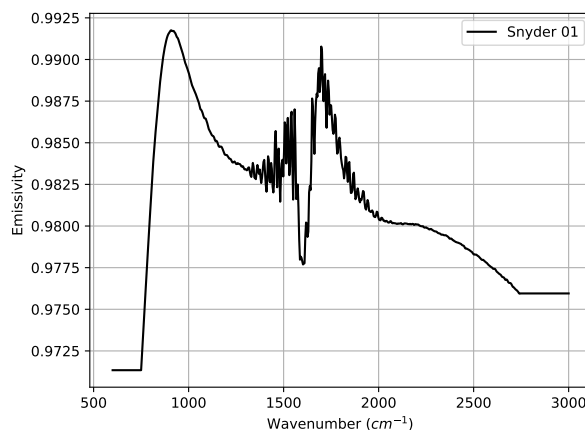
FIGURE 4.12 – Spectre d'émissivité Snyder 1.
