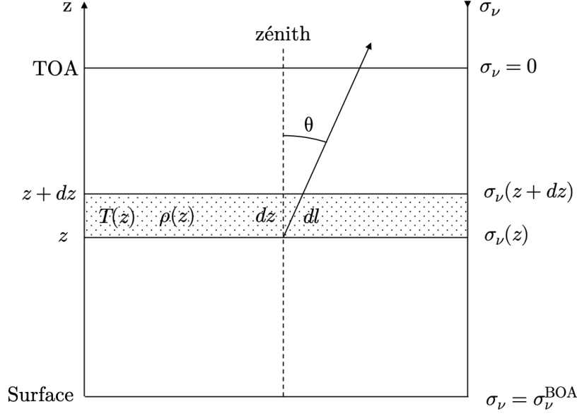
FIGURE 2.4 – Description de la géométrie utilisée : Approximation plan-parallèle
