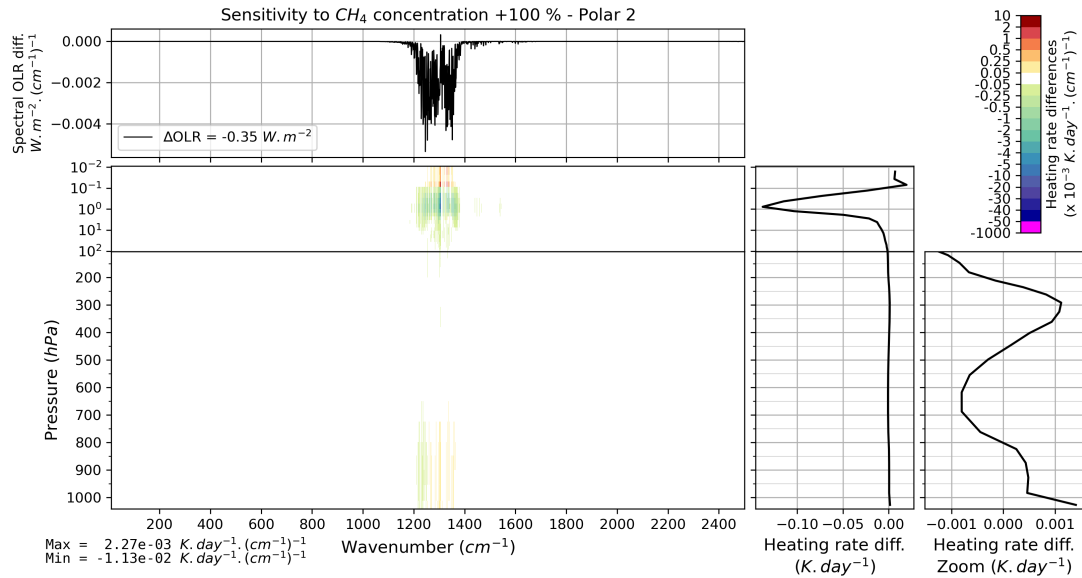
FIGURE B.25 – Effet d'un doublement verticalement uniforme de la concentration de \text{CH}_4 (de 1860 à 3720 ppbv) sur l'OLR et le taux de chauffage vertical pour l'atmosphère moyenne Polar 2 de TIGR 2000.
