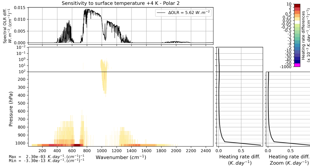
FIGURE B.10 – Effet d’une perturbation de 4 K de la température de surface sur l’OLR et le taux de chauffage vertical pour l’atmosphère moyenne Polar 2 de TIGR 2000.
