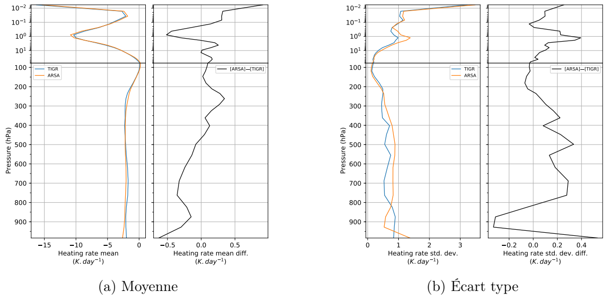
FIGURE 5.10 – Moyennes et écarts types des profils de taux de chauffage simulés par 4A-Flux sur la base d'apprentissage TIGR (bleu) et sur la base d'évaluation ARSA (orange) pour des atmosphères de type tropical et différences entre profils de moyenne et d'écart type (noir).
