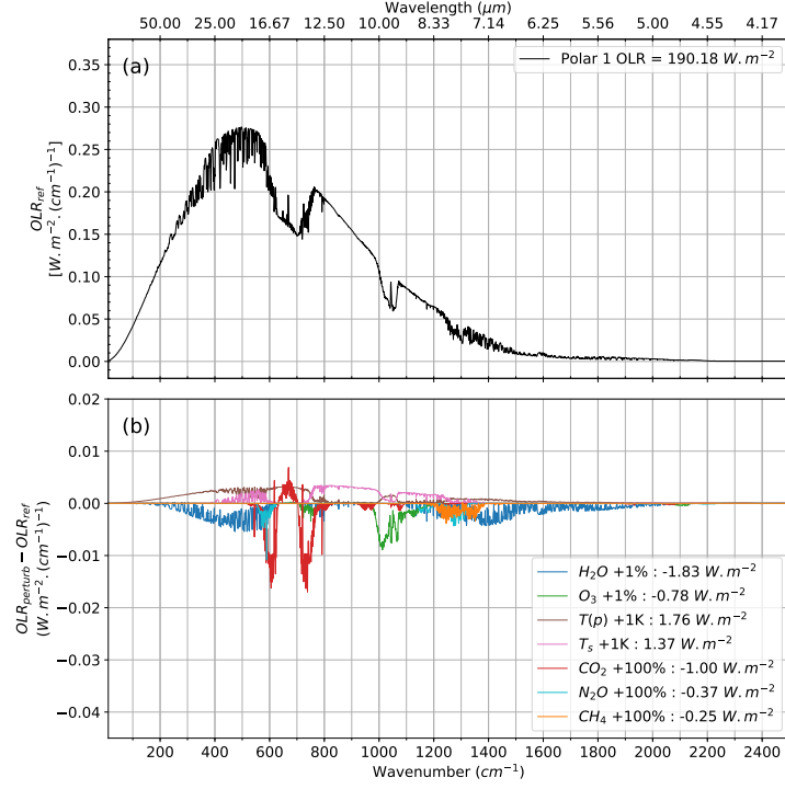
FIGURE B.4 – OLR (a) et sensibilité \Delta OLR_\nu (b) aux différentes perturbations de paramètres atmosphériques et de surface pour l'atmosphère moyenne Polar 1 de TIGR.
