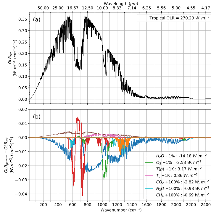
FIGURE B.1 – OLR (a) et sensibilité \Delta OLR_\nu (b) aux différentes perturbations de paramètres atmosphériques et de surface pour l'atmosphère moyenne Tropical de TIGR.
