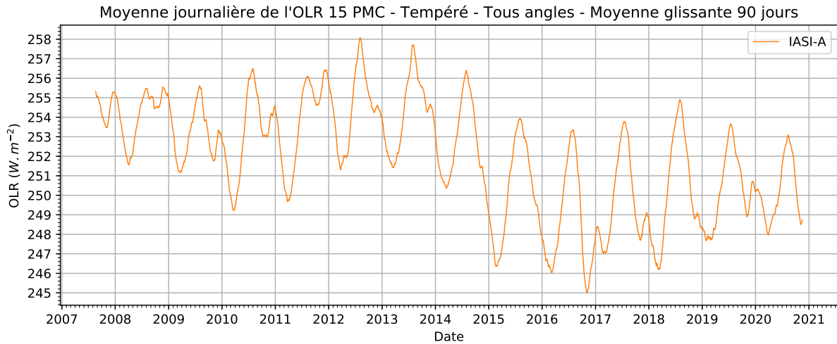
FIGURE 5.1 – Série temporelle de la moyenne journalière des OLR (ciel-clair, nuit, océans) estimés par l'ensemble des PMC en atmosphère de type tempéré uniquement, pour tous les angles de vue de IASI. Un lissage de la série est réalisé sur 90 jours glissants.
