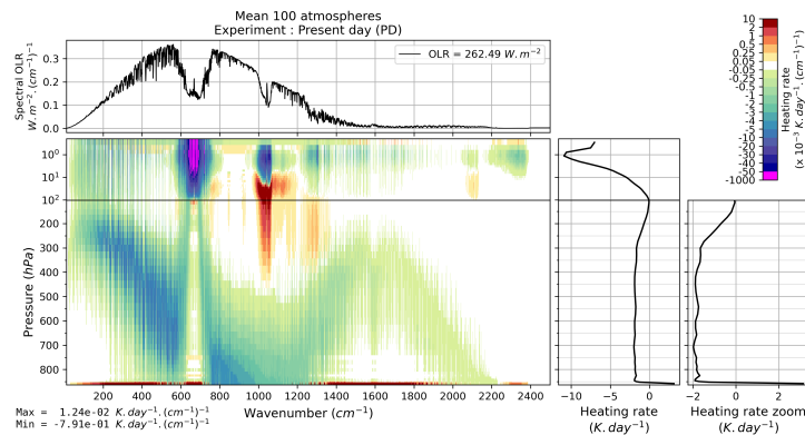
FIGURE 3.9 – OLR et taux de chauffage moyennés sur les 100 atmosphères RFMIP pour le scénario Present day (option de forçage f1).
