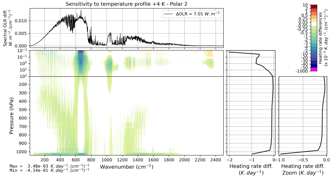
FIGURE B.15 – Effet d’une perturbation uniforme de 4 K de la température de l’atmosphère sur l’OLR et le taux de chauffage vertical pour l’atmosphère moyenne Polar 2 de TIGR 2000.
