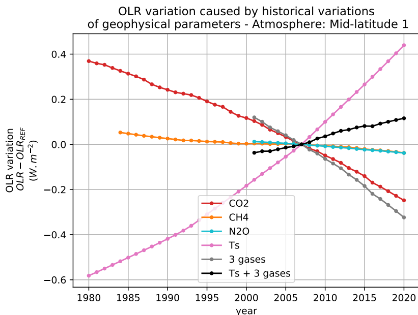
FIGURE B.42 – Variations de l'OLR par rapport à 2007 estimées à partir des variations historiques de température de surface et des concentrations des gaz à effet de serre (pris individuellement ou combinés) pour l'atmosphère moyenne Mid-latitude 1 de TIGR 2000
