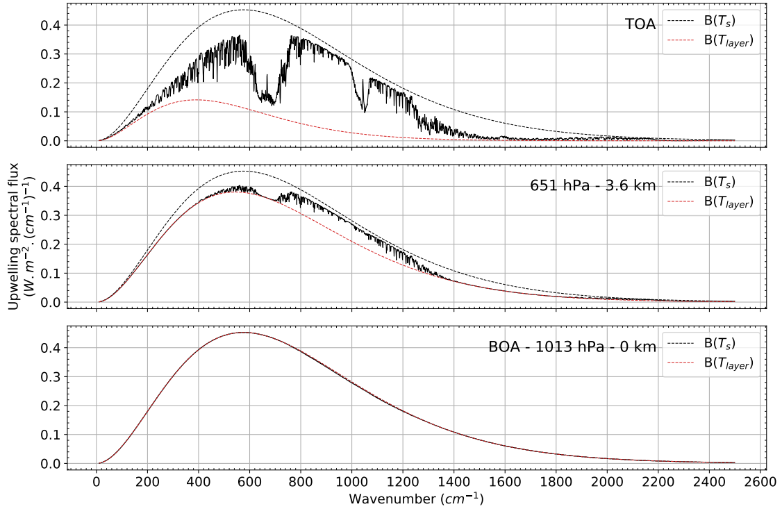
FIGURE 2.1 – Flux monochromatiques montants en ciel clair simulés à la résolution spectrale de 1 \text{ cm}^{-1} (trait plein) à la surface BOA (bas), à environ 3.6 km (milieu) et au sommet de l’atmosphère TOA (haut). Flux émis par un corps noir évalué à la température de surface B(T_s) (trait pointillé noir) et flux émis par un corps noir évalué à la température de l’atmosphère B(T_{layer}) à la surface BOA (bas), à environ 3.6 km (milieu) et au sommet de l’atmosphère TOA (haut). Les simulations ont été réalisées à partir de 4A-Flux (cf. section 2.3) pour une atmosphère de type tropical (TIGR 2000 - mean tropical class).
