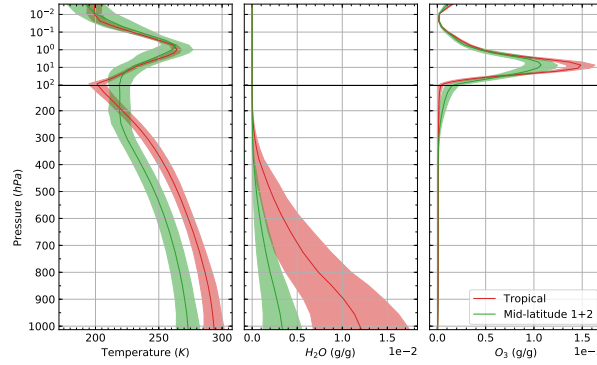
FIGURE 4.5 – Profils atmosphériques TIGR moyens (courbe pleine) et plage \pm 1 écart type (zones colorées) pour les masses d’air de types tropical (rouge) et tempéré (vert). Le profil de température se trouve à gauche, au centre se trouve le profil de concentration de vapeur d’eau et à droite le profil de concentration d’ozone.
