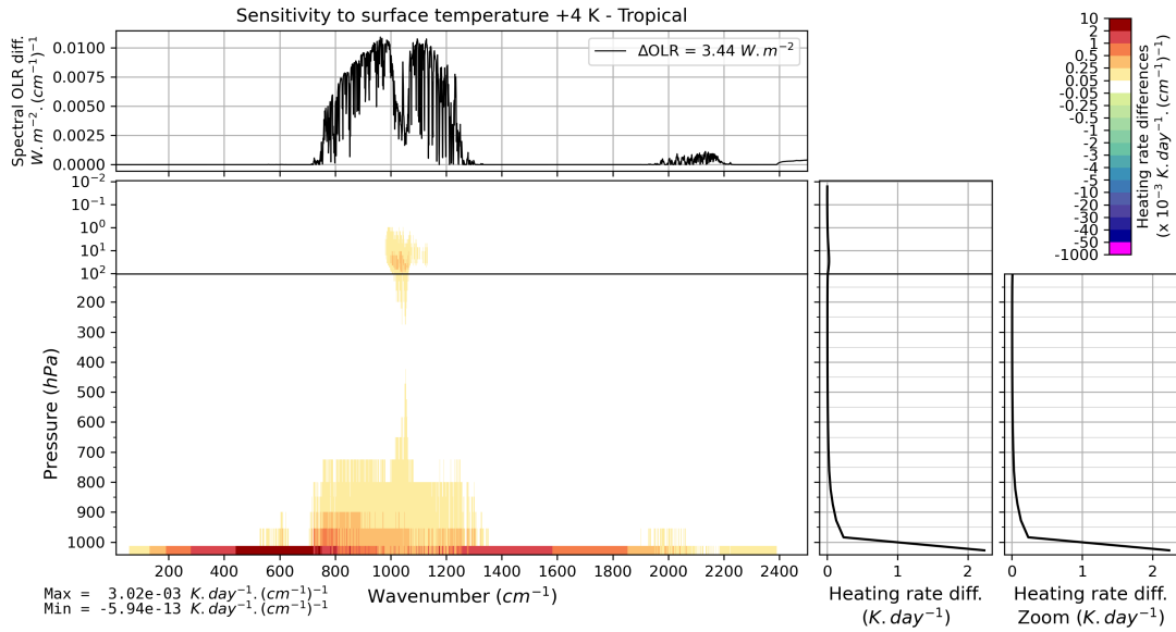
FIGURE B.6 – Effet d’une perturbation de 4 K de la température de surface sur l’OLR et le taux de chauffage vertical pour l’atmosphère moyenne Tropical de TIGR 2000.
