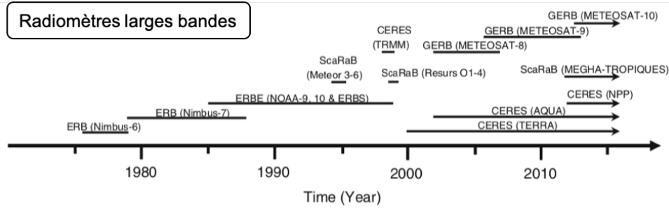
FIGURE 1.5 – Exemples de radiomètres larges bandes dédiés à la mesure de l’OLR et du RSW. Les plateformes sur lesquelles les instruments sont embarqués sont indiquées entre parenthèses et les flèches indiquent les missions toujours actives en 2016. Figure adaptée de BRINDLEY et BANTGES 2016.
