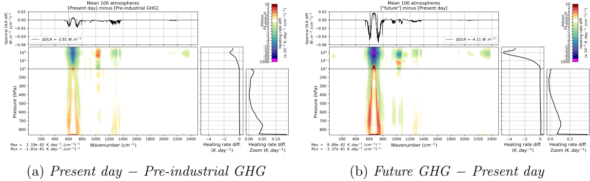
FIGURE 3.10 – Variation moyenne d’OLR et de taux de chauffage vertical sur la base RFMIP entre le scénario Pre-industrial GHG et le scénario Present day et entre le scénario Present day et le scénario Future GHG .
