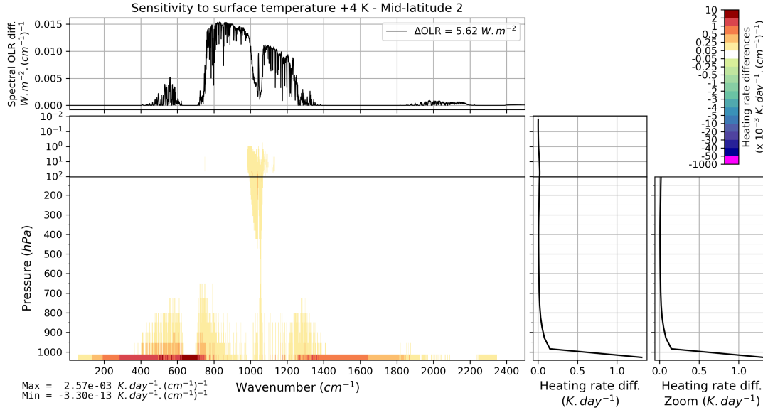
FIGURE B.8 – Effet d’une perturbation de 4 K de la température de surface sur l’OLR et le taux de chauffage vertical pour l’atmosphère moyenne Mid-latitude 2 de TIGR 2000.
