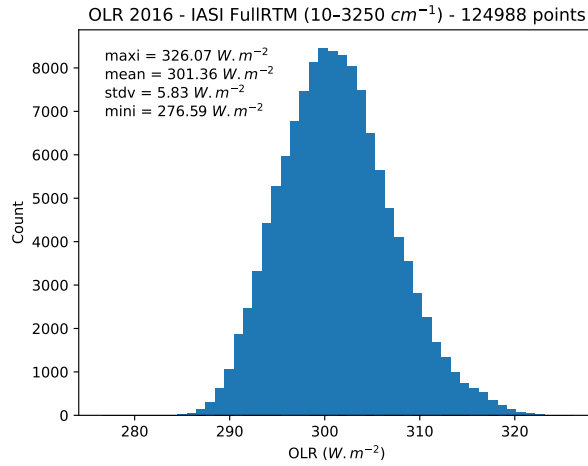
FIGURE 4.15 – Histogrammes des OLR simulés par l'approche FullRTM à partir de la base de mesures colocalisées IASI/ScaRaB 2016, sur la bande spectrale 10-3250 \text{cm}^{-1} .
