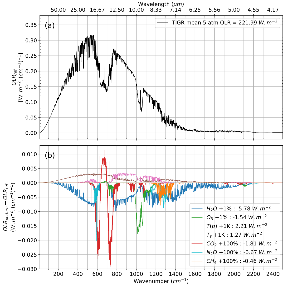
FIGURE 3.3 – OLR (a) et sensibilité \Delta OLR_\nu (b) aux différentes perturbations de paramètres atmosphériques et de surface pour la moyenne des cinq atmosphères moyennes de TIGR.
