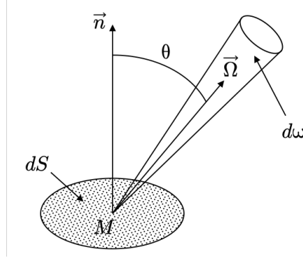
FIGURE 2.2 – Énergie radiative transportée par un faisceau de rayonnement électromagnétique dans la direction \vec{\Omega} , sous l'angle solide élémentaire d\omega à travers une surface transparente d'aire élémentaire dS et de normale \vec{n} orientée d'un angle \theta par rapport à la direction de propagation ( \cos \theta = \vec{n} \cdot \vec{\Omega} ).
