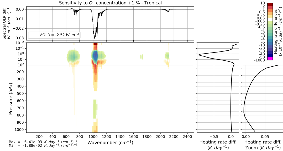
FIGURE B.36 – Effet d’une augmentation verticalement uniforme de 1 % de la concentration d’ozone sur l’OLR et le taux de chauffage vertical pour l’atmosphère moyenne Tropical de TIGR 2000.
