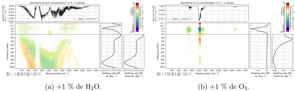
FIGURE 3.7 – Effet d'une augmentation verticalement uniforme de 1 % de la concentration de vapeur d'eau et d'ozone sur l'OLR moyen et le taux de chauffage vertical moyen des 5 classes TIGR 2000.
