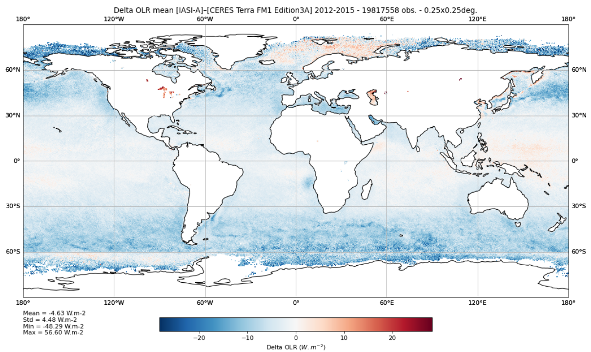
FIGURE 5.8 – Différence entre l'OLR moyen IASI-A estimé avec l'ensemble de 30 PMC (figure 5.7a) et l'OLR moyen mesuré par CERES Terra (FM1/Edition3A) (figure 5.7b) sur la période 2012-2015 sur une grille de 0.25° par 0.25°
