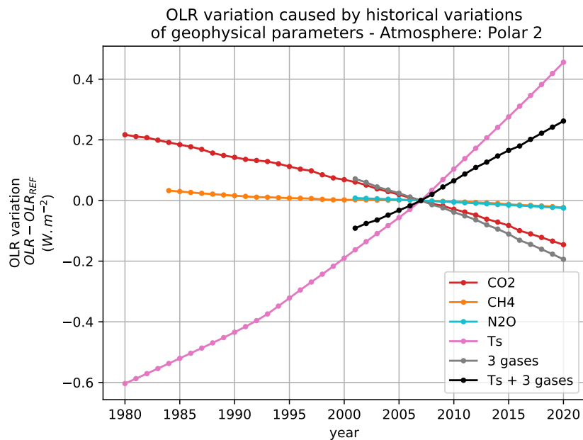
FIGURE B.45 – Variations de l'OLR par rapport à 2007 estimées à partir des variations historiques de température de surface et des concentrations des gaz à effet de serre (pris individuellement ou combinés) pour l'atmosphère moyenne Polar 2 de TIGR 2000
