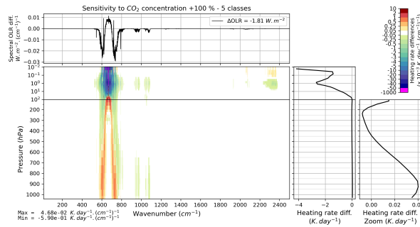
FIGURE 3.5 – Effet d'un doublement verticalement uniforme de la concentration de \text{CO}_2 (de 395 à 790 ppmv) sur l'OLR moyen et le taux de chauffage vertical moyen des 5 classes TIGR 2000.
