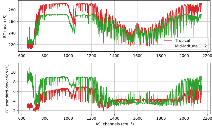
FIGURE 4.6 – Moyenne et écart type des spectres de température de brillance IASI simulés en visée au nadir sur la base TIGR pour les types de masses d'air tropicales (rouge) et tempérées (vert).
