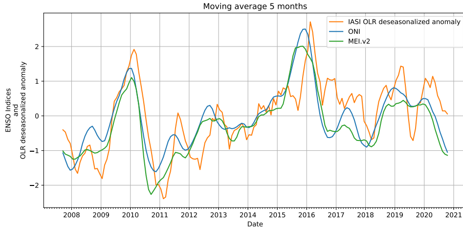
FIGURE 5.5 – Comparaison de la série temporelle de l’anomalie d’OLR tropical désaisonnalisée IASI-A et des séries d’indice de suivi du phénomène ENSO que sont ONI (Oceanic Niño Index) et MEI.v2 (Multivariate ENSO Index version 2). Un lissage de la série est réalisé sur 150 jours glissants.
