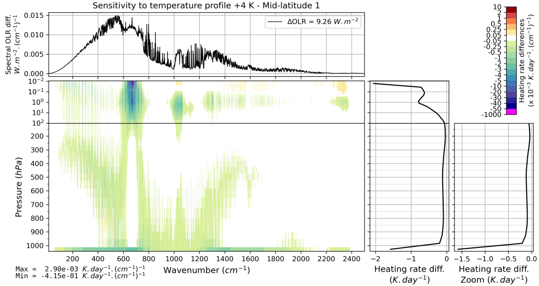
FIGURE B.12 – Effet d’une perturbation uniforme de 4 K de la température de l’atmosphère sur l’OLR et le taux de chauffage vertical pour l’atmosphère moyenne Mid-latitude 1 de TIGR 2000.
