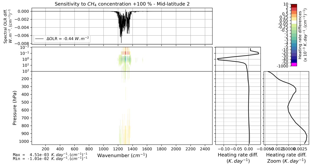
FIGURE B.23 – Effet d'un doublement verticalement uniforme de la concentration de CH_4 (de 1860 à 3720 ppbv) sur l'OLR et le taux de chauffage vertical pour l'atmosphère moyenne Mid-latitude 2 de TIGR 2000.
