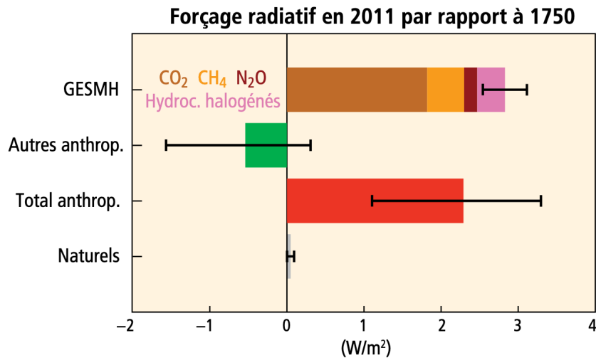
FIGURE 1.3 – Forçage radiatif des changements climatiques pendant l'ère industrielle (1750–2011). Les barres indiquent le forçage provoqué par les gaz à effet de serre au mélange homogène (GESMH), les autres forçages anthropiques, le total des forçages anthropiques et les forçages naturels. Les marges d'erreur indiquent l'incertitude à 5–95 %. Les autres forçages anthropiques comprennent les effets des changements survenus au niveau des aérosols, de l'ozone et de l'albédo lié à l'utilisation des terres. Les forçages naturels englobent les effets de l'activité solaire et de l'activité volcanique. (PACHAURI et MAYER 2015, figure 1.4, p. 45)
