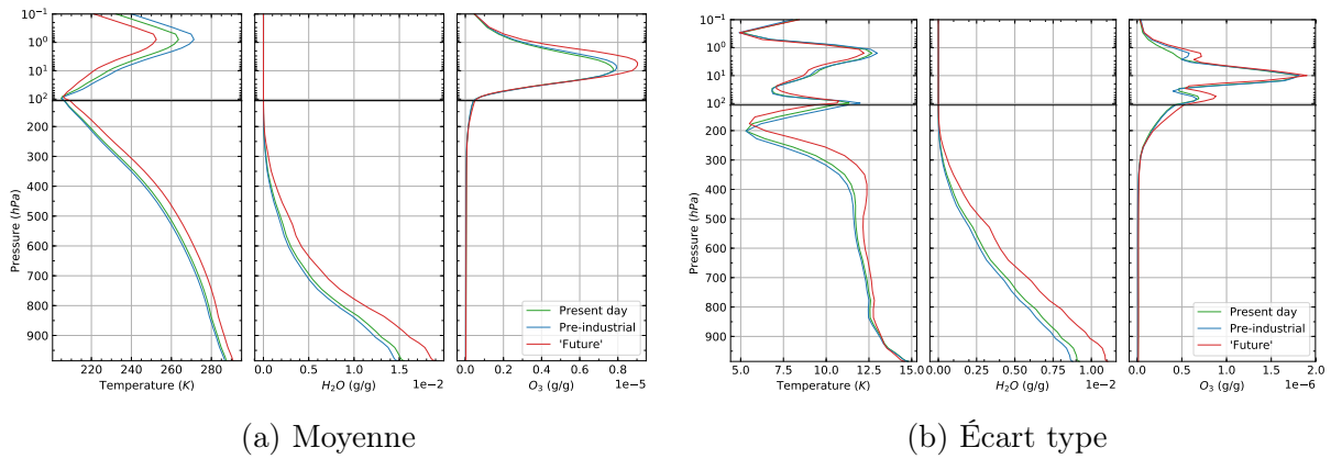
FIGURE 3.8 – Statistiques pondérées des 100 profils de température, de concentration de vapeur d'eau et de concentration d'ozone de la base de données RFMIP pour les scénarios préindustriel, présent et futur.
