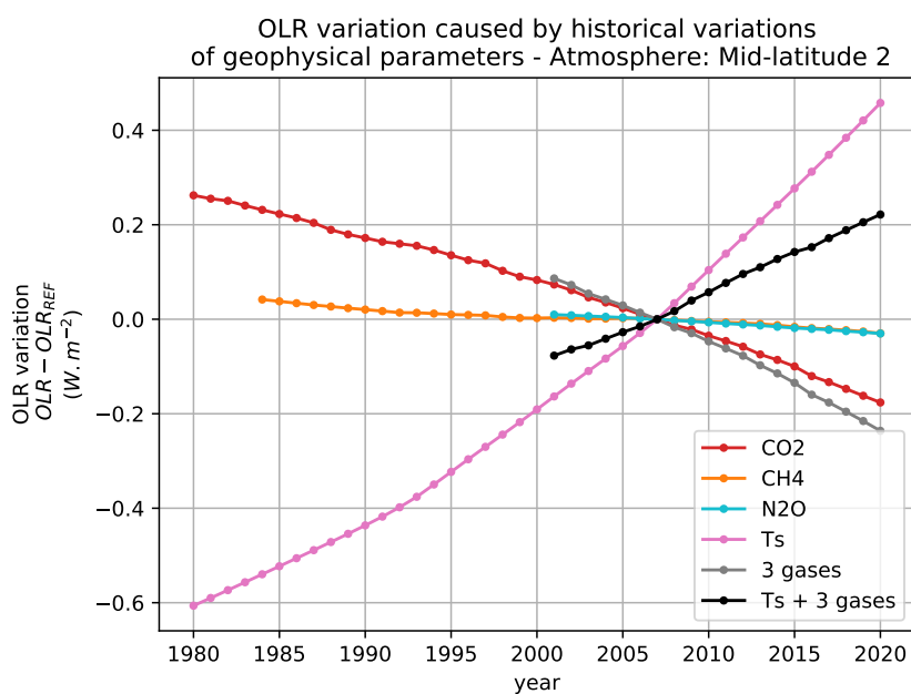
FIGURE B.43 – Variations de l'OLR par rapport à 2007 estimées à partir des variations historiques de température de surface et des concentrations des gaz à effet de serre (pris individuellement ou combinés) pour l'atmosphère moyenne Mid-latitude 2 de TIGR 2000
