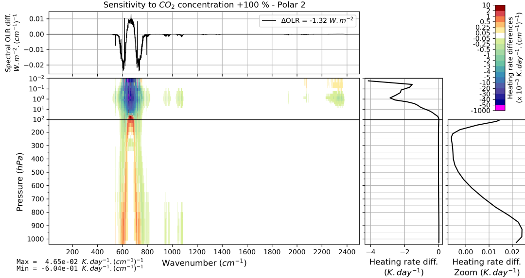
FIGURE B.20 – Effet d'un doublement verticalement uniforme de la concentration de \text{CO}_2 (de 395 à 790 ppmv) sur l'OLR et le taux de chauffage vertical pour l'atmosphère moyenne Polar 2 de TIGR 2000.
