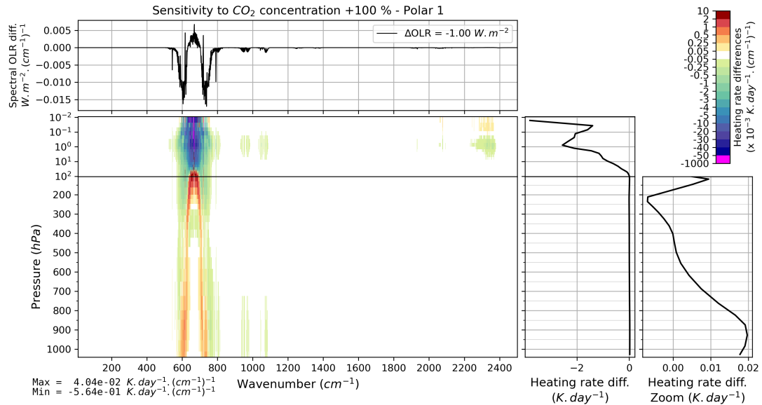
FIGURE B.19 – Effet d'un doublement verticalement uniforme de la concentration de CO 2 (de 395 à 790 ppmv) sur l'OLR et le taux de chauffage vertical pour l'atmosphère moyenne Polar 1 de TIGR 2000.
