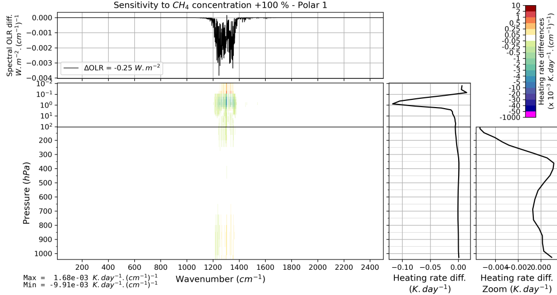
FIGURE B.24 – Effet d'un doublement verticalement uniforme de la concentration de \text{CH}_4 (de 1860 à 3720 ppbv) sur l'OLR et le taux de chauffage vertical pour l'atmosphère moyenne Polar 1 de TIGR 2000.
