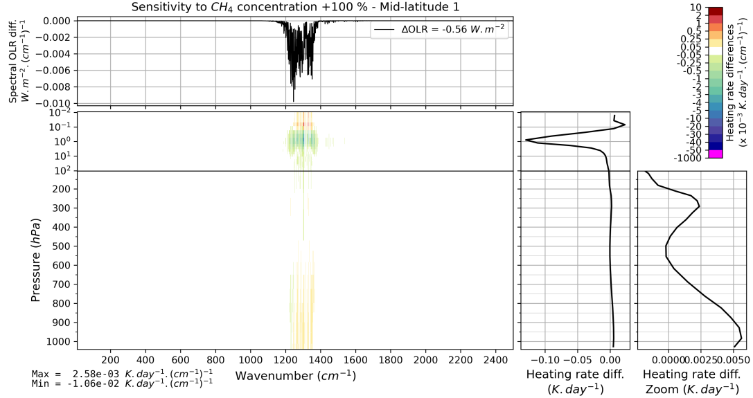
FIGURE B.22 – Effet d'un doublement verticalement uniforme de la concentration de CH_4 (de 1860 à 3720 ppbv) sur l'OLR et le taux de chauffage vertical pour l'atmosphère moyenne Mid-latitude 1 de TIGR 2000.
