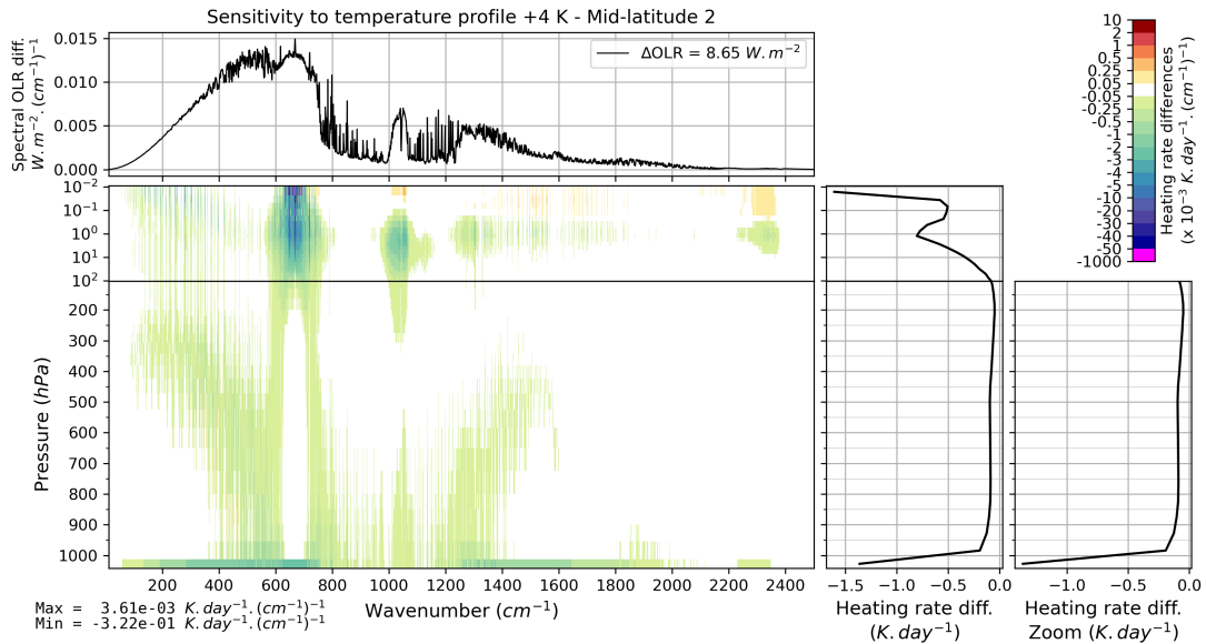
FIGURE B.13 – Effet d’une perturbation uniforme de 4 K de la température de l’atmosphère sur l’OLR et le taux de chauffage vertical pour l’atmosphère moyenne Mid-latitude 2 de TIGR 2000.
