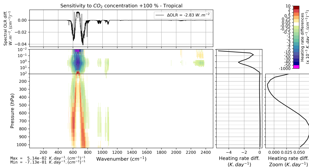
FIGURE B.16 – Effet d'un doublement verticalement uniforme de la concentration de CO 2 (de 395 à 790 ppmv) sur l'OLR et le taux de chauffage vertical pour l'atmosphère moyenne Tropical de TIGR 2000.
