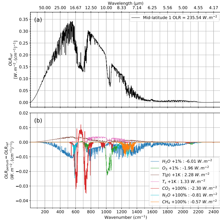
FIGURE B.2 – OLR (a) et sensibilité \Delta OLR_\nu (b) aux différentes perturbations de paramètres atmosphériques et de surface pour l’atmosphère moyenne Mid-latitude 1 de TIGR.
