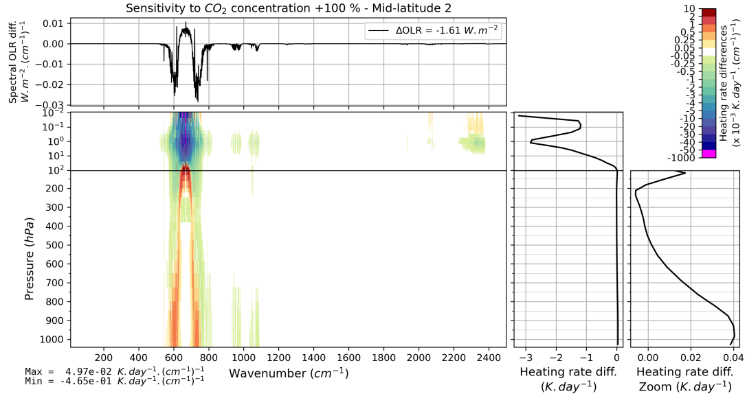
FIGURE B.18 – Effet d'un doublement verticalement uniforme de la concentration de CO 2 (de 395 à 790 ppmv) sur l'OLR et le taux de chauffage vertical pour l'atmosphère moyenne Mid-latitude 2 de TIGR 2000.
