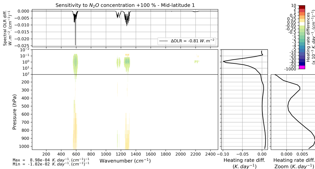
FIGURE B.27 – Effet d'un doublement verticalement uniforme de la concentration de N_2O (de 324 à 648 ppbv) sur l'OLR et le taux de chauffage vertical pour l'atmosphère moyenne Mid-latitude 1 de TIGR 2000.
