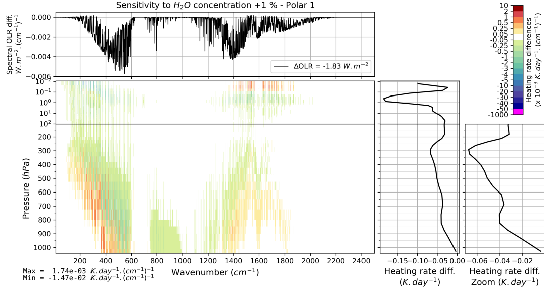
FIGURE B.34 – Effet d’une augmentation verticalement uniforme de 1 % de la concentration de vapeur d’eau sur l’OLR et le taux de chauffage vertical pour l’atmosphère moyenne Polar 1 de TIGR 2000.
