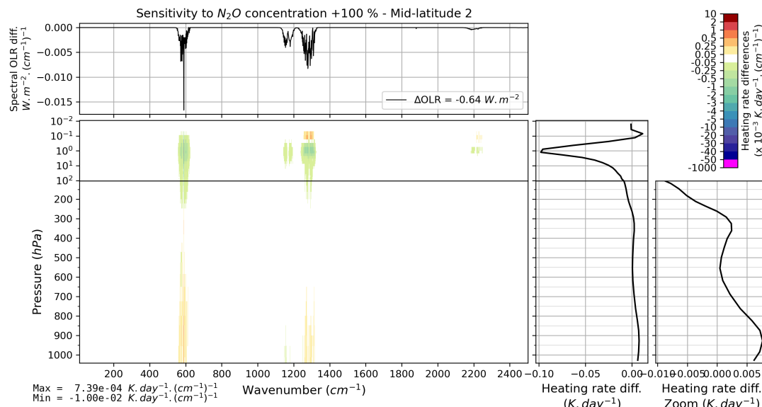
FIGURE B.28 – Effet d'un doublement verticalement uniforme de la concentration de N_2O (de 324 à 648 ppbv) sur l'OLR et le taux de chauffage vertical pour l'atmosphère moyenne Mid-latitude 2 de TIGR 2000.
