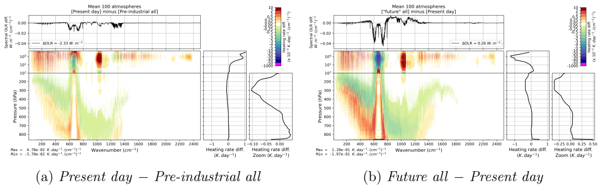
FIGURE 3.11 – Variation moyenne d'OLR et de taux de chauffage vertical sur la base RFMIP entre le scénario Pre-industrial all et le scénario Present day et entre le scénario Present day et le scénario Future all .
