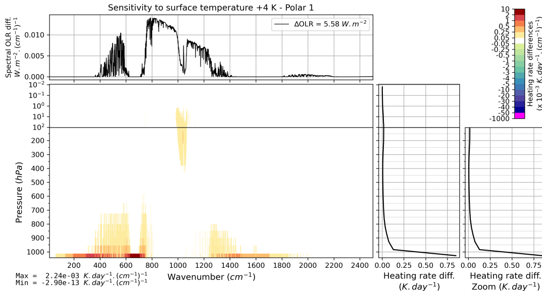
FIGURE B.9 – Effet d’une perturbation de 4 K de la température de surface sur l’OLR et le taux de chauffage vertical pour l’atmosphère moyenne Polar 1 de TIGR 2000.
