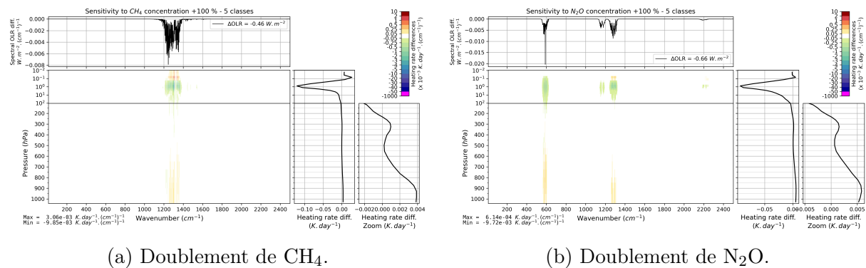
FIGURE 3.6 – Effet d'un doublement verticalement uniforme de la concentration de \text{CH}_4 (de 1860 à 3720 ppbv) et de \text{N}_2\text{O} (de 324 à 648 ppbv) sur l'OLR moyen et le taux de chauffage vertical moyen des 5 classes TIGR 2000.
