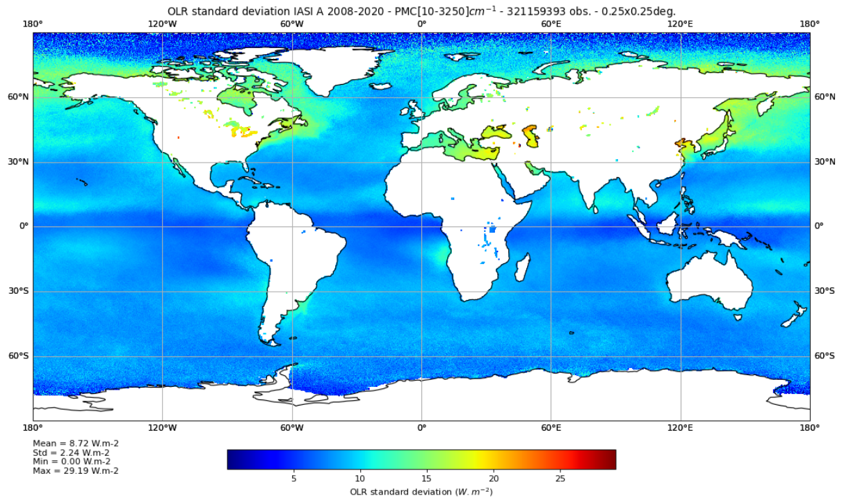
(b) Écart type d'OLR IASI-A
