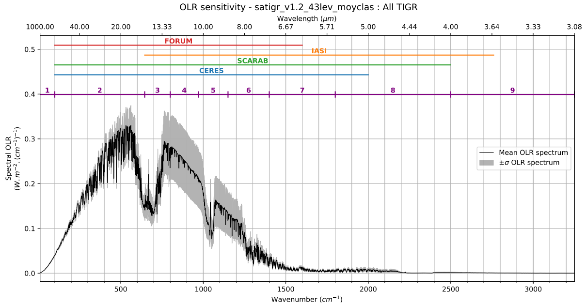
FIGURE 3.1 – Moyenne des spectres d’OLR simulés par 4A-Flux, à la résolution spectrale de 1 \text{ cm}^{-1} , pour les 2311 atmosphères de la base TIGR 2000 toutes classes confondues. La zone grisée correspond à la plage [moyenne \pm écart type] et les bandes horizontales représentent les bandes de sensibilité spectrale de CERES, ScaRaB, IASI et FORUM, ainsi que la segmentation en neuf bandes représentatives de zones spectrales d’intérêt.
