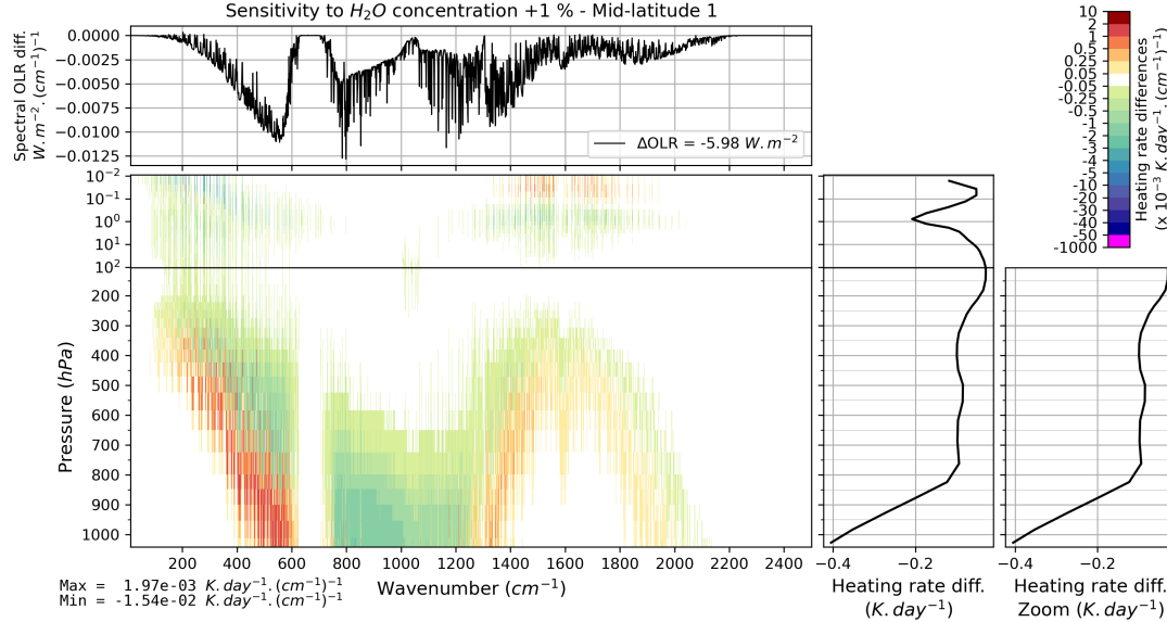
FIGURE B.32 – Effet d’une augmentation verticalement uniforme de 1 % de la concentration de vapeur d’eau sur l’OLR et le taux de chauffage vertical pour l’atmosphère moyenne Mid-latitude 1 de TIGR 2000.
