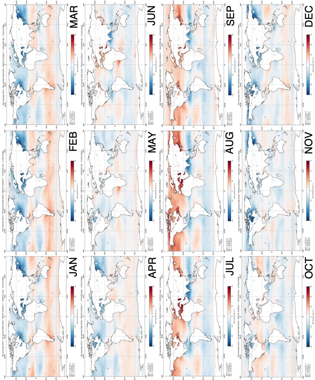
FIGURE 5.9 – Anomalies mensuelles de l'OLR IASI-A par rapport à la moyenne annuelle. Ces anomalies sont calculées sur toute la période 2008-2020. L'échelle de couleur s'étend de -30 à 30 W m^{-2} .
