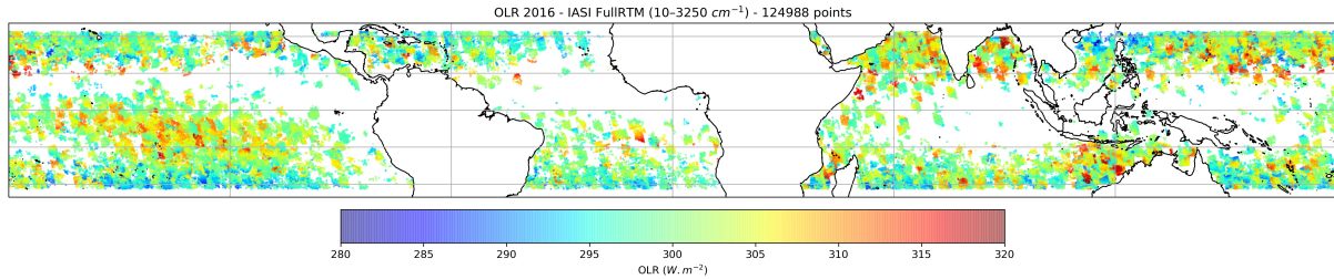
FIGURE 4.16 – Cartes de l'OLR IASI-A intégré sur la bande spectrale LW (10–3250 \text{cm}^{-1} ) estimé par l'approche FullRTM à partir de la base de mesures colocalisées IASI/ScaRaB 2016. La valeur de l'OLR est représentée par l'échelle de couleur.
