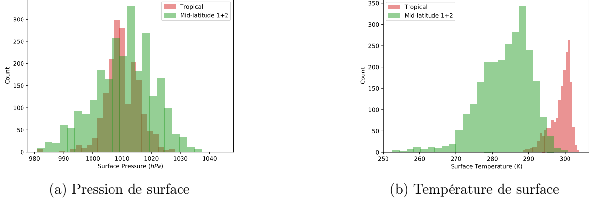
FIGURE 4.8 – Histogrammes des paramètres de surface des bases d’évaluation ARSA du PMC pour les types de masses d’air Tropical et Mid-latitude 1 et 2 en condition nadir, sur mer et de nuit.
