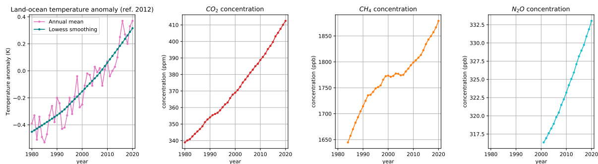
FIGURE 3.12 – Variations historiques récentes de quatre paramètres atmosphériques. De gauche à droite sont présentées : l'anomalie de température globale sur mer et sur terre par rapport à 2012 en moyenne annuelle avec un lissage lowess (source : NASA/GISS) et les moyennes annuelles maritimes des concentrations de \text{CO}_2 , \text{CH}_4 et \text{N}_2\text{O} (source : NOAA/GML).
