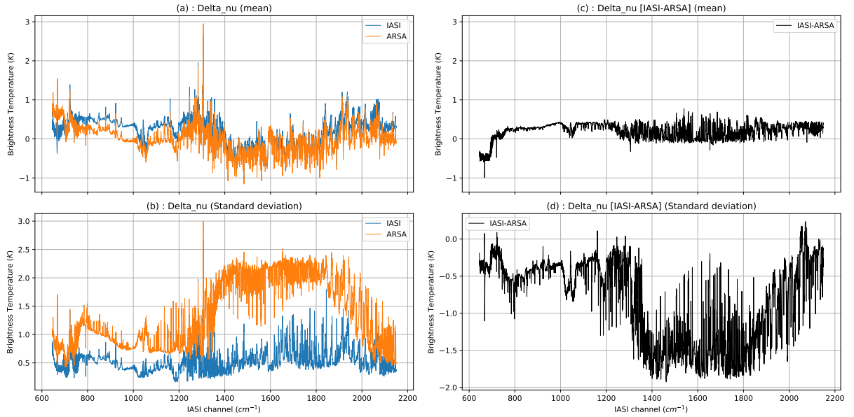
FIGURE 4.19 – Prétraitement deltac des canaux de température de brillance observés sur les bases IASI/ScaRaB 2016 et ARSA. Cadran (a) : valeurs de \Delta_{RTM,\nu}^{IASI} en bleu et \Delta_{RTM,\nu}^{ARSA} en orange. Cadran (b) : Écart type obtenu sur les bases IASI (en bleu) et ARSA (en orange). Cadran (c) : différence [\Delta_{RTM,\nu}^{IASI} - \Delta_{RTM,\nu}^{ARSA}] . Cadran (d) : différence entre les écarts types (IASI-ARSA).
