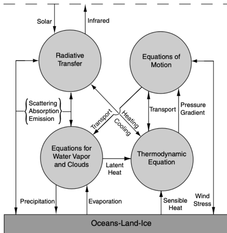
FIGURE 2.5 – Principales composantes et interactions physiques et mathématiques d'un modèle de circulation générale pour les simulations climatiques (extrait de LIOU 2002, p. 504)
