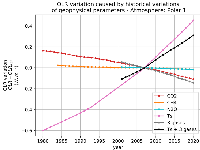
FIGURE B.44 – Variations de l'OLR par rapport à 2007 estimées à partir des variations historiques de température de surface et des concentrations des gaz à effet de serre (pris individuellement ou combinés) pour l'atmosphère moyenne Polar 1 de TIGR 2000
