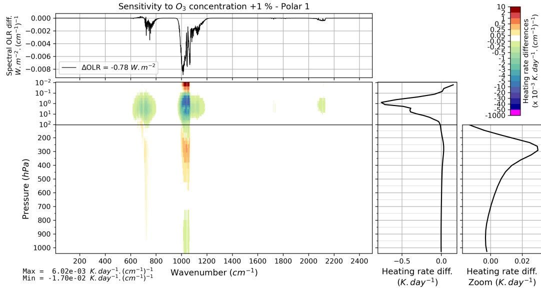
FIGURE B.39 – Effet d’une augmentation verticalement uniforme de 1 % de la concentration d’ozone sur l’OLR et le taux de chauffage vertical pour l’atmosphère moyenne Polar 1 de TIGR 2000.
