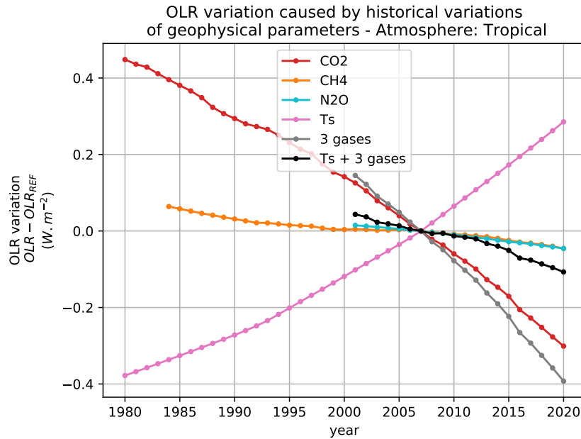
FIGURE B.41 – Variations de l'OLR par rapport à 2007 estimées à partir des variations historiques de température de surface et des concentrations des gaz à effet de serre (pris individuellement ou combinés) pour l'atmosphère moyenne Tropical de TIGR 2000
