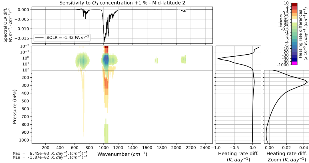
FIGURE B.38 – Effet d’une augmentation verticalement uniforme de 1 % de la concentration d’ozone sur l’OLR et le taux de chauffage vertical pour l’atmosphère moyenne Mid-latitude 2 de TIGR 2000.
