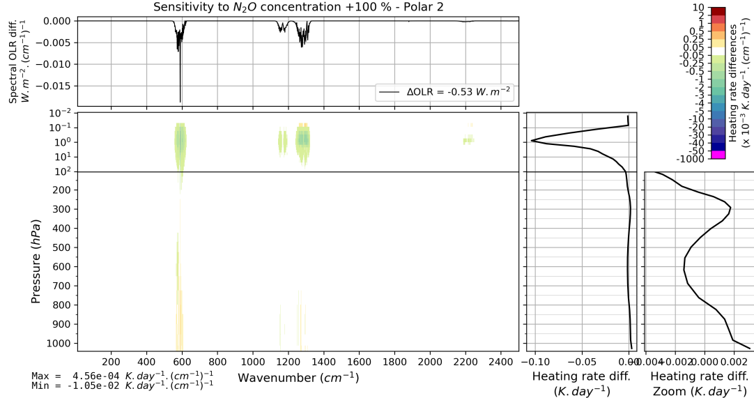
FIGURE B.30 – Effet d'un doublement verticalement uniforme de la concentration de N_2O (de 324 à 648 ppbv) sur l'OLR et le taux de chauffage vertical pour l'atmosphère moyenne Polar 2 de TIGR 2000.
