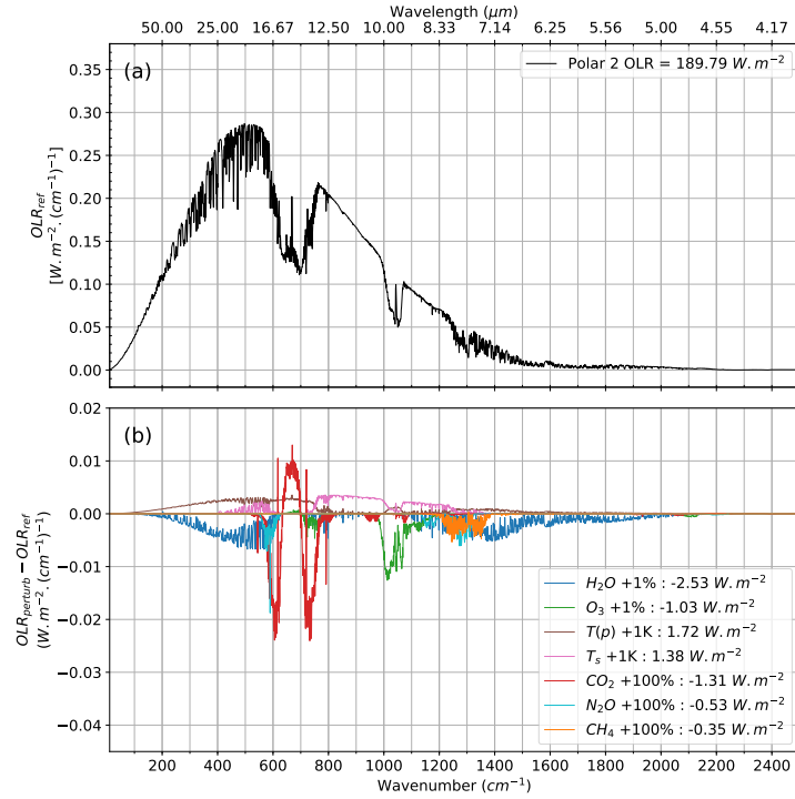
FIGURE B.5 – OLR (a) et sensibilité \Delta OLR_\nu (b) aux différentes perturbations de paramètres atmosphériques et de surface pour l'atmosphère moyenne Polar 2 de TIGR.
