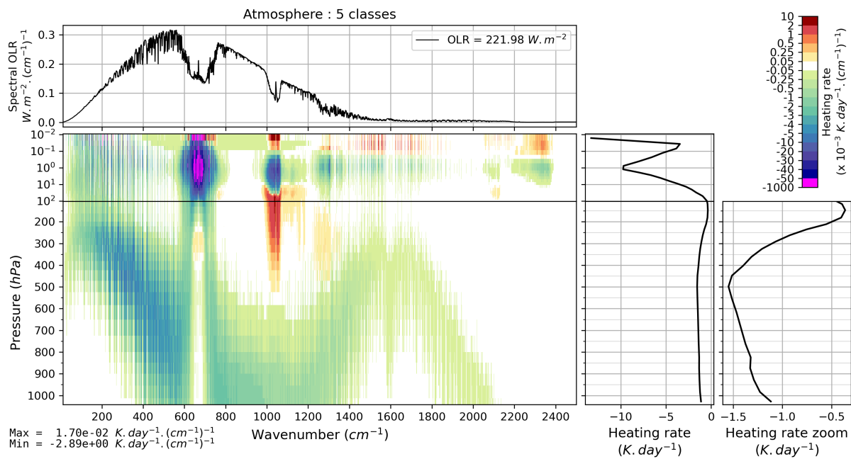
FIGURE 3.2 – OLR et taux de chauffage moyennés sur les cinq situations moyennes TIGR. En haut à gauche est représenté le spectre d'OLR et sa valeur intégrée entre 10 et 2500 cm^{-1} . En bas à gauche se trouve le taux de chauffage en fonction du nombre d'onde et du niveau de pression. En bas au centre se trouve le profil de taux de chauffage intégré entre 10 et 2500 cm^{-1} . En bas à droite est représenté un zoom sur le taux de chauffage dans la troposphère.
