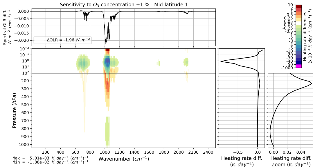
FIGURE B.37 – Effet d’une augmentation verticalement uniforme de 1 % de la concentration d’ozone sur l’OLR et le taux de chauffage vertical pour l’atmosphère moyenne Mid-latitude 1 de TIGR 2000.
