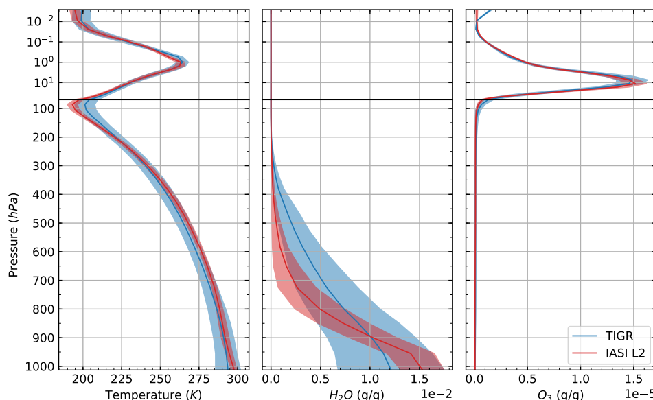
FIGURE 5.13 – Profils atmosphériques moyens (courbe pleine) et plage \pm 1 écart type (zones colorées) pour les types de masses d'air tropicales des bases TIGR (bleu) et IASI L2 (rouge). Le profil de température se trouve à gauche, au centre se trouve le profil de concentration de vapeur d'eau et à droite le profil de concentration d'ozone.
