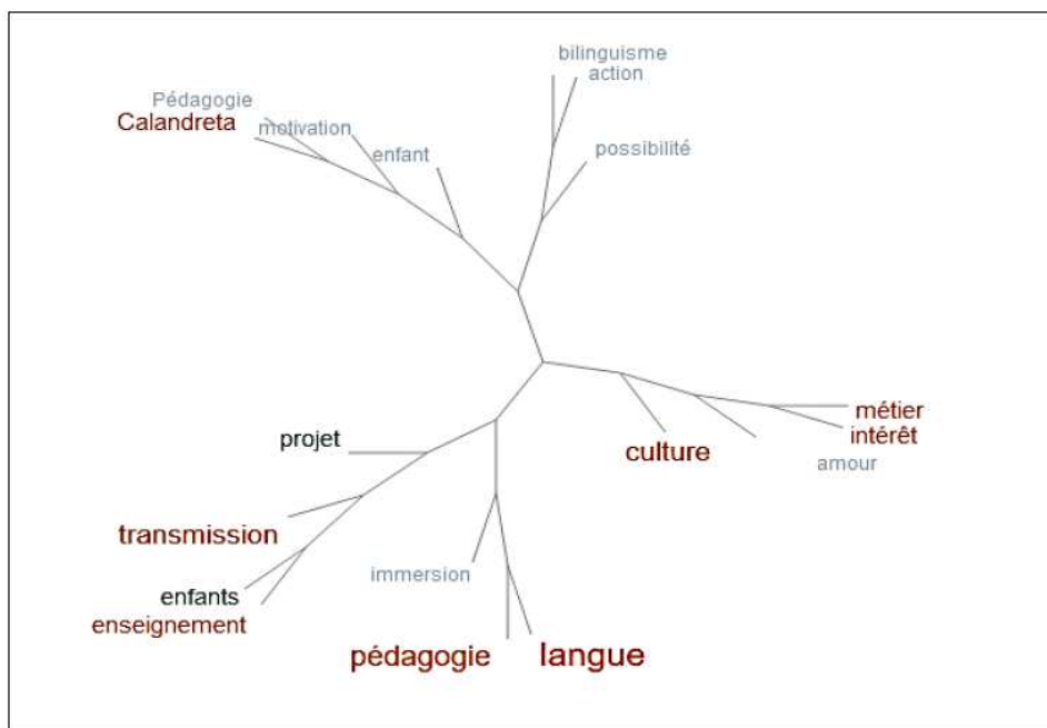
Figure n°19 : nuage arboré 154
