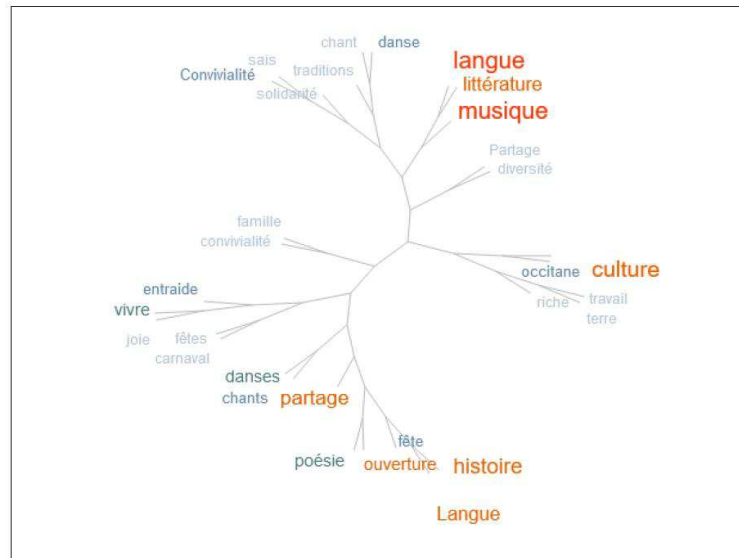
Figure 16 : nuage arboré 152
