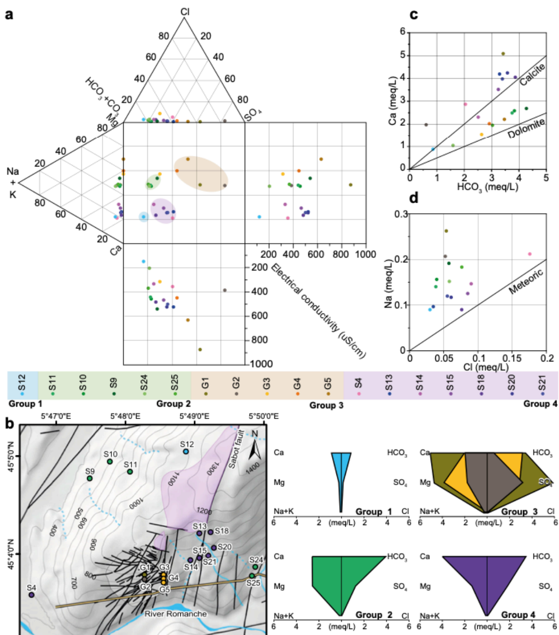
Figure 33 : Analyse hydrogéochimique des sources drainant le massif de Séchilienne avec a. Diagramme de Durov. b. Carte de localisation et diagrammes de Stiff. c. Concentrations Ca vs HCO 3 et d. Concentrations Na vs Cl (Vallet et al., 2015).
