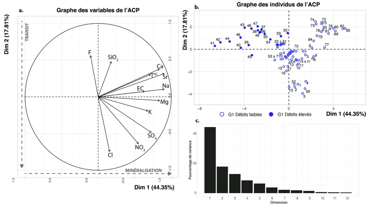
Figure 79: Analyse en composantes principales de l'exutoire G1 sur la composition chimique et les paramètres physico-chimiques (température T °C , conductivité électrique EC) des prélèvements automatiques datés d'octobre 2015 à octobre 2017 ; a. Graphique des variables, b. Graphique des individus, c. Pourcentages de variance.
