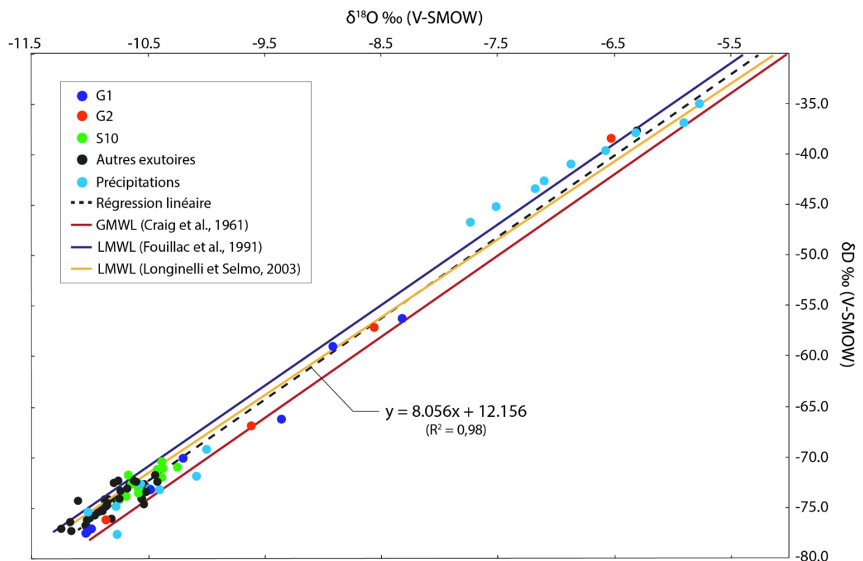
Figure 90: Diagramme \delta^{18}\text{O} and \delta\text{D} pour les échantillons d'eau du versant de Séchilienne et les eaux pluviales. Les lignes météorologiques tracées correspondent à la Droite Météorique Mondiale DML (GMWL ; Craig, 1961). La Droite Météorique Locale du massif central DML (LMWL ; Fouillac et al., 1991), la Droite Météorique Locale pour l'Italie du Nord DML (NILMWL ; Longinelli et Selmo, 2003).
