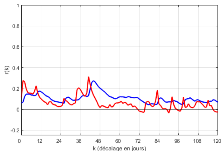
Figure 53: Corrélation croisée sur l'année hydrologique 2015/2016 entre la pluie efficace (PE ; variable d'entrée) et le débit (Q ; variable de sortie) pour les exutoires G1 (bleu) et G2 (rouge).
