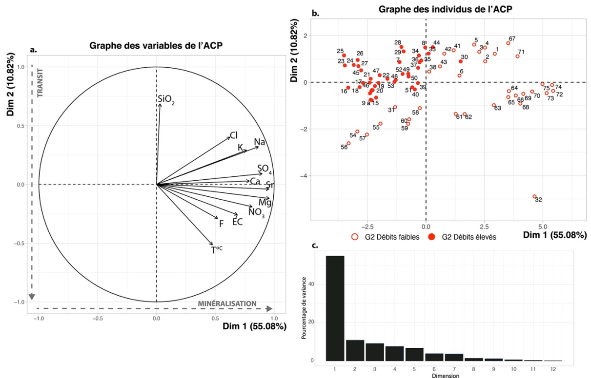
Figure 80: Analyse en composantes principales de l'exutoire G2 sur la composition chimique et les paramètres physico-chimiques (température T^{°C} , conductivité électrique EC) des prélèvements automatiques datés d'octobre 2015 à octobre 2017 ; a. Graphique des variables, b. Graphique des individus, c. Pourcentages de variance.
