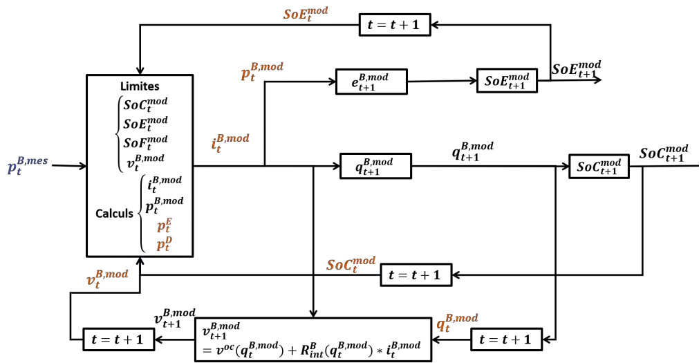
FIGURE III.26 – Synoptique du modèle OCVR
