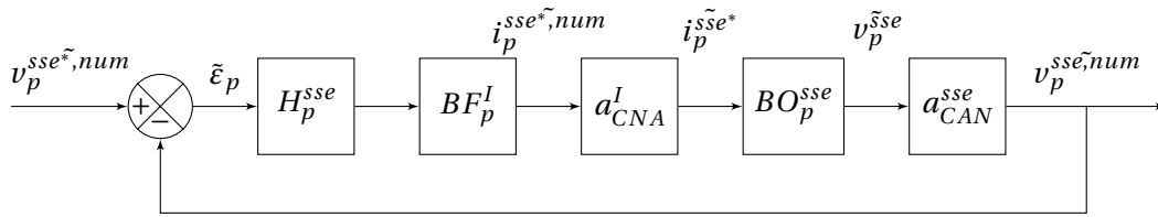
FIGURE 8 – Schéma bloc de la BdT du SSE en numérique et en BF à partir du modèle moyen "petit signal"
