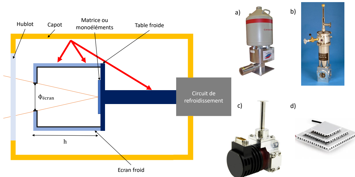
FIGURE 1.7 – Schéma de principe d'un détecteur infrarouge. Sont présentés aussi différentes méthode de refroidissement a) cryostat à bain b) cryostat à circulation c) machine à froid de type Stirling et d) un module Peltier (à 3 étages ici). Dans le cas du module Peltier, il n'y a pas de doigt froid, le détecteur est fixé directement sur le module.
