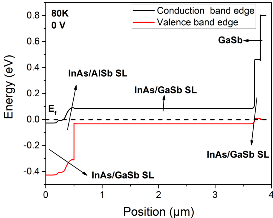
FIGURE 3.19 – Diagramme de bandes de la barrière à 80K et 0V [Alchaar et al., 2019].
