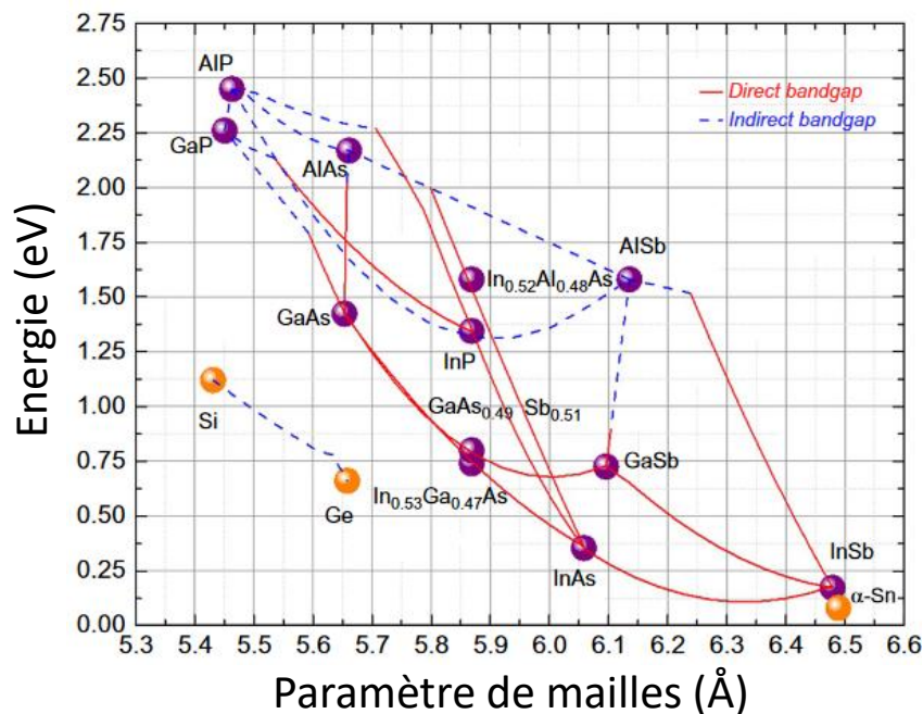
FIGURE 1.8 – Énergie de bande interdite en fonction du paramètre de maille pour des semiconducteurs III-V et II-VI.
