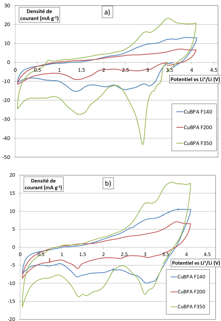
Figure 143 : Voltammétrie cyclique de CuBPA fluorés à différentes températures a) Premier cycle b) Deuxième cycle Vitesse de balayage : 0,02 mV/s
