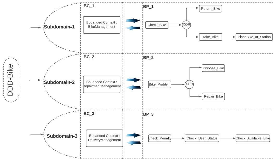
FIGURE 2.13: Illustration d'une conception dirigée par domaine
