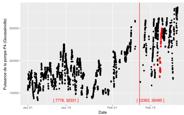
(n) Puissance hydraulique générée par la pompe P4 (du circuit vers le chauffage urbain 2)
