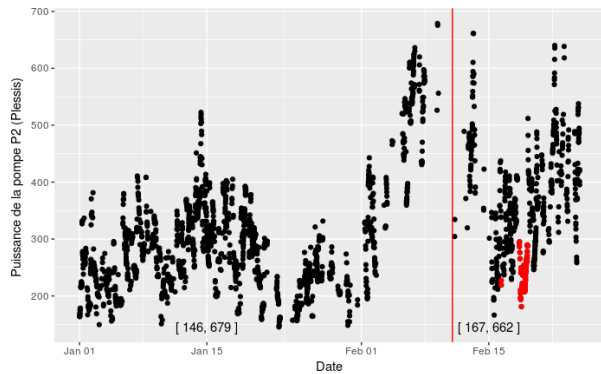
(l) Puissance hydraulique générée par la pompe P2 (du circuit vers le chauffage urbain 1)
