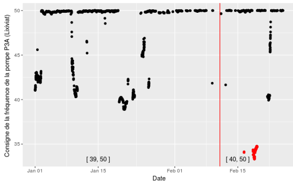
(g) Consigne de fréquence du variateur électronique de la pompe P3A (du circuit vers le procédé industriel)
