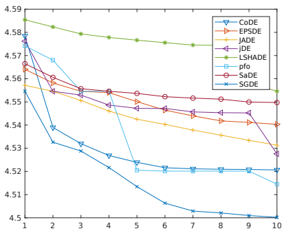
(c) 1EDP
