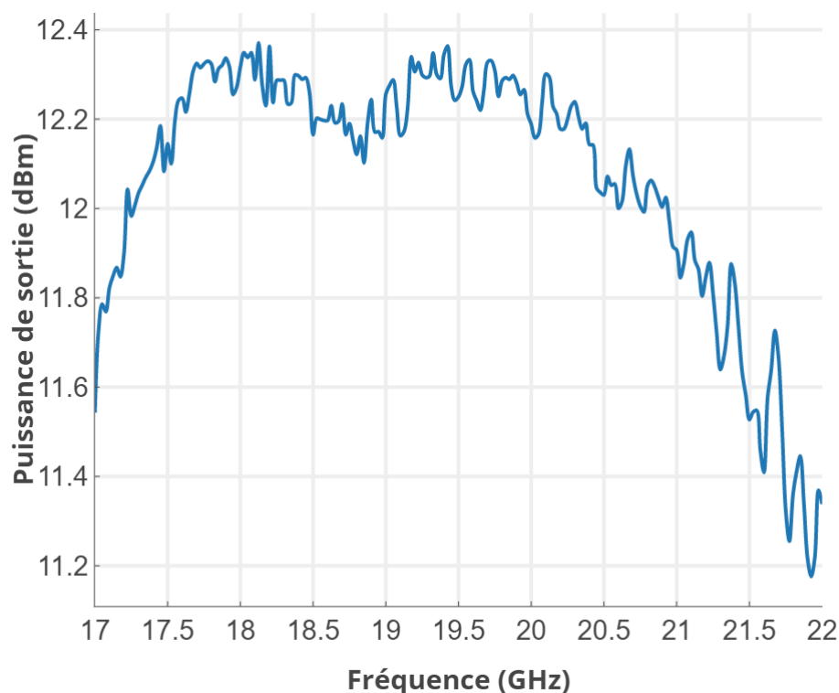
Figure 3.10 – Puissance de sortie en dBm en fonction de la fréquence à puissance d’entrée de saturation fixé à -1.2 dBm
