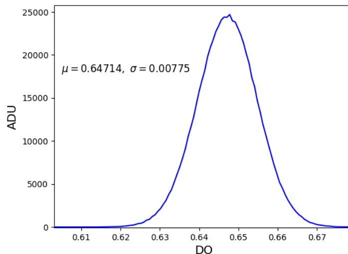
Figure III-43. Exemple d'historgramme de densités optiques dans une région d'intérêt circulaire de 15 mm de diamètre, obtenu pour un film pleinement irradié à 10 Gy.
