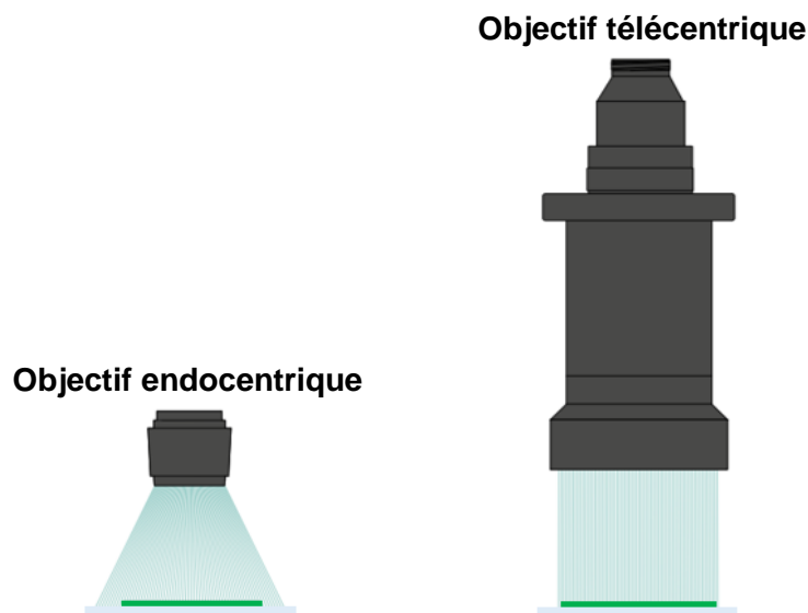
Figure III-13. Objectif endocentrique (à gauche) et télécentrique (à droite).
