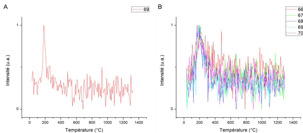
Figure 104 : Fragments de masse supérieure à m/z = 60 détectés A. dans le produit S3 et B. dans le produit S4
