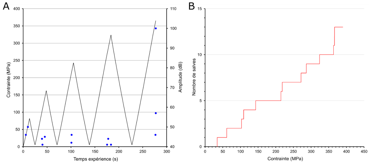
Figure 155 : A. Contraite appliquée et B. émission acoustique lors d'un essai en cyclage de SPS_Co_4
