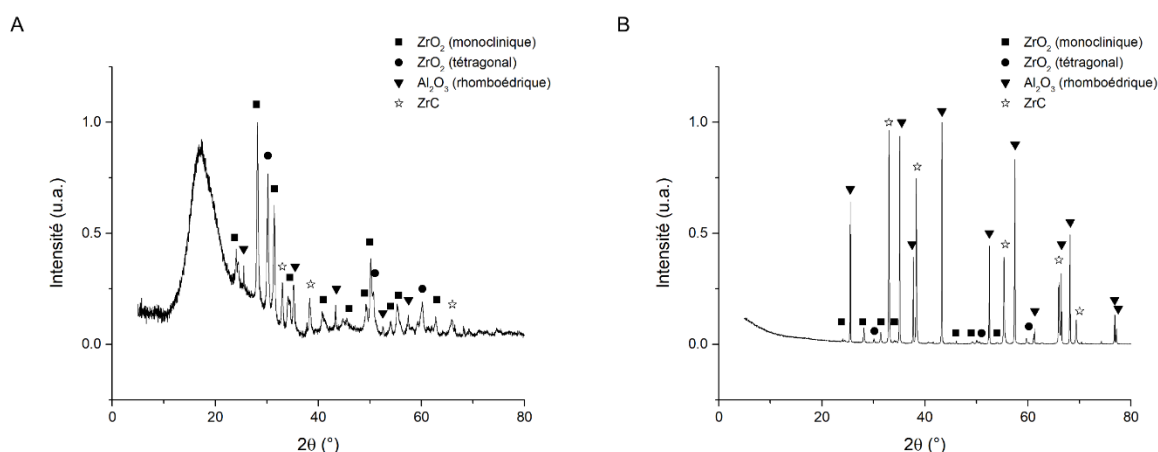
Figure 100 : Diffractogrammes des produits A. S2 et B. S3 après traitement thermique sous argon à respectivement 1300^\circ C et 1550^\circ C pendant 2 heures
