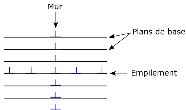
Figure 126 : Schéma de principe des murs et des empilements de dislocation par rapport aux plans de base [270]
