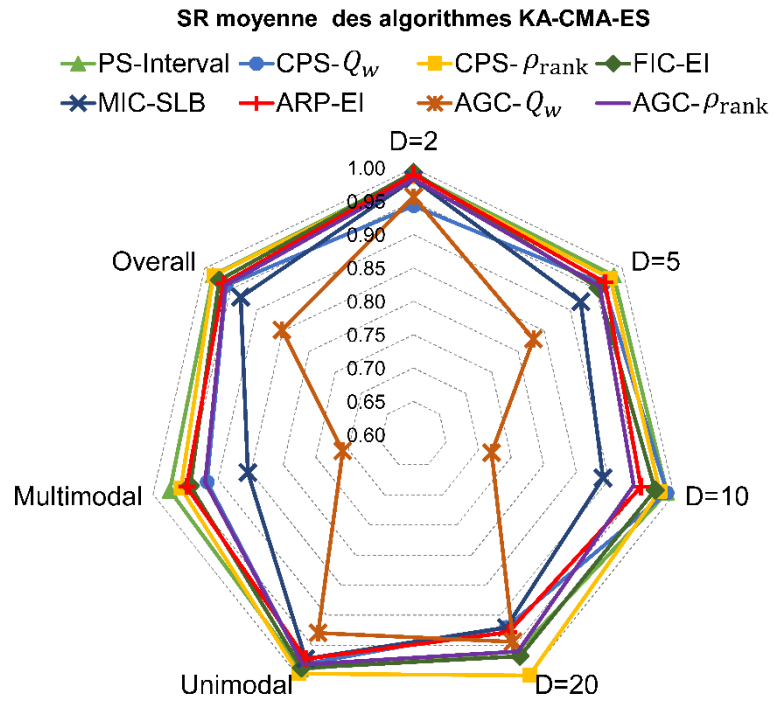
Figure 6.13 Comparaison du taux de réussite moyen (SR) des algorithmes KA-CMA-ES.
