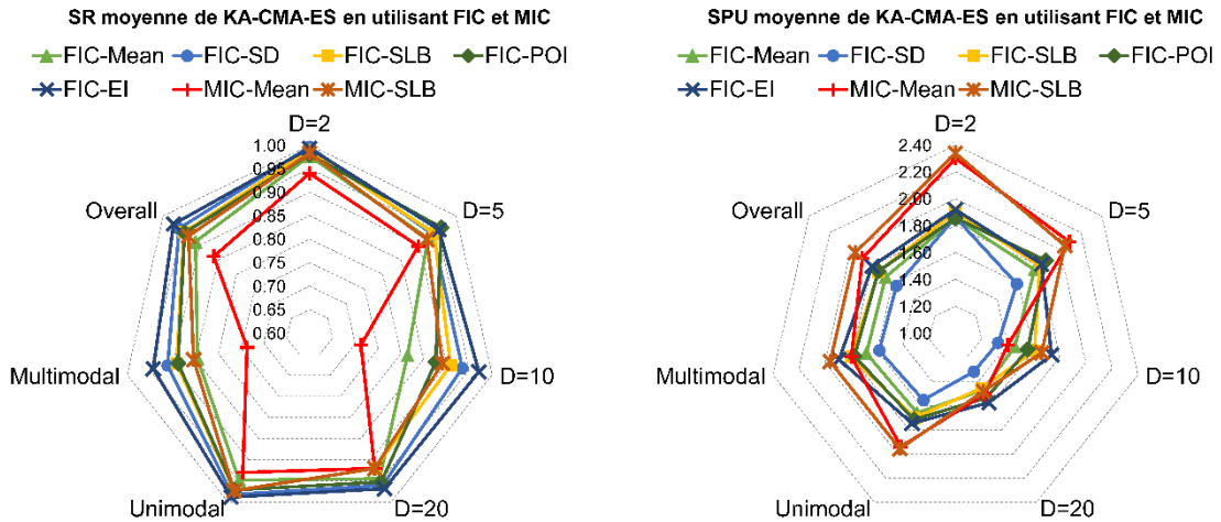
Figure 6.10 Moyenne SR et SPU de KA-CMA-ES en utilisant un contrôle individuel fixe et mixte (FIC et MIC).
