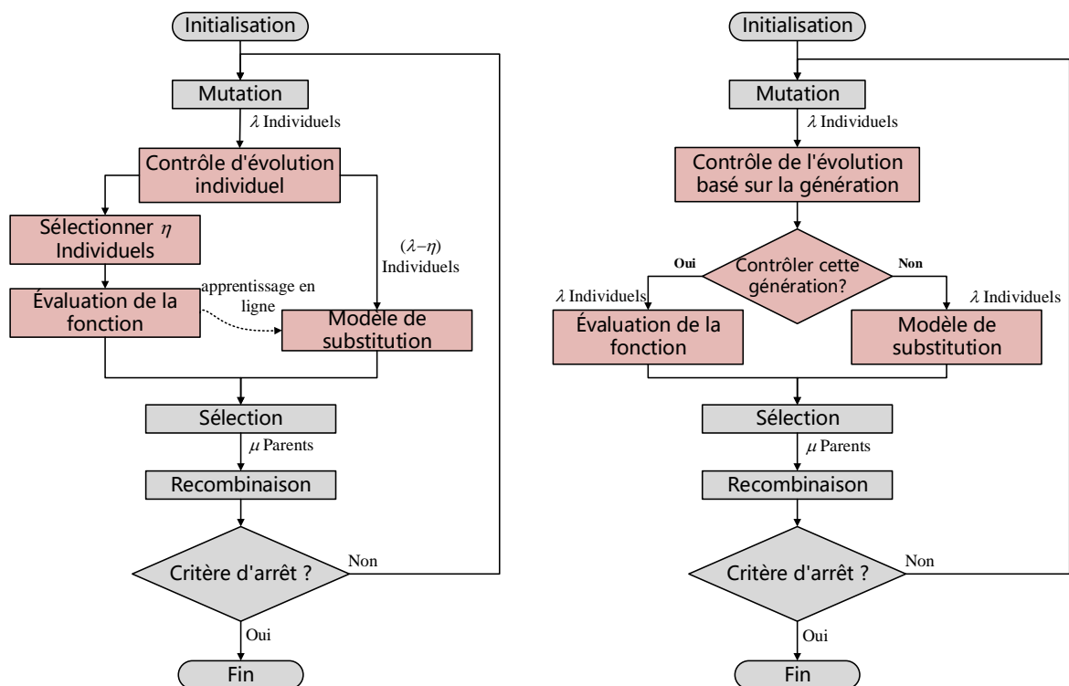
Figure 6.4 Illustration du contrôle de l'évolution dans la stratégie d'évolution assisté par substitution : (1) contrôle basé sur l'individu et (2) contrôle basé sur la génération.
