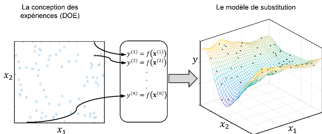
Figure 6.2 Processus de modélisation de substitution
