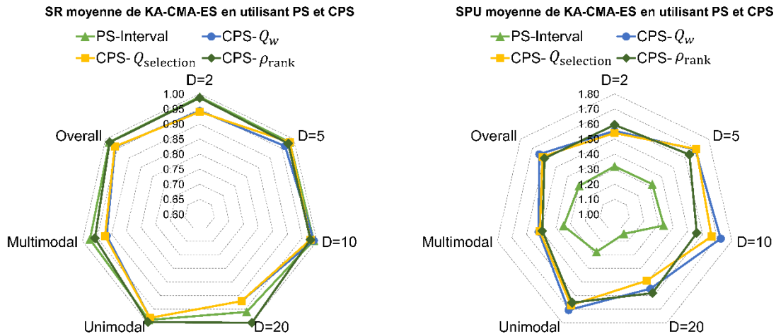
Figure 6.7 Taux moyen de réussite et accélération de la présélection sans et avec le contrôle de l'impact du modèle.
