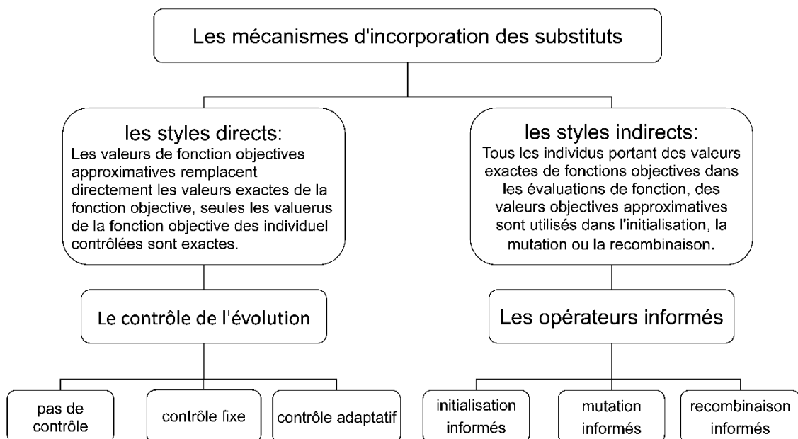
Figure 6.1 Les mécanismes d'incorporation des modèles de substitution dans les EAs
