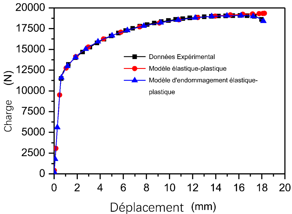
Figure 6.20 Comparaison des courbes force-déplacement des modèles élastique-plastique et élastique-plastique avec les paramètres identifiés
