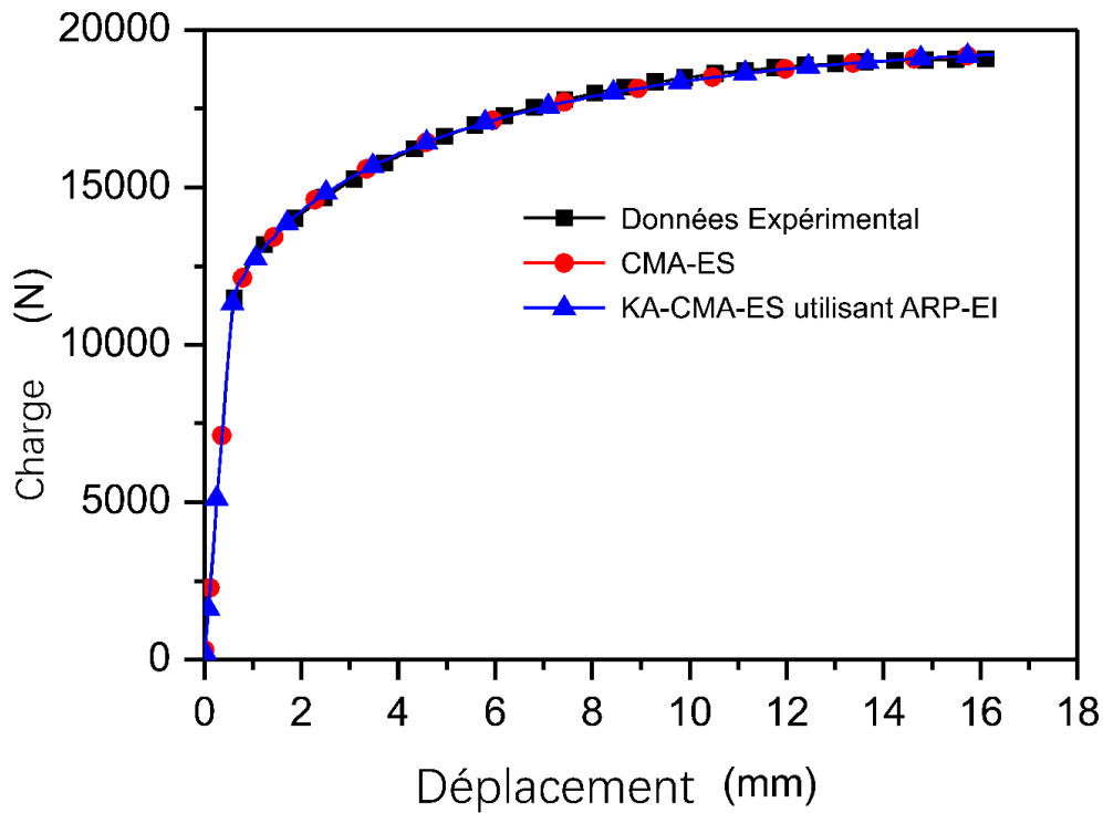
Figure 6.17 Courbes de déplacement de force (avant étrangement) correspondant à des paramètres de durcissement de contrainte identifiés et données expérimentales
