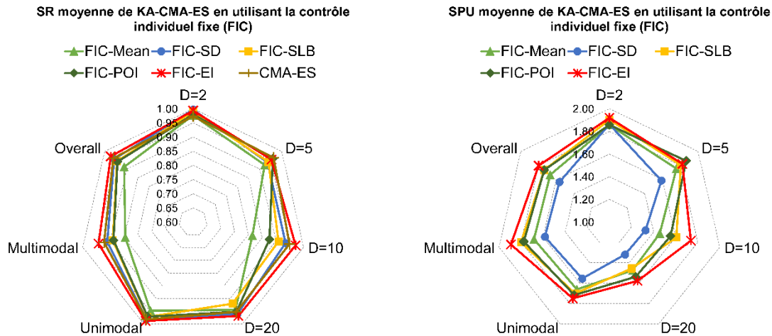
Figure 6.8 Taux moyen de réussite (SR) et performance d'accélération (SPU) de KA-CMA-ES en utilisant un contrôle individuel fixe avec différentes mesures.
