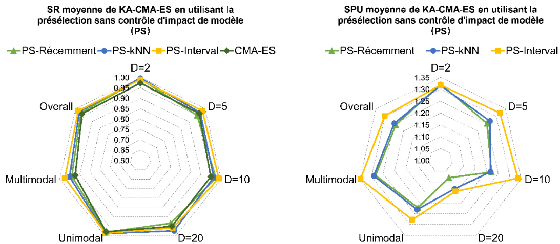
Figure 6.5 Taux de réussite moyen et des performances d'accélération de KA-CMA-ES en utilisant la présélection sans contrôle de l'impact du modèle (PS).
