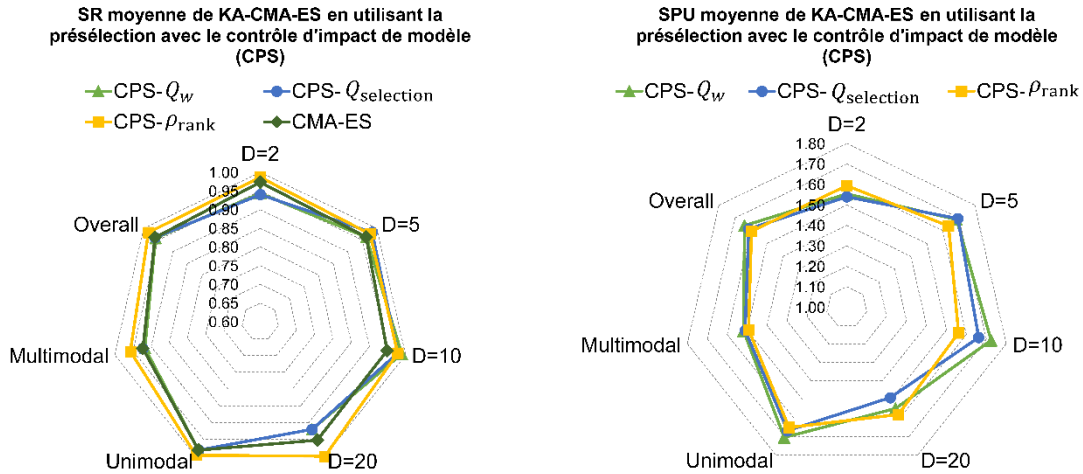
Figure 6.6 Taux moyen de réussite et taux de présélection supérieur à celui du contrôle de l'impact du modèle à l'aide de différentes mesures de la qualité du modèle.
