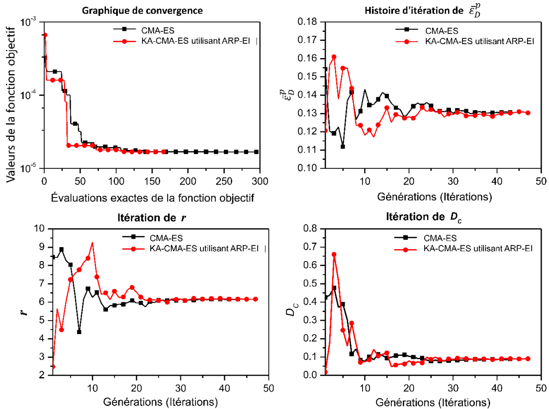
Figure 6.18 Graphes de convergence et d'itération de l'identification des paramètres d'endommagement
