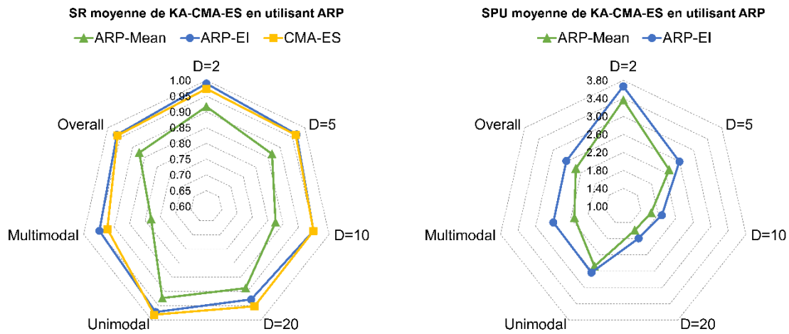
Figure 6.11 Taux moyen de réussite et performance d'accélération de KA-CMA-ES en utilisant ARP.
