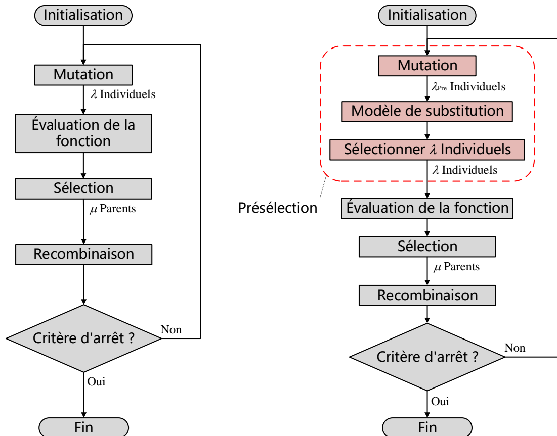
Figure 6.3 Illustration de la présélection dans la stratégie d'évolution assistée par modèle de substitution: (1) la norme (\mu, \lambda) -ES et (2) l'ES assistée par la présélection.
