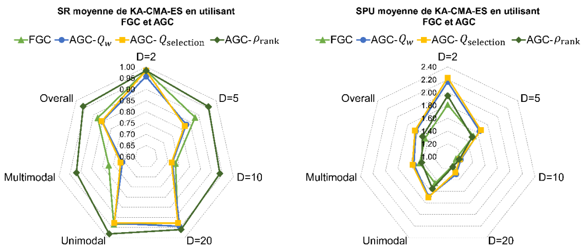
Figure 6.12 Taux moyen de réussite et accélération de KA-CMA-ES en utilisant FGC et AGC.
