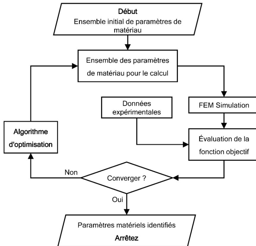
Figure 6.15 La procédure d'identification des paramètres
