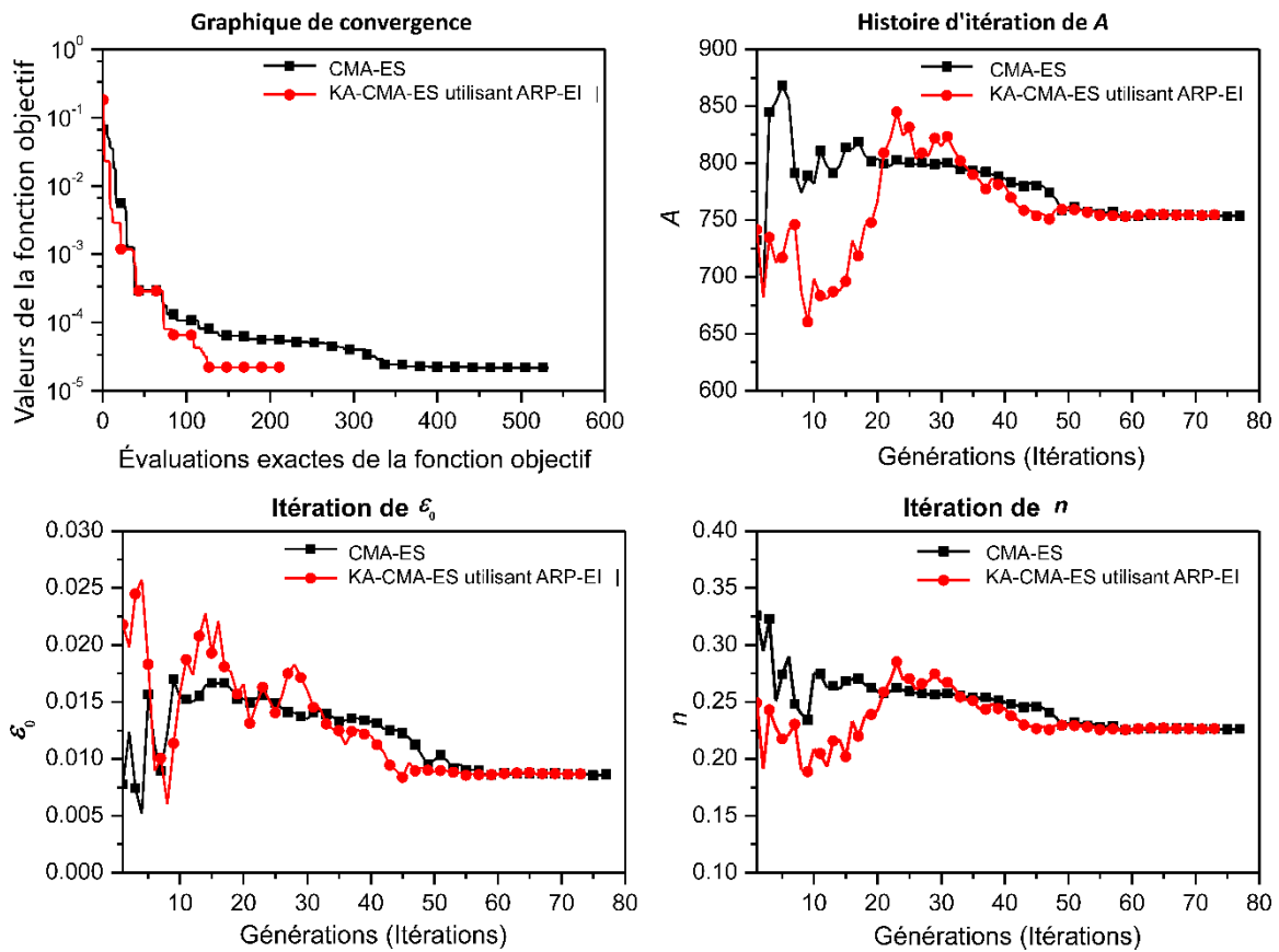
Figure 6.16 Graphes de convergence et d'itération de l'identification des paramètres de durcissement
