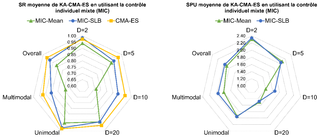
Figure 6.9 Taux moyen de réussite (SR) et performance d'accélération (SPU) de KA-CMA-ES en utilisant un contrôle mixte individuel (MIC).
