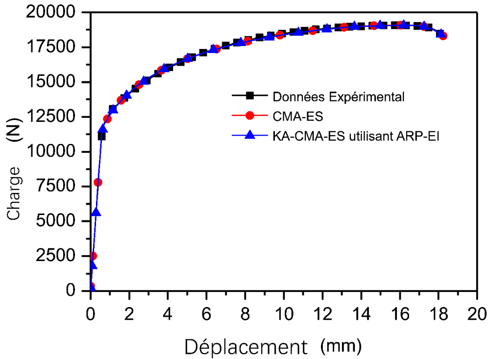
Figure 6.19 Courbes de force-déplacement correspondant aux paramètres d'endommagement identifiés et données expérimentales
