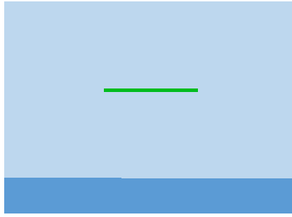
Figure 154. Guide d'onde en SiN (vert) interré dans de la silice (bleu ciel) sur substrat Si (bleu)
