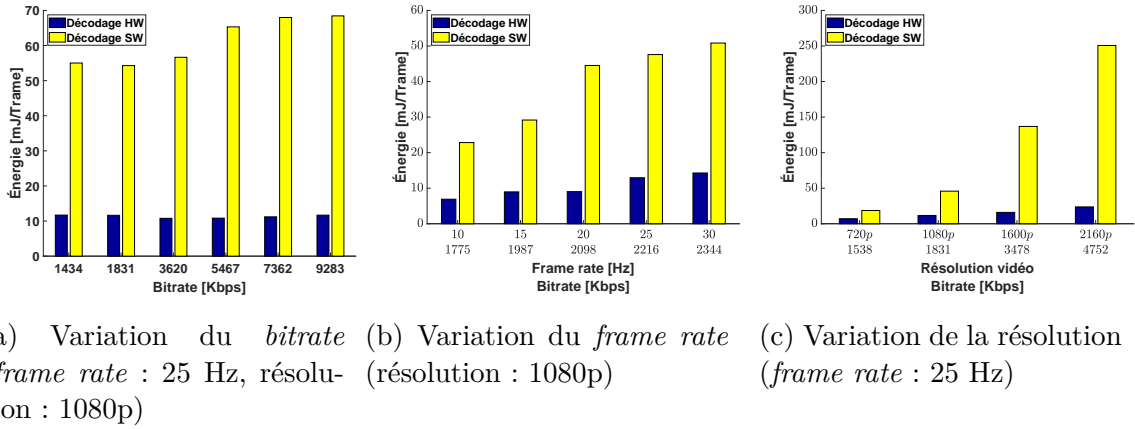
Figure 7.12 – Consommation énergétique des décodages HEVC HW vs SW (Séquence vidéo : kimono, QPs : 21 to 37, PSNRs : 22.97 à 43.8, plateforme : RB3)
