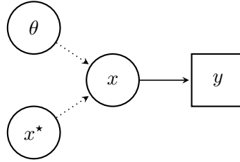
Figure 1.2.: Graph orienté acyclique de la paramétrisation non centrée.
