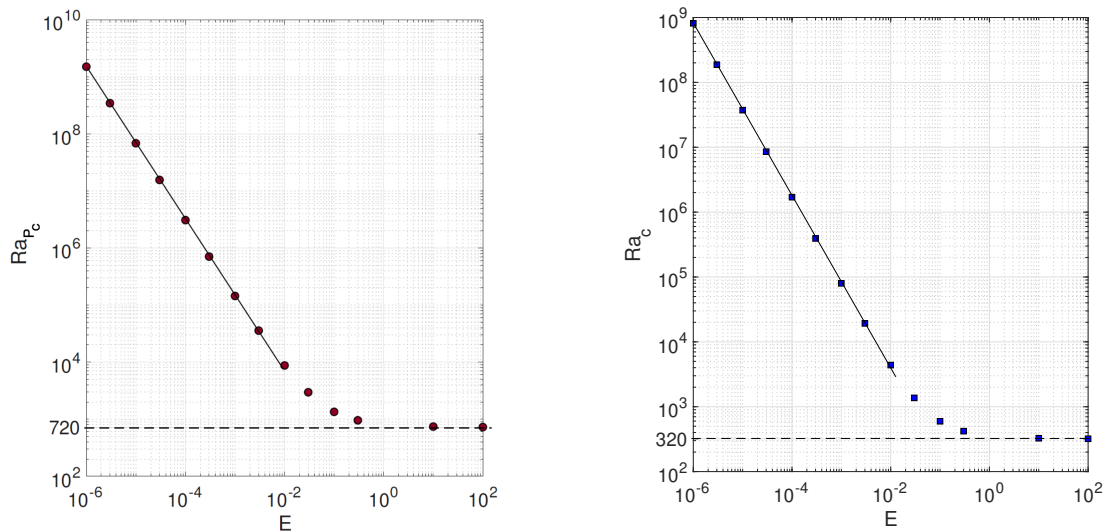
Figure 5.3: Gauche : Stabilité de la convection radiative en rotation pour les conditions aux limites NS-SF et \ell/H = 0.05 . La ligne pointillée correspond au Ra_{Pc} calculé par Goluskin sans rotation. La ligne continue correspond à Ra_{Pc} = 14.775E^{-4/3} . A droite : stabilité de la convection RB pour les conditions aux limites NS-SF. La ligne continue est la loi d'échelle pour la rotation en géométrie de RB. La ligne pointillée correspond au Ra_{Pc} calculé par Goluskin sans rotation.
