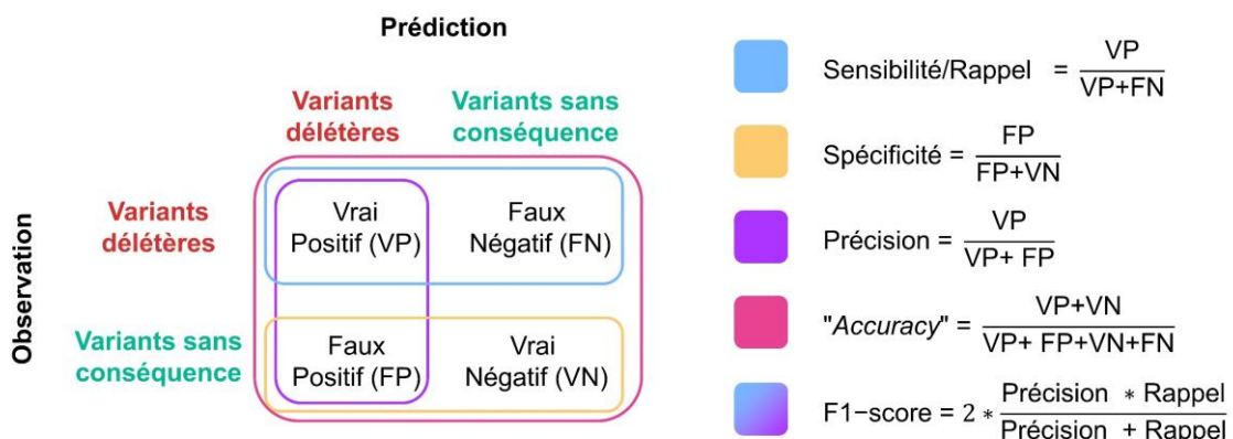
Figure 30 – Métriques d'évaluation des outils de prédiction Source personnelle avec inspiration de newbiettn.github.io
