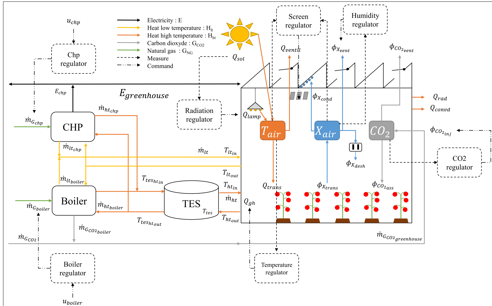
FIGURE 4.9 – Schéma de la serre agricole avec les variables climatiques, les équipements supports et les régulateurs.
