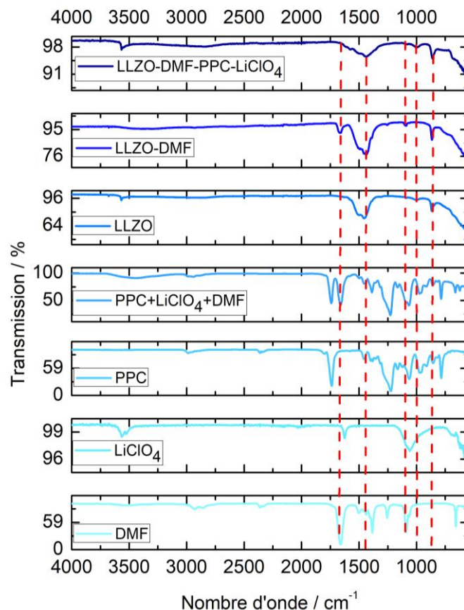
Figure IV.32. De bas en haut : spectres infrarouge du DMF, du \text{LiClO}_4 , du PPC, du PPC/ \text{LiClO}_4 , du LLZO, du LLZO fritté sans PPC/ \text{LiClO}_4 et avec du DMF, du LLZO fritté avec du PPC/ \text{LiClO}_4 et avec du DMF.
