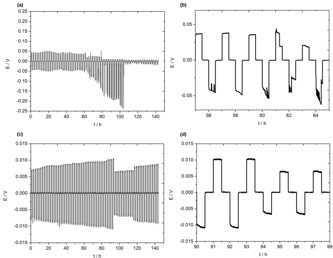
Figure III.47. Cyclage galvanostatique à une densité de courant de 50 \mu\text{A}.\text{cm}^{-2} et à 22^\circ\text{C} des cellules symétriques \text{Li-Al} \mid 5\% \text{Li}_3\text{BO}_3\text{-LLZO} \mid \text{Li-Al} à différentes pressions. a) sous une pression de 0,09 \text{ MPa} , b) agrandissement du moment à partir duquel un court-circuit doux a été observé, c) sous une pression de 0,4 \text{ MPa} et d) agrandissement du moment auquel une diminution de la polarisation a été observée.
