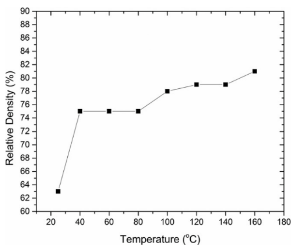
Figure IV.4. Influence de la température sur la densité relative finale du LAGP pour une pression fixée à 400 MPa pendant 20 min[6].
