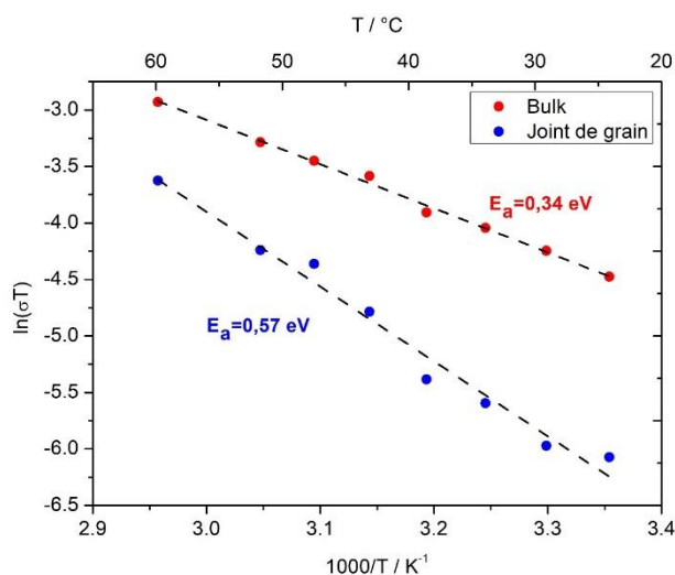
Figure III.24. Tracé d'Arrhénius correspondant à la conductivité ionique en fonction de la température d'une pastille de LLZO fritté à 1150°C pendant 12 h sans \text{Li}_3\text{BO}_3 . Les données correspondantes au bulk et aux joints de grain sont données en rouge et en bleu respectivement.
