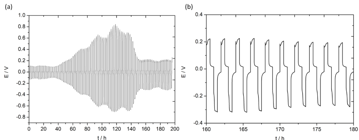
Figure IV.35. Profil de cyclage de la cellule symétrique Li/LP30/LLZO-PPC-LiClO 4 -DMF/LP30/Li à un courant de 75 \mu\text{A}.\text{cm}^{-2} pendant (a) 200h et (b) agrandissement entre 160h et 180h. Une pression de 0,09 MPa a été exercée sur la cellule.
