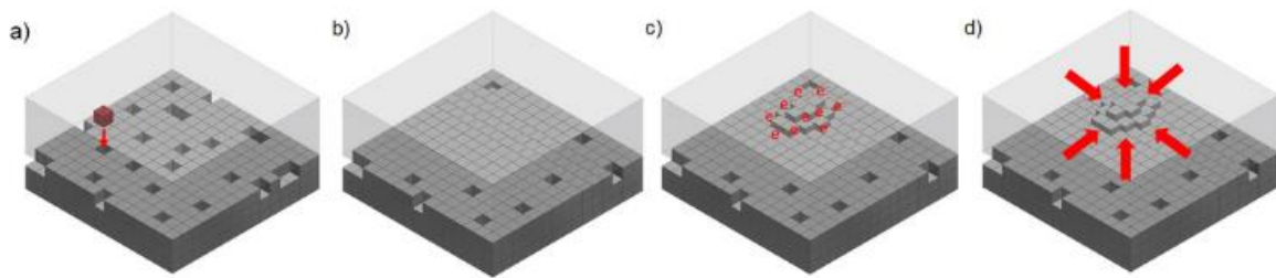
Figure III.8. Illustration de l'interface entre le lithium en gris foncé et le LLZO en gris clair. a) à faible densité de courant le lithium se dépose dans des sites vacants b) à une densité de courant proche de la CCD, la mobilité du lithium devient trop faible c) la surface de l'électrode n'a pas le temps de se reconstruire ce qui mène à une mauvaise distribution du courant, certaines zones étant plus riche en électrons que d'autres d) le lithium s'accumule préférentiellement dans ces zones riche électriquement par recombinaison d'un ion \text{Li}^+ et d'un électron créant ainsi des « points chauds » sur lesquels vont croître le lithium[40].
