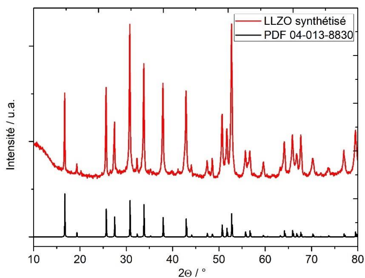
Figure III.11. Diagramme de diffraction des rayons X de la poudre de LLZO synthétisée (rouge).
