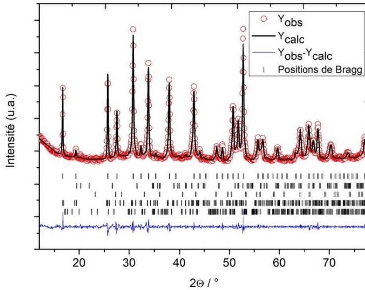
Figure III.12. Affinement par la méthode de Le Bail[60] de la poudre de LLZO synthétisée. Les données expérimentales et calculées sont représentées par des cercles rouges et une ligne noire respectivement. La différence entre les données expérimentales et les données calculées est représentée par une ligne bleue. Les positions de Bragg sont représentées par des marques noires verticales. De hauts en bas : LLZO cubique, \text{Li}_2\text{ZrO}_3 , \text{La}_2\text{Zr}_2\text{O}_7 , LLZO quadratique et \text{Li}_6\text{Zr}_2\text{O}_7 . R_p = 10.8\% , R_{wp} = 10.1\% , R_{exp} = 6.73\% et \chi^2 = 2.27 .
