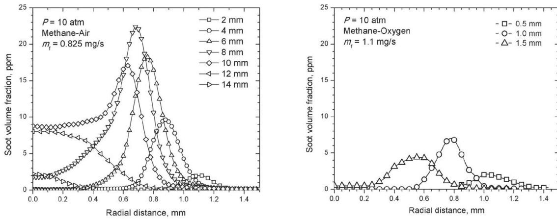
Figure 1.16: Évolution de la formation des suies à P=10 \text{ atm} pour le méthane-air avec un débit m_f = 0.825 \text{ mg/s} et méthane-oxygène avec un débit m_f = 1.1 \text{ mg/s} [104].
