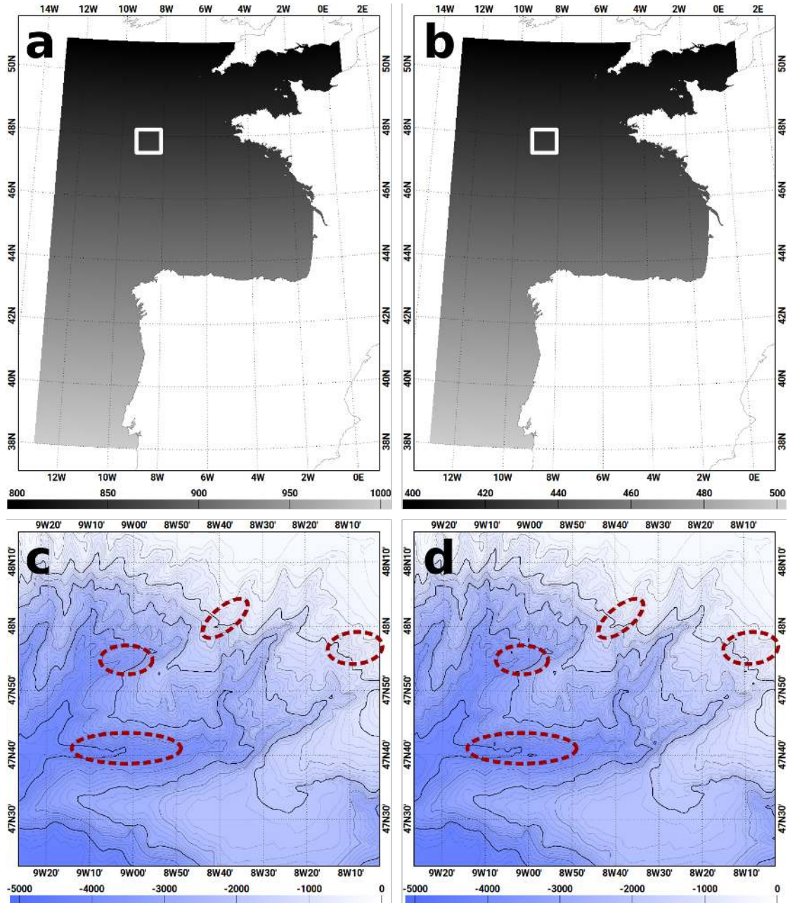
FIGURE 3.1 – Résolution des configurations BOBIBE avec (a) une grille à 1000 m et (b) une grille à 500 m et (c-d) détail de la bathymétrie du banc de la Petite Sole. Le carré blanc indique la localisation du détail de bathymétrie. Les zones en pointillés rouges soulignent quelques zones où la bathymétrie change d'une configuration à l'autre.
