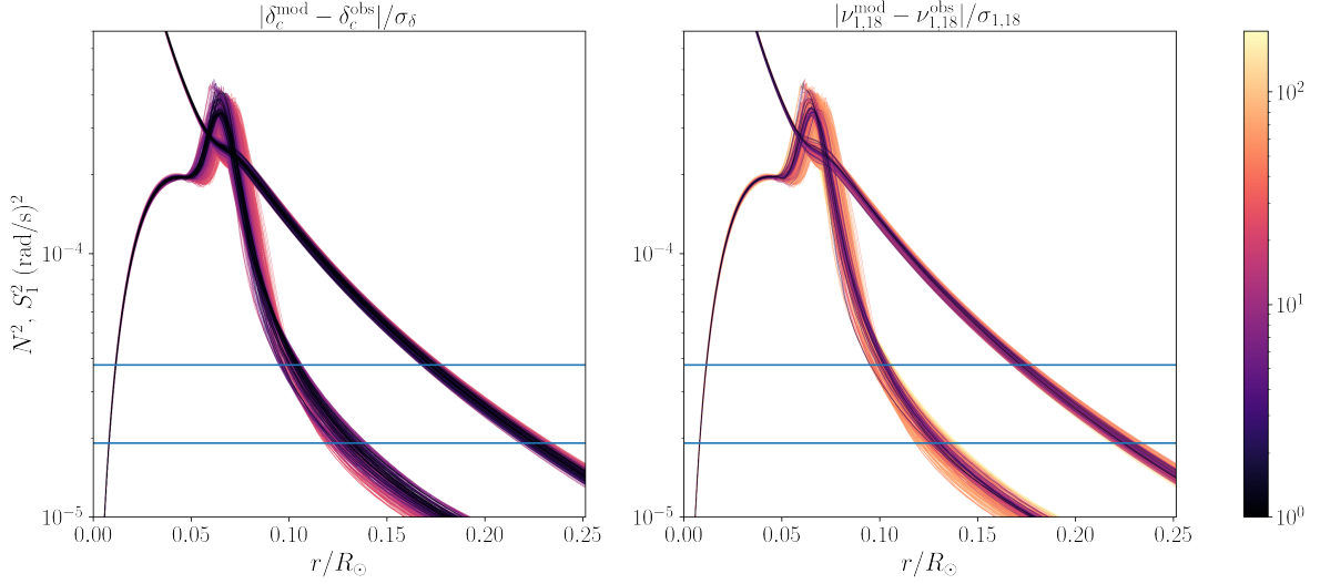
FIGURE 7.8. – Profils de N^2 et de S_1^2 des modèles de la grille grossière. Les profils de gauche et de droite sont respectivement colorés selon les accords avec les observations de \delta_c et \nu_{1,18} . Les lignes horizontales représentent les fréquences angulaires observées des modes g-dominés
