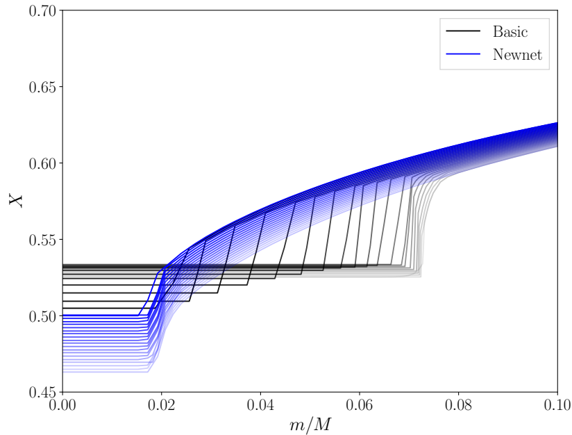
FIGURE 9.10. – Evolution du profil en X d'un modèle juste après ajout d'overshoot. Chaque profil est représenté à chaque itération en temps, du plus foncé au plus clair. En bleu le modèle est calculé avec un réseau newnet, analogue au cas d'un mélange diffusif, alors que le modèle en noir est calculé avec un modèle basic, analogue au cas d'un mélange instantané.
