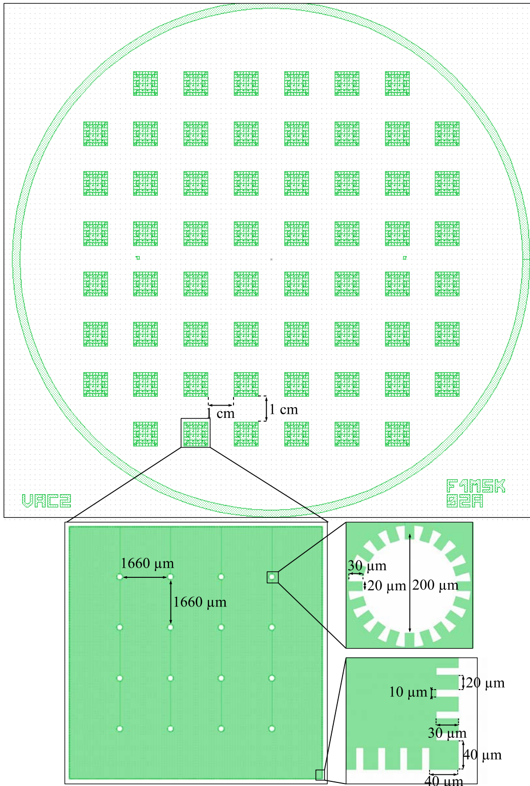
Figure H-3 : Design du niveau F1MSK. Les motifs apparaissent en champ clair sur le masque.
