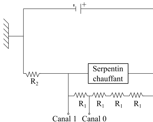
Figure I-2 : Schématisation du montage électrique du banc de test thermique.
