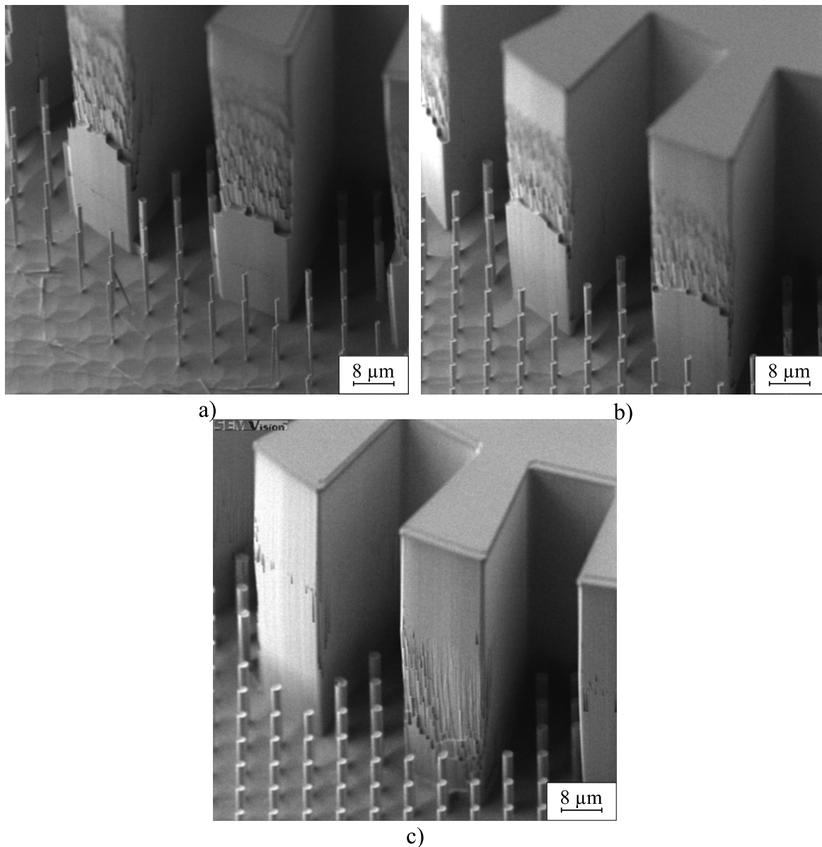
Figure 4-16 : Observation MEB de la mèche de micropiliers de 3 \mu\text{m} aux abords d'un des piliers de support pour trois recettes de gravure différentes : a) recette Cavit _1, b) recette Cavit _2 avec pression de gravure r duite et c) recette Cavit _3 avec pression et flux de \text{SF}_6 r duits.
