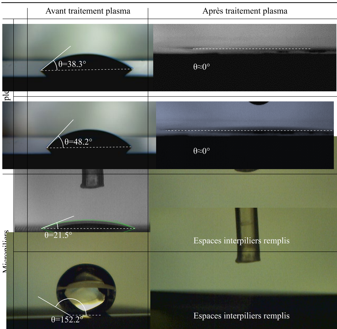
Figure 6-9 : Angle de contact avant et après traitement plasma O_2 , 150 W, 5 min dans le cas de micropiliers et de silicium plein porosifiés et non porosifiés.
