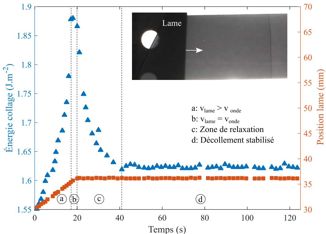
Figure 5-8 : Caractérisation de l'énergie de collage par méthode Maszara réalisée en atmosphère anhydre sur un échantillon recuit à 200°C et conditionné plusieurs mois en atmosphère de salle blanche.
