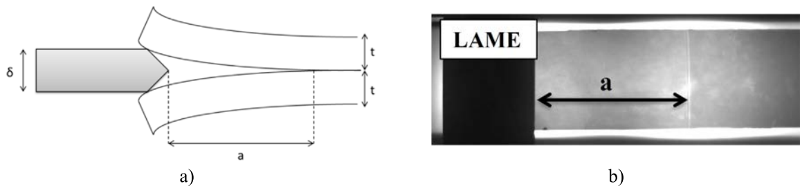
Figure 5-6 : Description de la méthode de mesure Maszara a) et observation IR du décollement d'une barrette échantillon d'un collage SiO 2 -SiO 2 b) [89].
