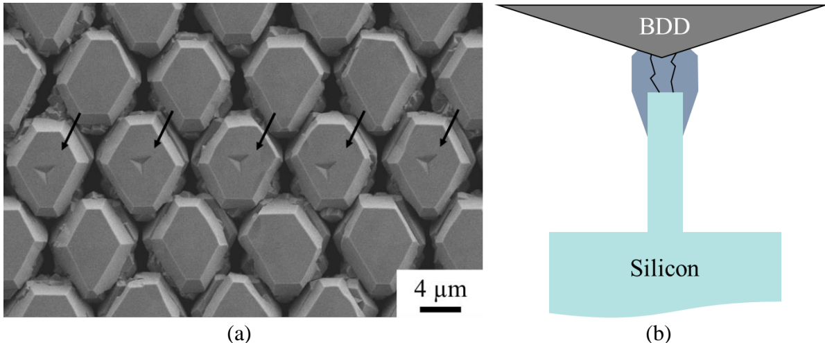
Figure IV.24 – (a) Image MEB des empreintes résiduelles (pointées par des flèches) laissées sur les îlots d'AlN avec une pointe Berkovich. (b) Schéma du système. La pointe Berkovich introduit des défauts dans le matériau menant à des fuites de courant électrique (schématisées par les deux traits noirs).
