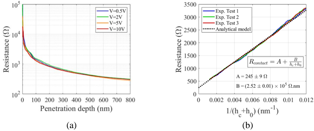
Figure III.8 – (a) Courbes brutes R - h obtenues sur l’or massif monocristallin avec une pointe Berkovich en BDD sous différentes tensions de polarisation. (b) Courbes de résistance électrique en fonction de l’inverse de la profondeur de contact idéale calculée avec le modèle d’Oliver-Pharr dans le domaine d’autosimilarité de la pointe. Régression linéaire afin de calculer les coefficient A et B de calibration électrique du système [24].
