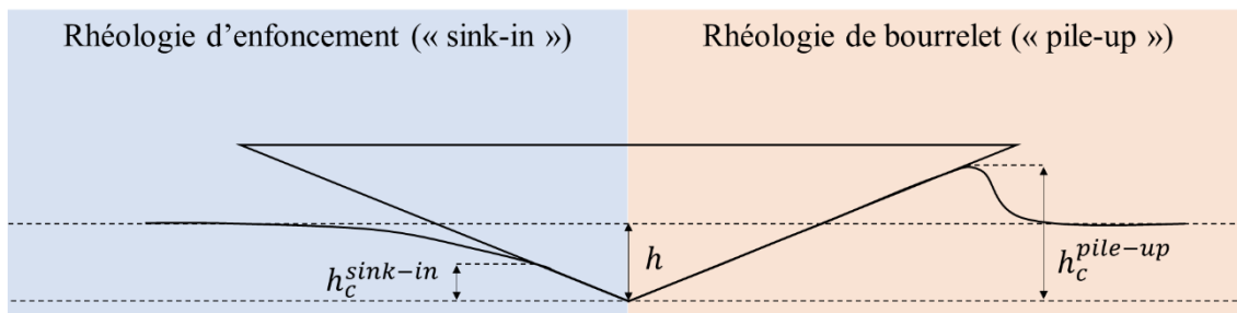
Figure I.10 – Schéma des différentes rhéologies des matériaux pouvant influencer la topologie du contact mécanique.
