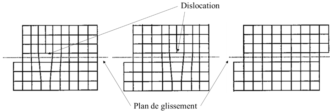
Figure I.5 – Schéma d’une dislocation dans un réseau cristallographique et de sa propagation sur un plan de glissement (de gauche à droite).
