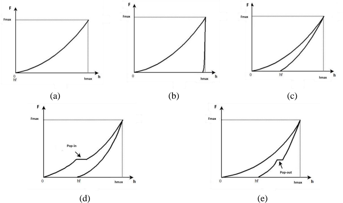
Figure I.7 – Courbes force-profondeur typiques d'un matériau (a) élastique parfait, (b) plastique parfait, (c) élastoplastique quelconque, (d) dans lequel un événement irréversible soudain se manifeste par l'apparition d'un pop-in, (e) dans lequel un événement irréversible soudain se manifeste par l'apparition d'un pop-out. [8], [17].
