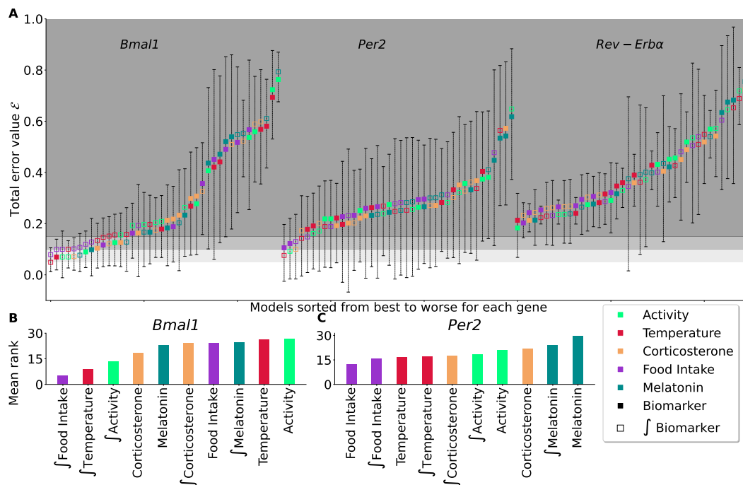
Figure 7: (A) Erreur totale pour chacun des modèles à 2 termes représentant un contrôle systémique sur la transcription de Bmal1 , Per2 ou Rev-Erb \alpha . Les couleurs indiquent les régulateurs impliqués dans chaque modèle, le carré du haut faisant référence au régulateur au poids le plus élevé en valeur absolue. Les zones définies par différentes nuances de gris font référence à des seuils d'erreur totale égaux à 0,05, 0,1 et 0,15. (B-C) Rang moyen des régulateurs parmi les modèles à 2 termes, du plus bas au plus élevé, pour les modèles ayant un impact sur la transcription de Bmal1 ou Per2 .
