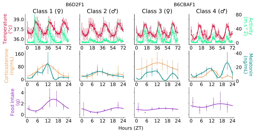
Figure 6: Biomarqueurs circadiens dans quatre classes de souris. Les données brutes sont représentées par des points (moyenne) et des barres d'erreur (écarts types). Pour des raisons de lisibilité, les barres d'erreur n'ont été affichées que toutes les 2,5 heures pour la première ligne. Les lignes pleines représentent la fonction moyenne obtenue par l'ajustement d'un processus Gaussien.
