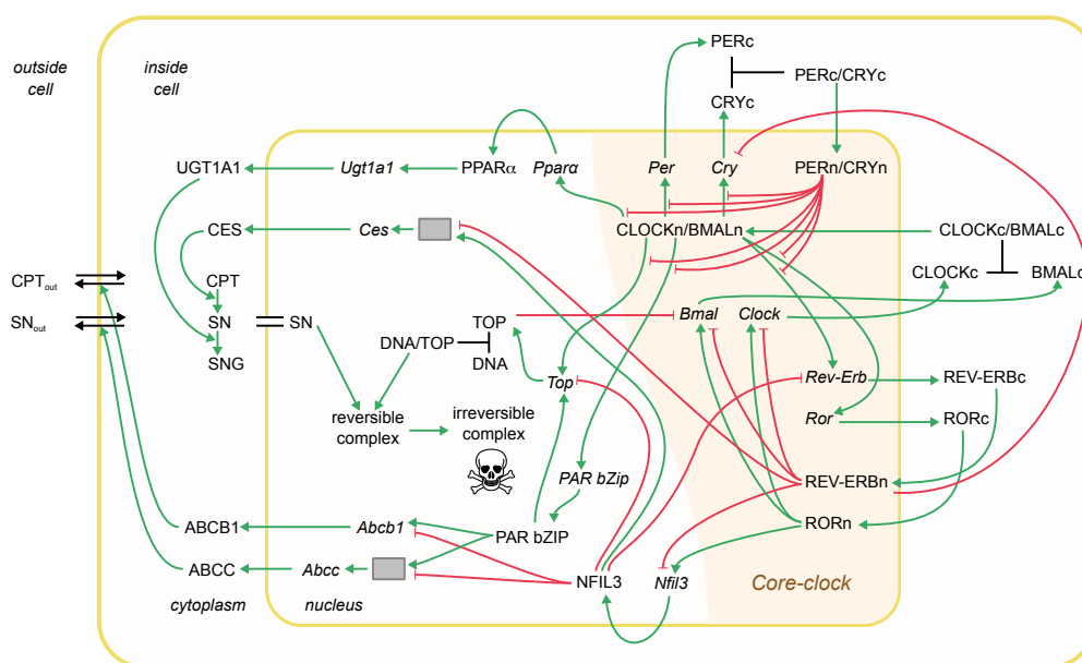
Figure 3: Le traitement de l'irinotecan est modélisé par un réseau transcription-traduction qui comprend l'horloge, les gènes pertinents pour l'irinotecan et la PK-PD de l'irinotecan. Les inhibitions sont représentées par des flèches rouges, les activations par des flèches vertes et la formation de complexes par des lignes noires. Les cases grises illustrent les sous-réseaux post-transcriptionnels nécessaires à l'ajustement du modèle aux données. La double ligne noire indique des concentrations égales entre le noyau et le cytoplasme. Les doubles flèches noires indiquent le transport cellulaire de CPT-11 et du SN-38 à l'intérieur et à l'extérieur de la cellule.
