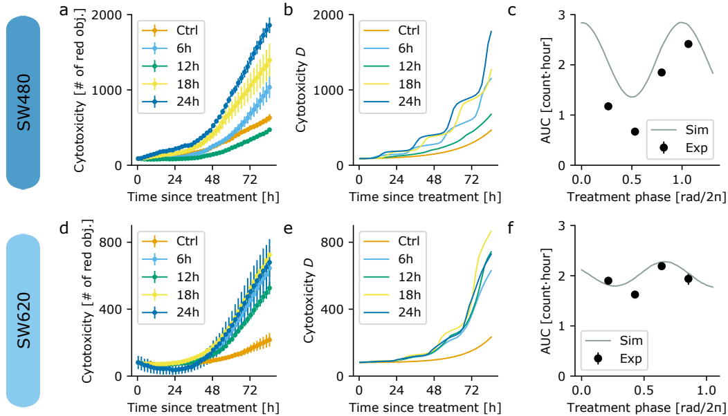
Figure 4: a-d Courbes de cytotoxicité mesurées expérimentalement, estimées par la mesure d'objets fluorescents rouges, pour des cellules SW480 non traitées (Ctrl), ou traitées avec l'irinotecan aux points de temps indiqués (6h, 12h, 18h ou 24h après la synchronisation). Le temps est aligné sur le début du traitement. b-e Ajustement du modèle PK-PD aux données expérimentales de cytotoxicité des lignées cellulaires SW480/SW620 (nombre de cellules mortes affiché, correspondant à la variable D de l'Equation (2.559)). c-f Aire sous la courbe des cellules SW480/SW620 traitées normalisée par le contrôle non traité (points noirs), comparée à l'aire sous la courbe pour le modèle ajusté (ligne grise).
