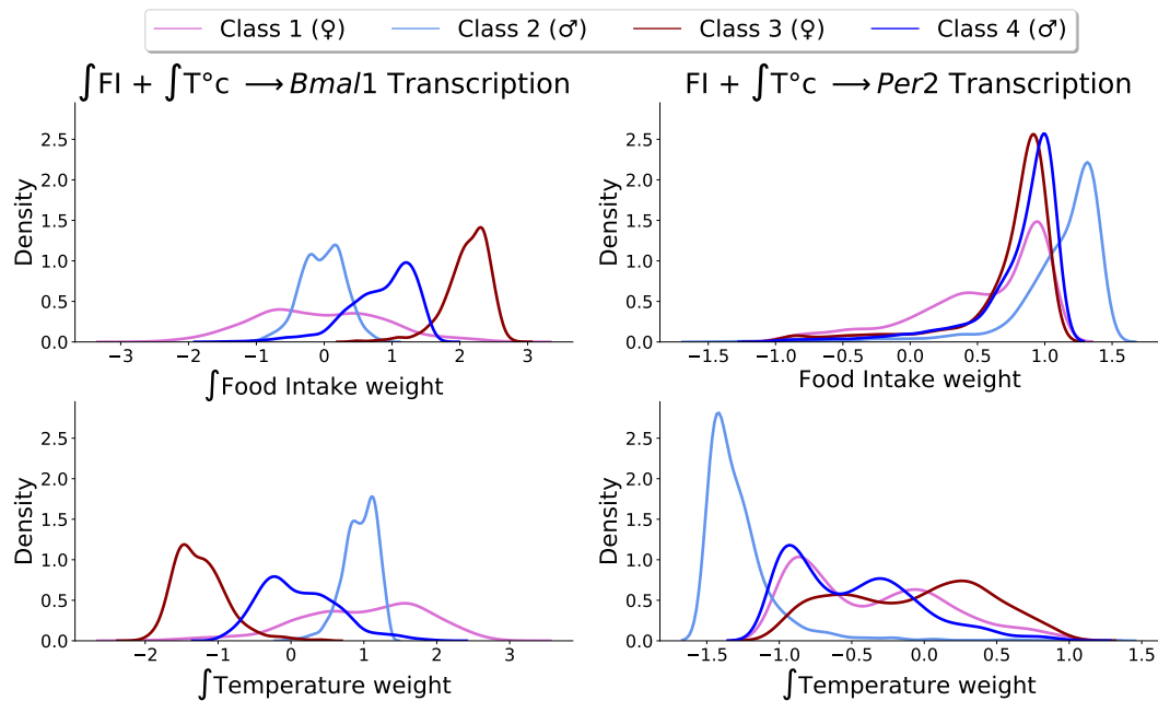
Figure 8: Densité des coefficients du meilleur modèle à 2 termes pour Bmal1 et Per2 , calculé sur les trajectoires résiduelles pour chaque classe de souris. FI : Apport alimentaire, T°C : Température.
