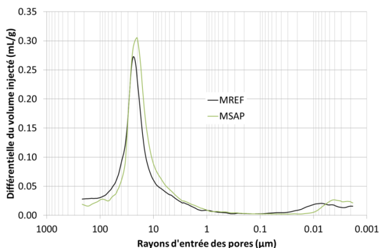
Figure III-19 - Distribution porale des échantillons de montmorillonite non traitée (MREF) et traitée à la saponine (MSAP). Courbes obtenues par intrusion de mercure dans les échantillons.
