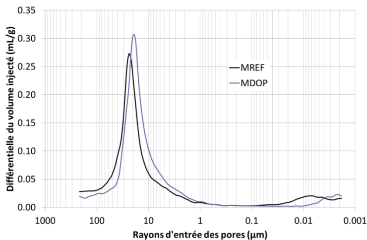
Figure III-23 - Distribution porale des échantillons non traités (MREF) et traité à la dopamine (MDOP). Courbes obtenues par intrusion de mercure dans les échantillons.
