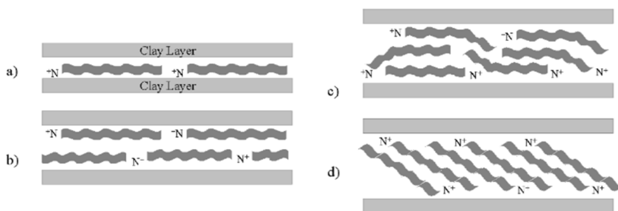
Figure I-28 - Configurations potentielles des cations d'alkylammoniums dans l'espace interfoliaire. (a) : adsorption en monocouche ; (b) : adsorption en bicouche ; (c) : adsorption en pseudo trois couches ; (d) : adsorption en assemblage paraffine (Lagaly, 1982, 1986; Bonczek et al., 2002).
