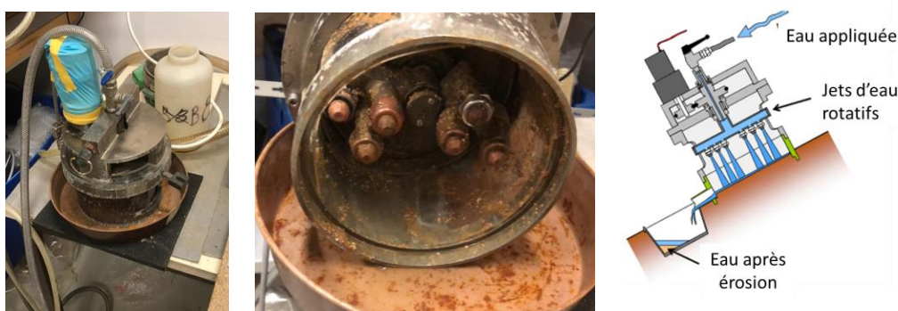
Fig. Annexes 46 – Schématisation du système d'érosion à l'eau MoJET (Haghighi, 2012).
