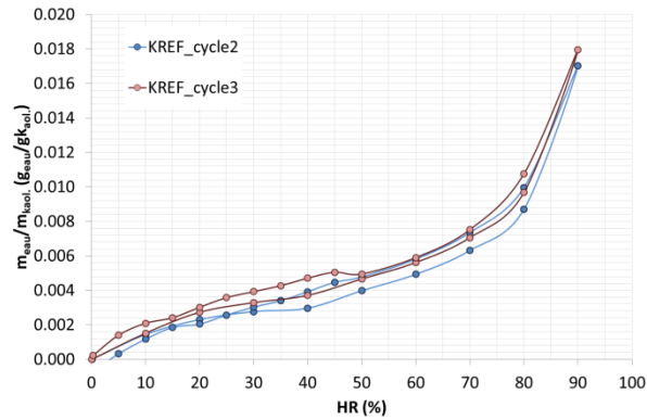
Figure IV-3 - Isothermes de sorption de l'eau sur la montmorillonite, l'illite et la kaolinite non traitées sur 3 cycles d'adsorption/désorption d'eau.
