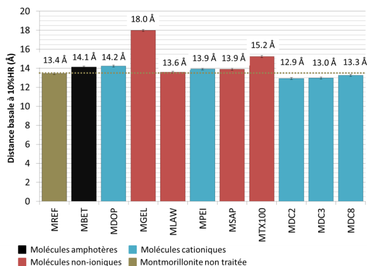
Figure III-2 – Distance basale de la montmorillonite après le traitement aux molécules organiques - 10%HR. En marron : montmorillonite non traitée ; en rouge : montmorillonite traitée avec les molécules non-ioniques ; en noir : montmorillonite traitée avec la molécule amphotère ; en bleu : montmorillonite traitée avec les molécules cationiques.
