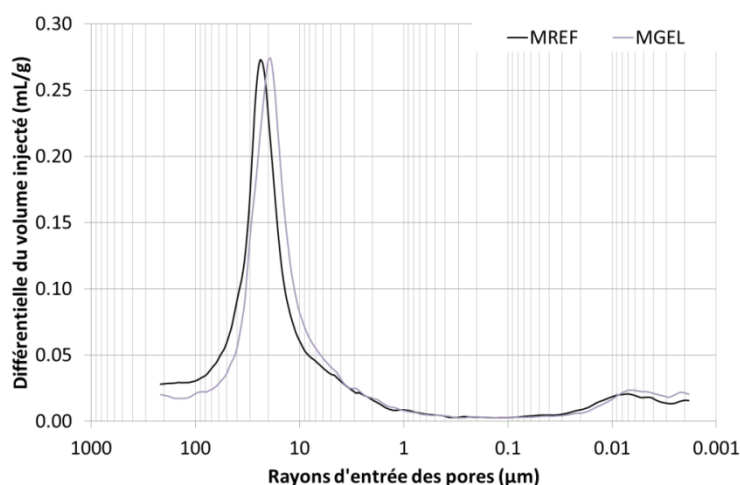
Figure III-18 - Distribution porale des échantillons de montmorillonite non traitée (MREF) et traitée à la gélatine de porc (MGEL). Courbes obtenues par intrusion de mercure dans les échantillons.
