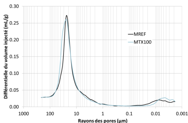
Figure III-20 - Distribution porale des éprouvettes de montmorillonite non traitée (MREF) et traitée au triton X100 (MTX100). Courbes obtenues par intrusion de mercure dans les éprouvettes.
