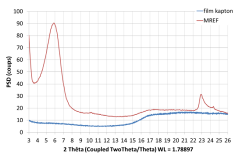
Figure II-3 - Diffractogrammes du film Kapton® seul et de la montmorillonite avec le film Kapton®
