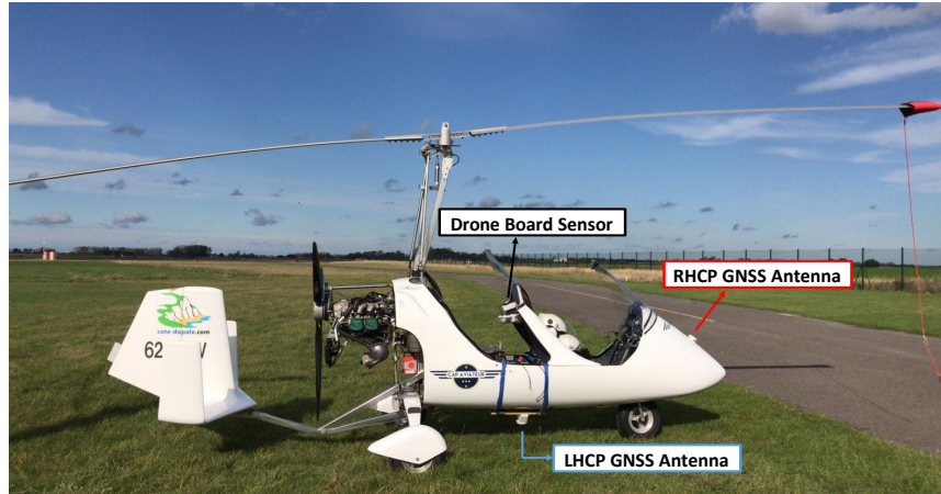
FIGURE 10: Autogire utilisé pour l'expérimentation, équipé des différents capteurs.
