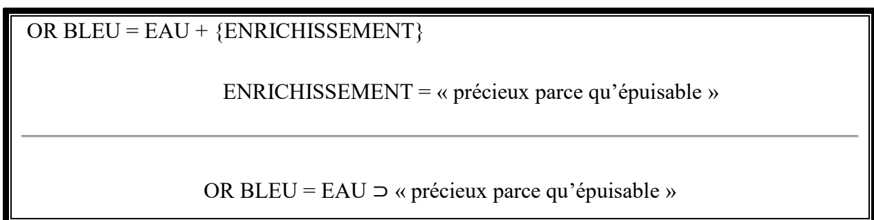
Figure 9 : Sens phraséologique enrichi de l'UP or bleu
