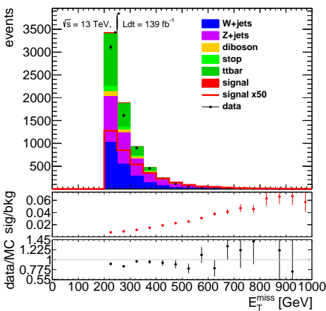
(e) E_T^{\text{miss}}
