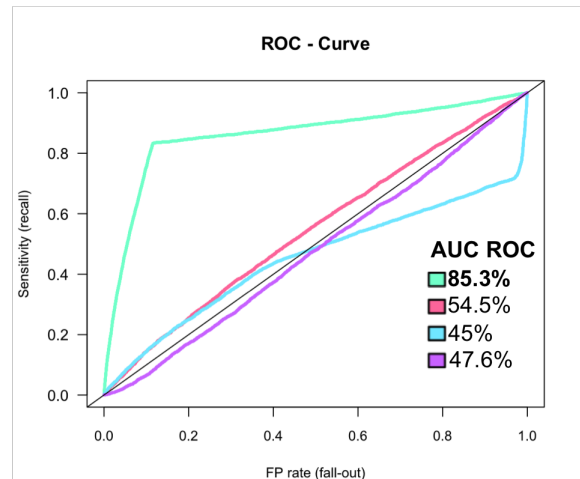
FIGURE 5.3 – Courbes ROC et PR pour E.coli et S. cerevisiae .
