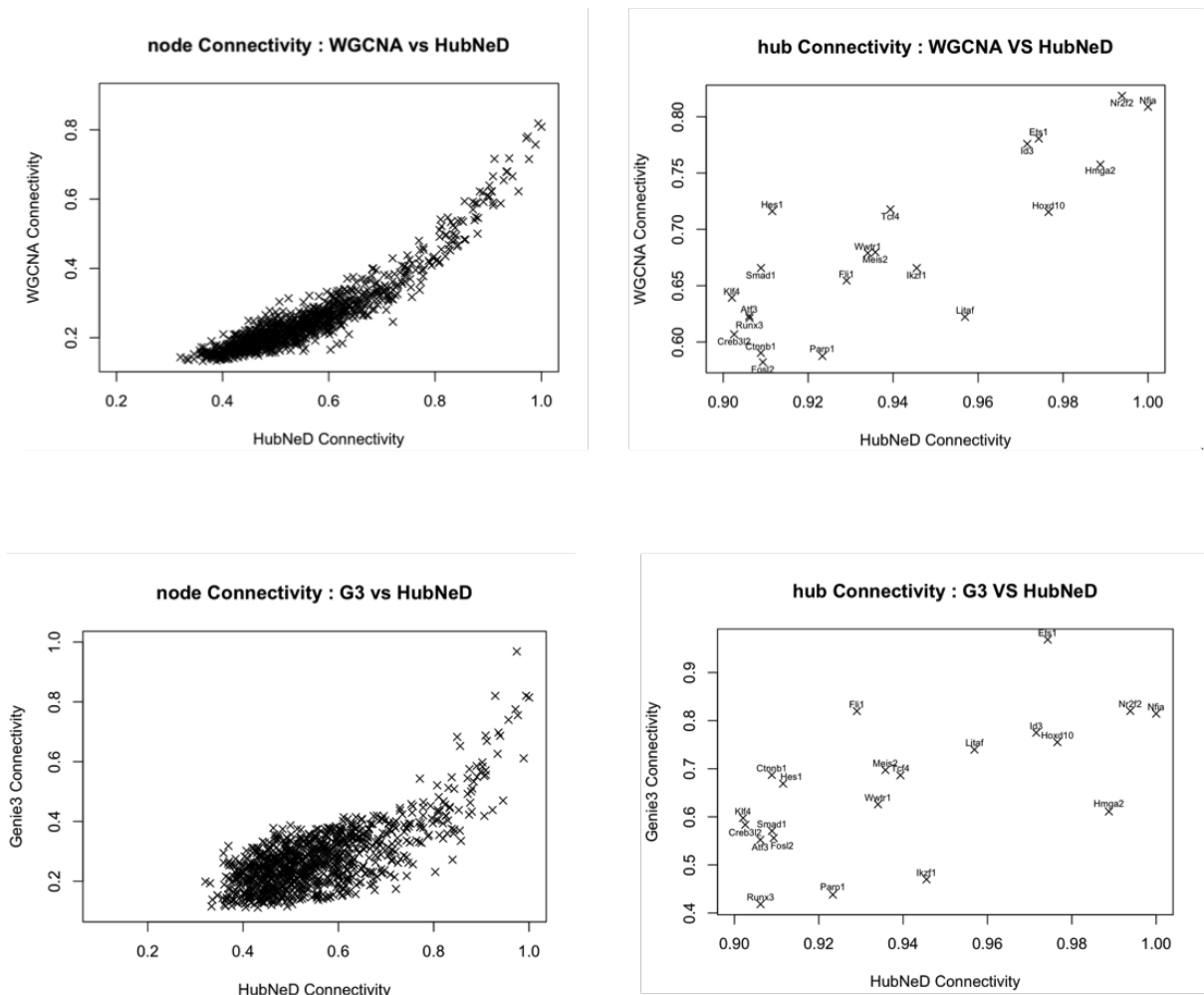
FIGURE 6.2 – Comparaison des connectivités des noeuds des réseaux reconstruits par HubNeD d'une part et WGCNA ou Genie3 d'autre part.
