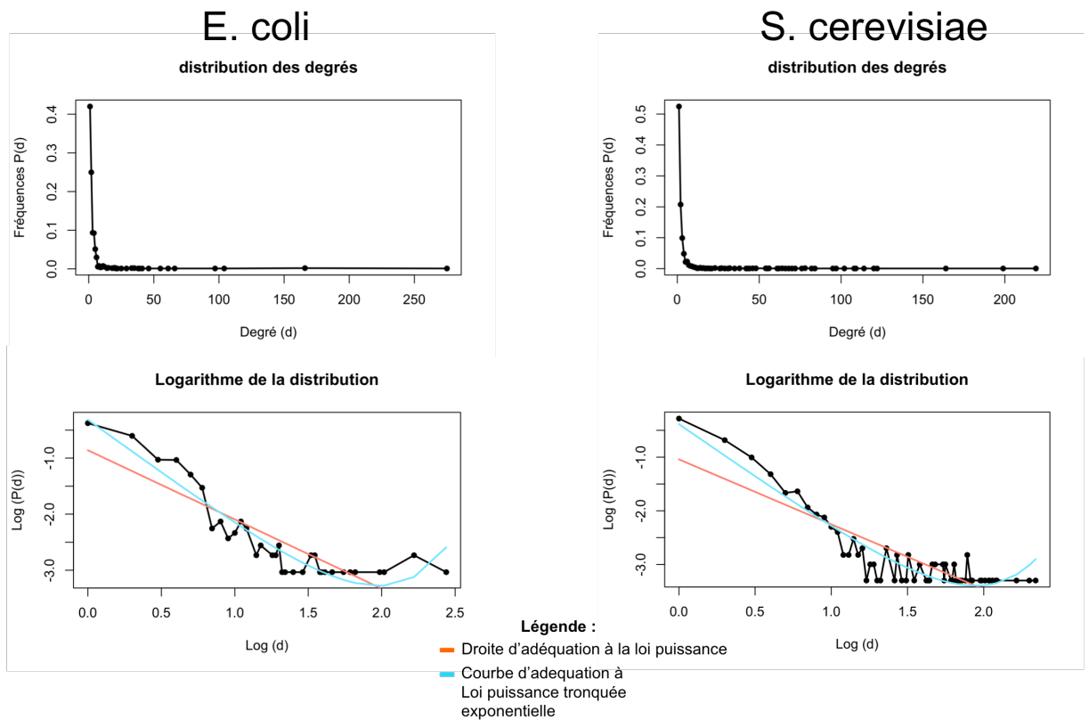
FIGURE 3.2 – Les distribution des degrés des RRGs de référence d’ E.coli et de S. cerevisiae . Les droites en orange correspondent aux droites de regression linéaire entre \log(P(d)) et \log(d) . Elles correspondent aux lois de puissances caractéristiques des topologies sans échelle. Les distributions des degrés sont plus proches des courbes en vert qui correspondent à des distributions en loi de puissance tronquée par une exponentielle.
