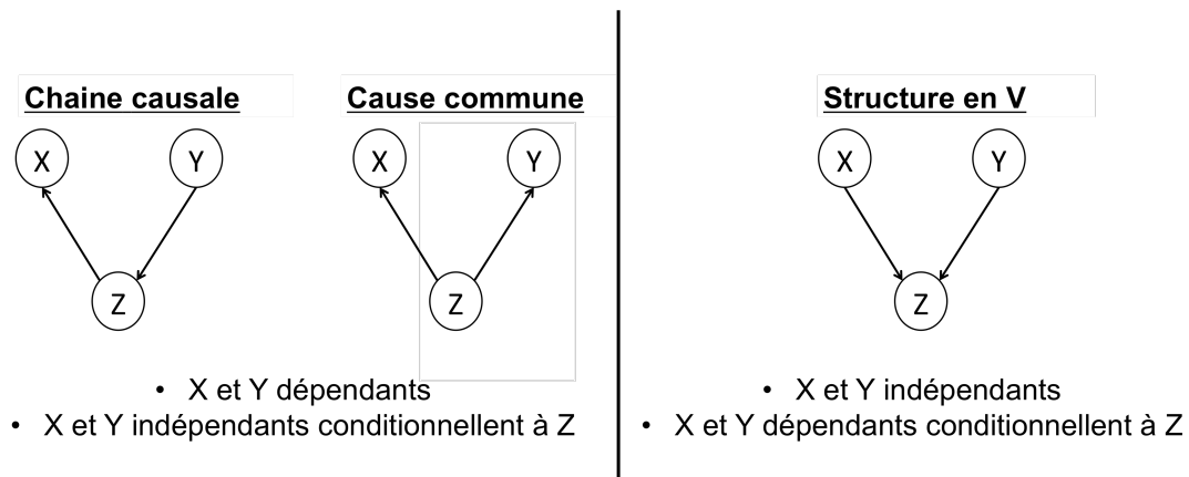
FIGURE 3.6 – Indépendance conditionnelles et réseaux Bayésiens
