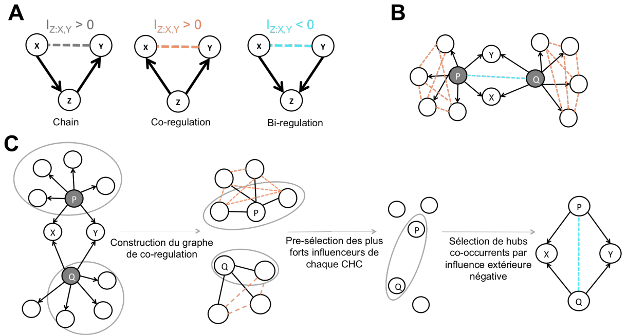
FIGURE 4.6 – Usage des scores d'influence pour la détection des hubs dans le contexte des données simulées. A. Les trois structures possibles avec trois noeuds x, y, z et deux arêtes (x, z) et (y, z) : chaîne (gauche), co-régulation (centre) et bi-régulation (droite). Pour chaque triplet, une ligne discontinue indique l'arête I_{z;x,y} , l'influence de z sur la relation entre x et y . Pour les chaînes et co-régulations, I_{z;x,y} est significativement positif (lignes discontinues grise et orange). Pour la bi-régulation, I_{z;x,y} est significativement négatif (ligne en pointillé bleu). B. Un réseau simple à 2 hubs déconnectés affiche des structures de co-régulation formées entre chaque hub et leurs cibles respectives (lignes pointillées orange) et des structures de bi-régulation formées entre les 2 hubs et leurs cibles communes x et y (ligne pointillée bleue) C. Procédure de sélection des hubs. Un simple réseau avec deux hubs (noeuds gris) est considéré (à gauche).
