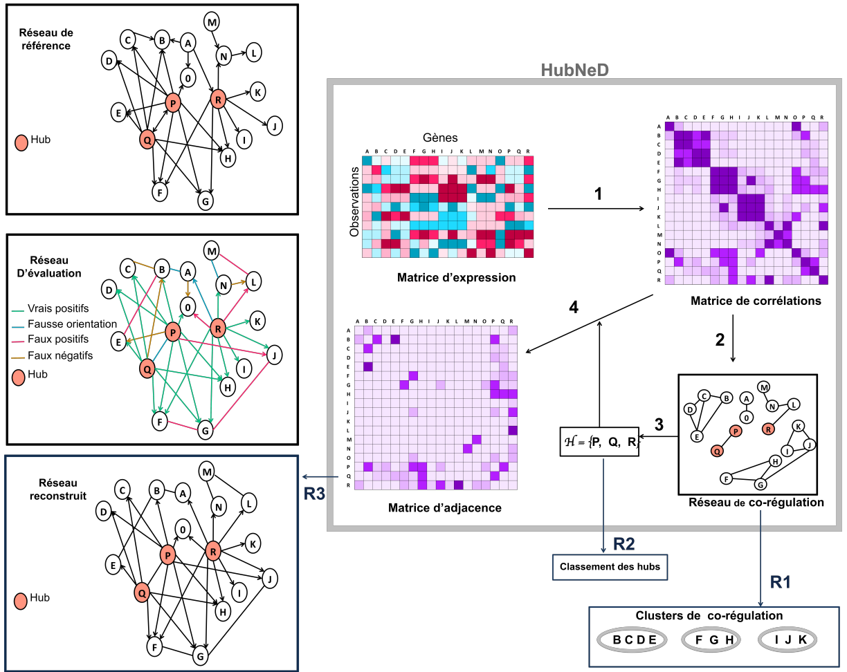
FIGURE 4.2 – Étapes du déroulement de la reconstruction d'un RRG par HUBNeD sur un exemple simple. Les 4 étapes sont représentés par les flèches numérotées de 1 à 4. 1 : Calcul des scores de corrélation de Pearson
