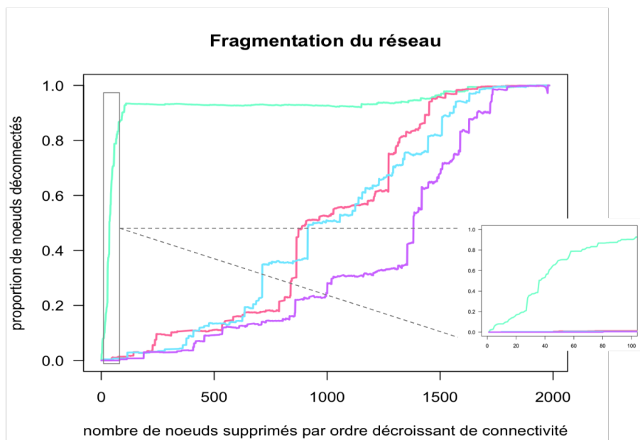
FIGURE 5.2 – Capacité des méthodes à fragmenter les RRGs d' E. coli et de S. cerevisiae
