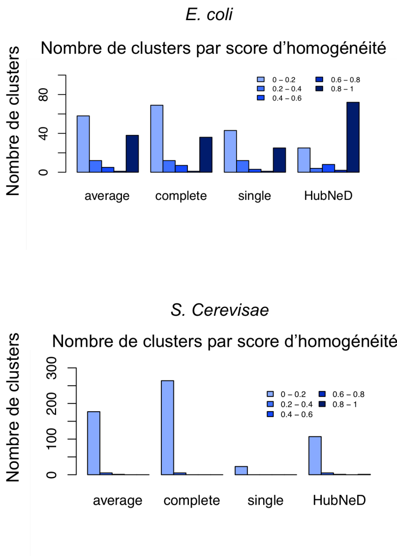
FIGURE 5.1 – Barplot montrant les performances du clustering par co-régulation homogène d’HubNeD comparé à trois différentes méthodes de clustering partiel. Les performances sont évaluées par l’homogénéité des clusters extraits. Pour un cluster spécifique, un score d’homogénéité de 0 signifie que les gènes dans le cluster ne partagent pas de régulateur commun et un score d’homogénéité de 1 signifie que tous les gènes ont exactement les mêmes régulateurs. HubNed est clairement la meilleure méthode pour capturer des grappes de co-régulation parfaitement homogènes pour E.coli . Toutes les méthodes fonctionnent mal pour S. cerevisiae .
