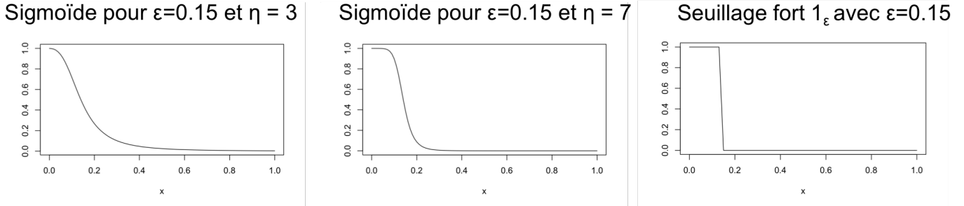
FIGURE 4.4 – courbes de fonctions de seuillage souple (les deux courbes à gauche) et une courbe pour le seuillage fort (à droite)
