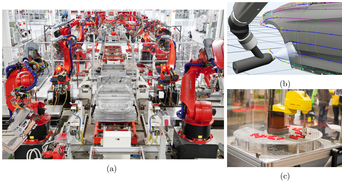
Figure 2 – (a) Ligne d’assemblage de la giga-usine Tesla : à chaque poste, plusieurs manipulateurs équipés de soudeuses à l’arc appliquent les points de soudure préprogrammés. (b) Trajet planifié pour une opération automatisée de pulvérisation sur la carrosserie d’une voiture. (c) Un robot SCARA effectuant des opérations de pick-and-place dans un environnement bien structuré.
