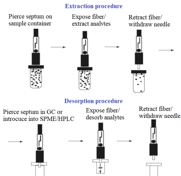
Figure 3.4 : Diagramme schématique des procédures d'adsorption et de désorption en SPME (Source: Reproduit avec la permission de Supelco Bulletin, (1998), 923, 1–5. © Sigma-Aldrich Co.).
