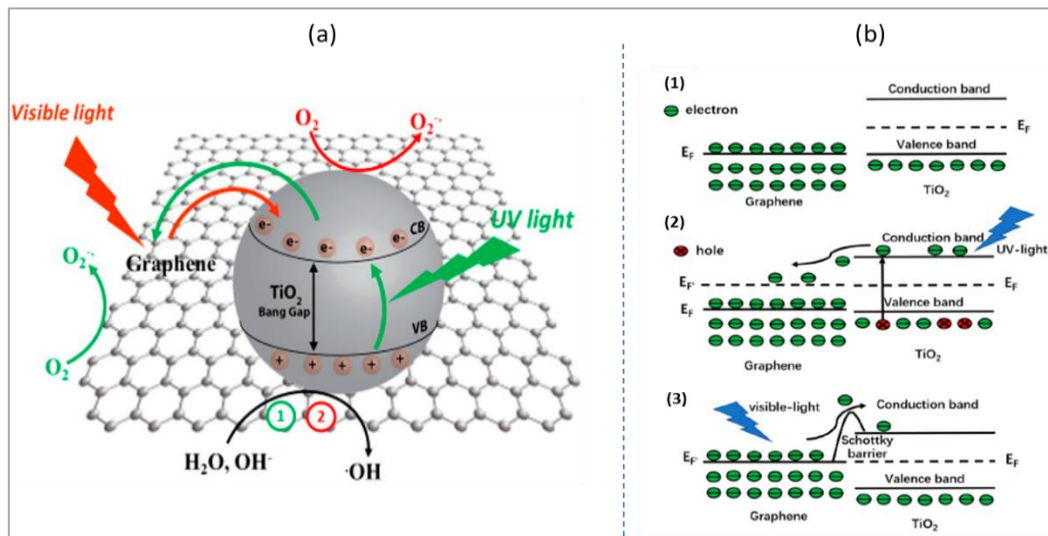
Figure I.25: Les processus de transfert de charges photogénérées sous UV ou Visible dans les composites \text{TiO}_2/\text{graphène} [292] [306]
