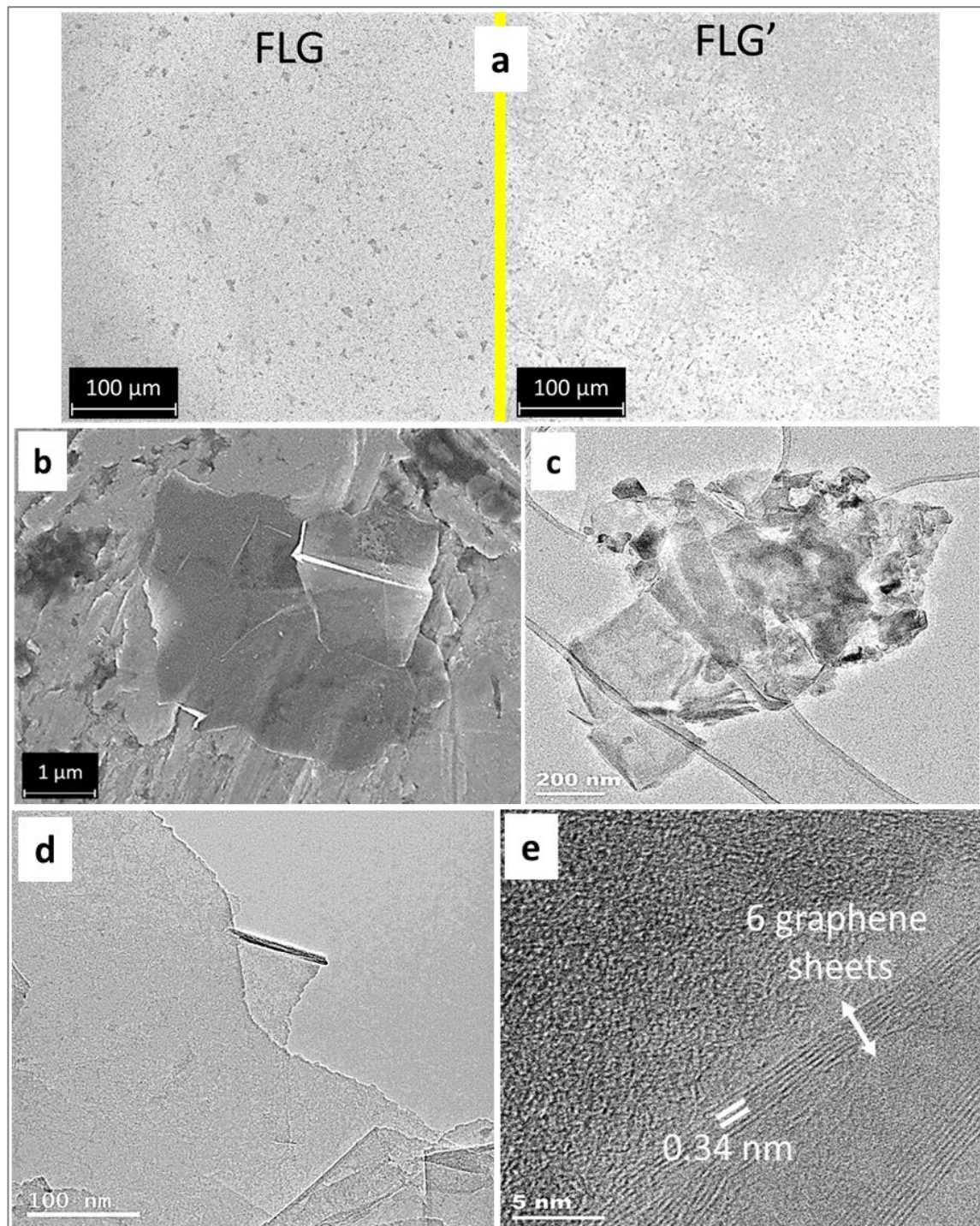
Figure II.23: (a) Images MEB de FLG et FLG' (effet de sonication), (b) Images MEB et (c-e) MET de FLG
