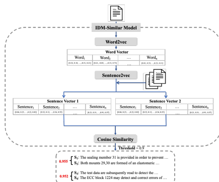
Fig. 3. Le cadre d'IDM-Similar
