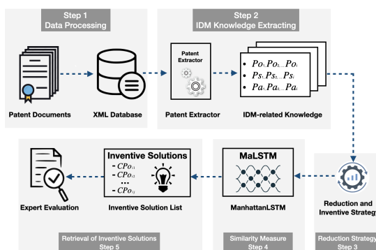
Fig. 4. Le cadre de SAM-IDM
