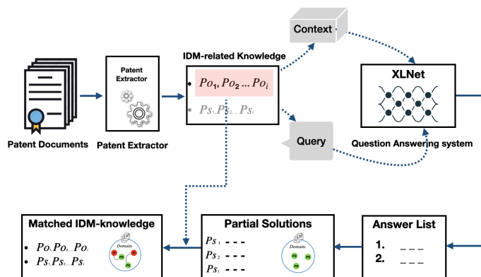
Fig. 5. Le cadre de l’IDM-Matching
