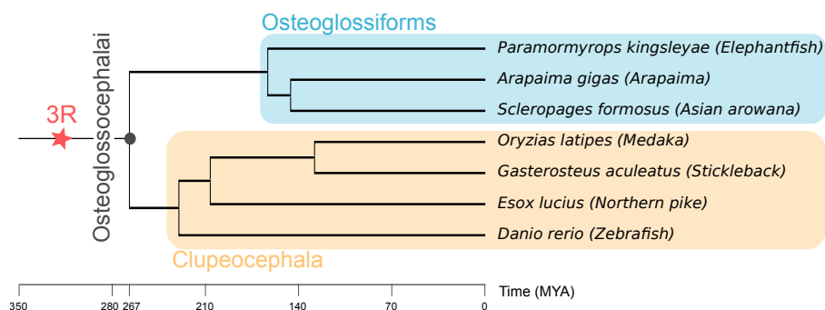
FIGURE 4.10 – Phylogénie des espèces Osteoglossocephalai utilisées. Les dates de divergences (en millions d'années) sont extraites de TimeTree (KUMAR et al. 2017). La position de la duplication 3R, datée à 320 millions d'années (VANDEPOELE et al. 2004), est indiquée par une étoile.
