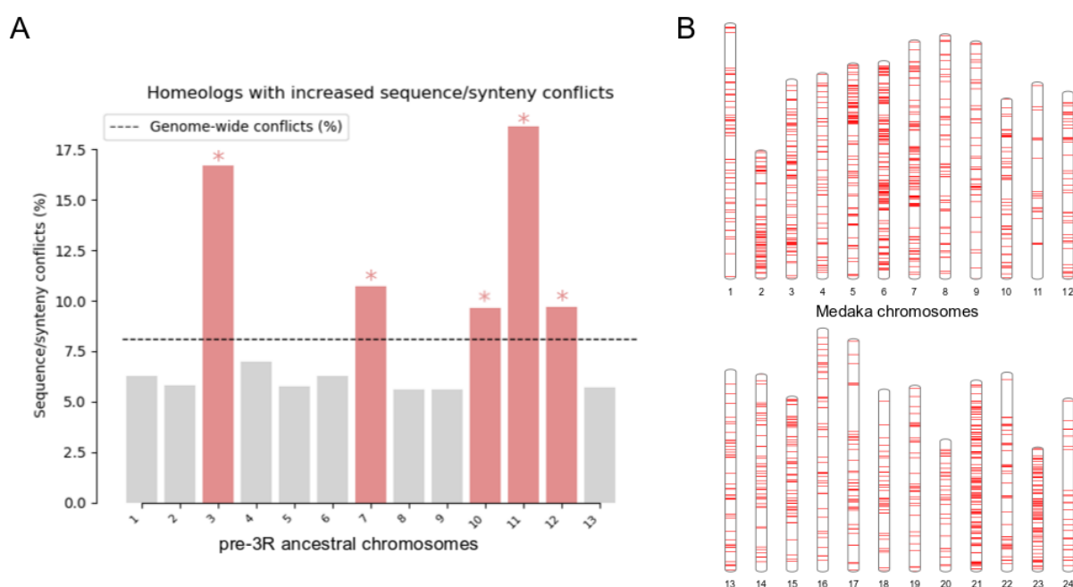
FIGURE 4.11 – Distribution des conflits séquences/synténie dans les génomes d’Osteoglossoccephalai. A. Chromosomes homéologues enrichis en conflits de prédictions entre séquence et synténie. Représentation comme en Figure 4.8, à l’exception de l’axe des abscisses qui correspond aux 13 chromosomes pré-3R (voir le chapitre précédent). Les paires d’homéologues qui descendent des chromosomes pré-duplication 3, 7, 10, 11 et 12 sont enrichis en conflits séquence/synténie (* p-valeur < 0.05, tests hypergéométriques corrigés pour les tests multiples). B. Distribution des gènes appartenant aux 1 121 arbres incongruents sur le génome du medaka, comme en Figure 4.8.
