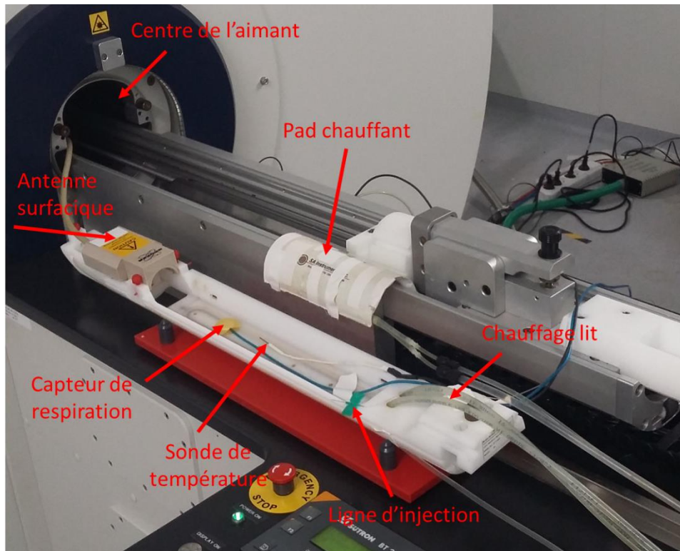
Figure VI-1 : Configuration expérimentale
