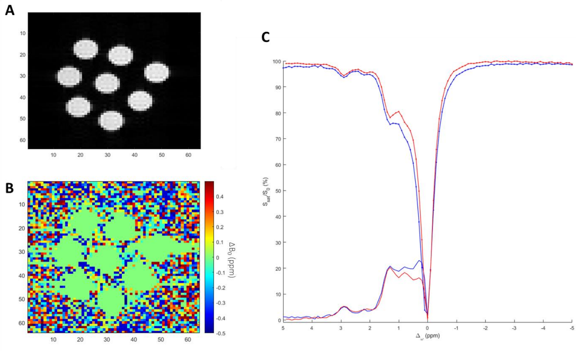
Figure V-7 : Processus de correction WASSR appliqué sur fantôme
