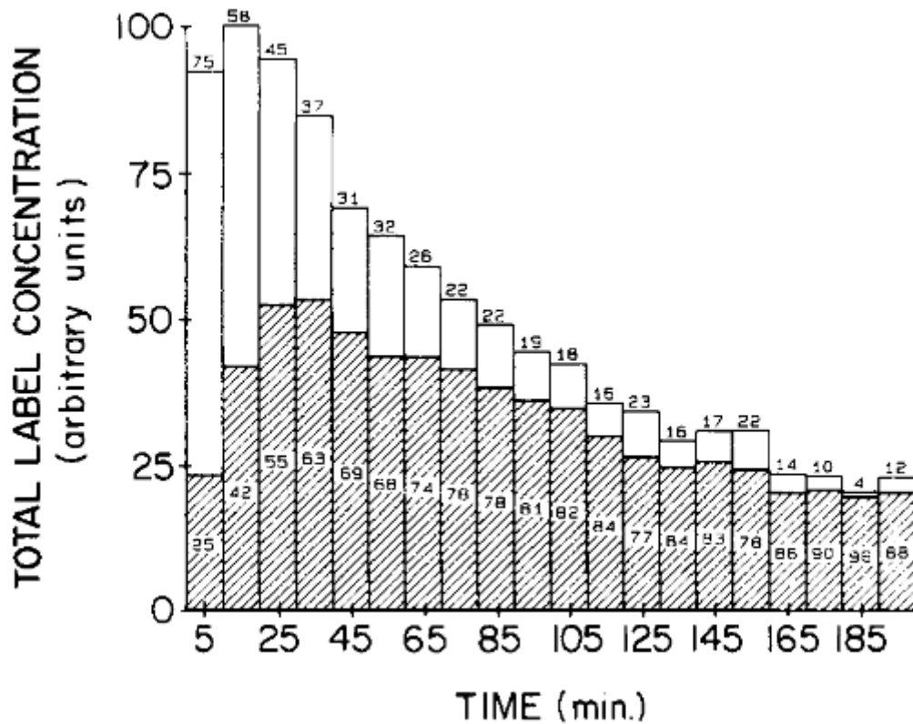
Figure VII-13: Moyenne des aires des pics ^{13}\text{C}(^1\text{H}) RMN du ^{13}\text{C}2\text{DG} et ^{13}\text{C}2\text{DG}6\text{P} dans le tissu cérébral après injection de ^{13}\text{C}2\text{DG} à 0,5 g/kg (n=4), (Kotyk et al. 1989)
